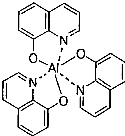
Alq3:
