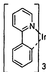
Ir(ppy) 3
