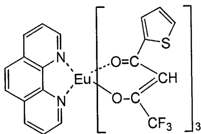
Eu(TTFA) 3 Phen (D3)
