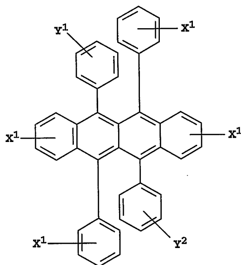
Formula Va
