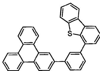
H2
