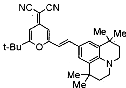
DCJTb
