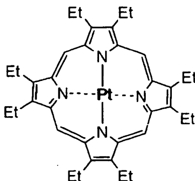
PtOEP
