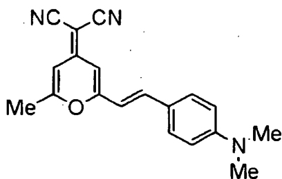
DCM
