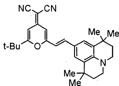
DCJTB
