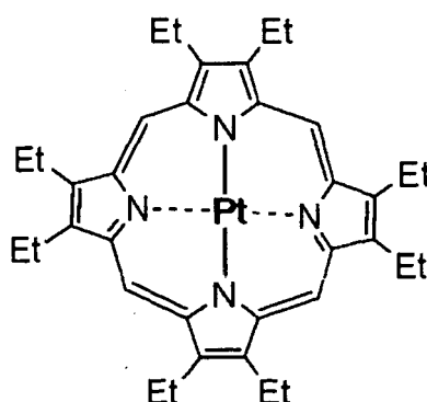
PtOEP
