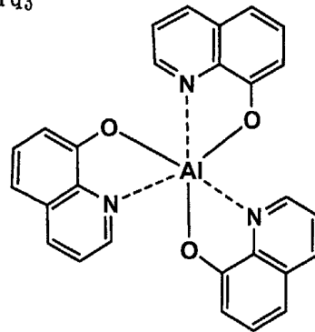
Alq 3
