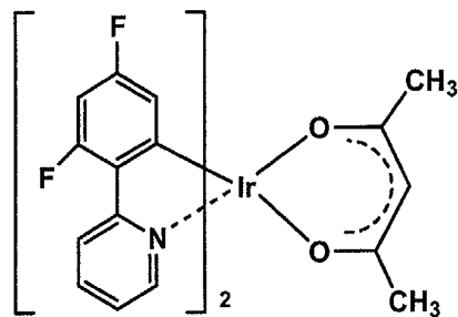
Ir-10
