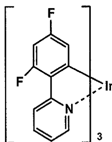
Ir-11
