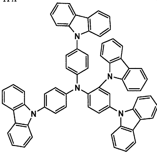
TPA
