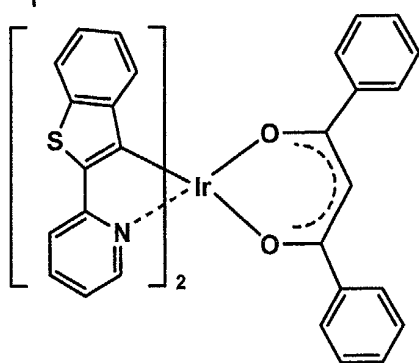
Ir-7
