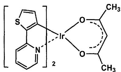
Ir-5
