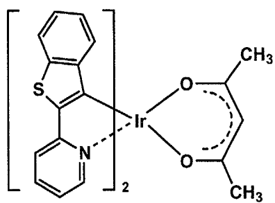
Ir-9
