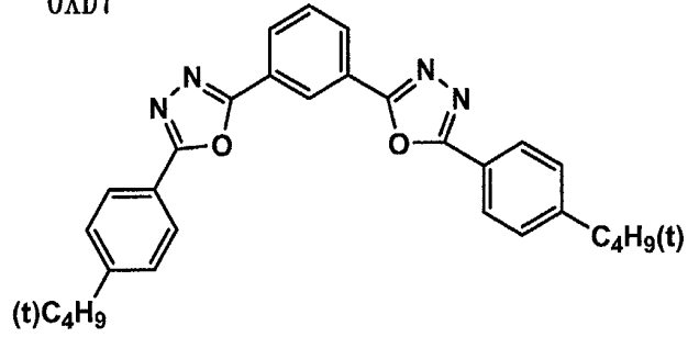
OXD7
