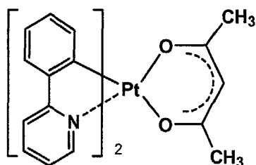
Pt-1
