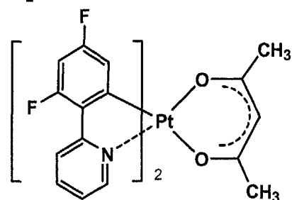
Pt-2
