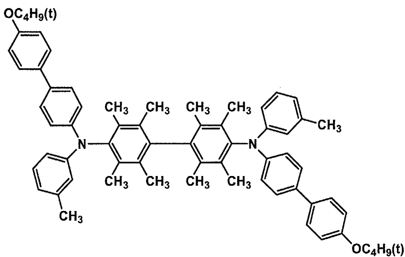
NP-14
