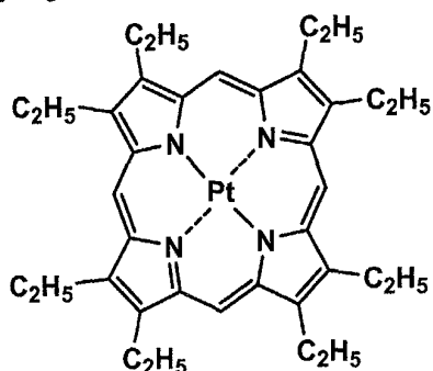
Pt-3
