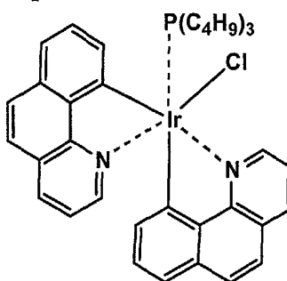
Ir-4
