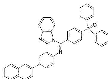
[Formula 1-18]
