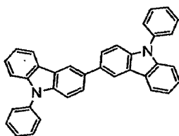
Compound F1
