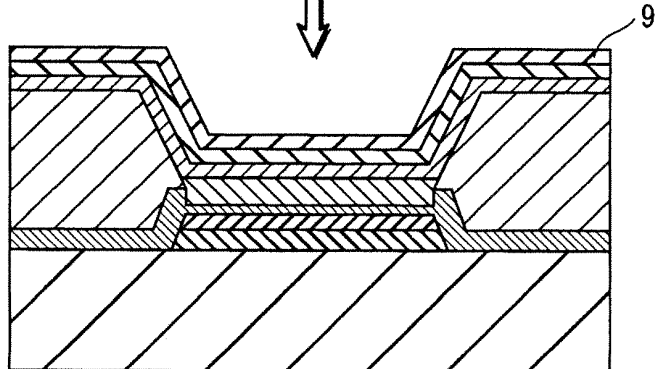
FIG. 8H
