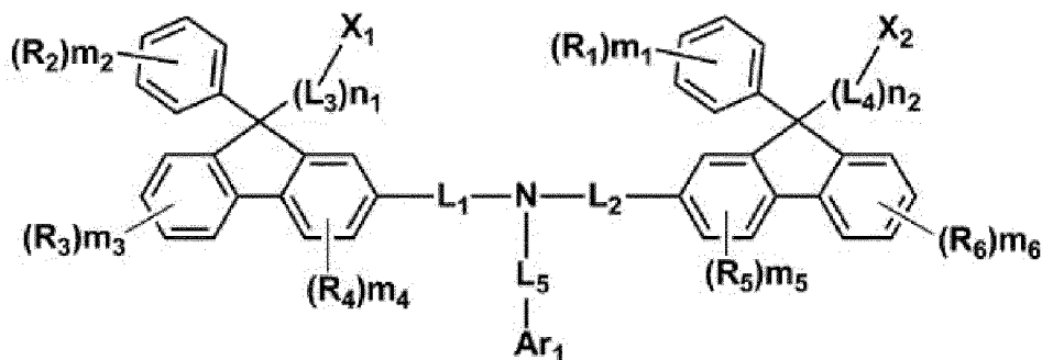
[Formule chimique 1]
