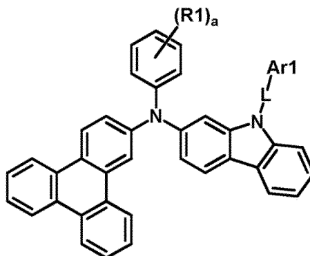
[Formule chimique 4]
