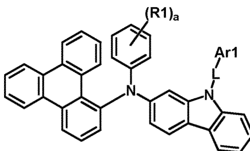
[Formule chimique 5]
