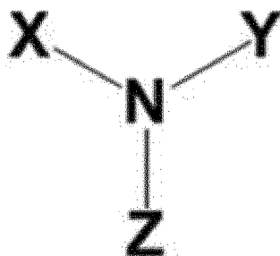
[Formule chimique 1]
