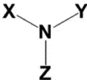
chemische Formel 1
