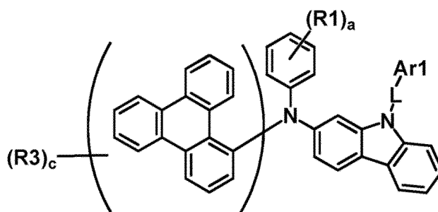
[Formule chimique 3]
