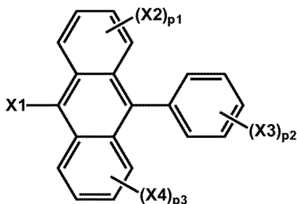
[Formule chimique 7]
