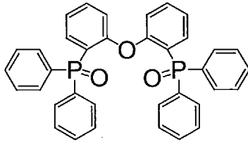
DPEPO
