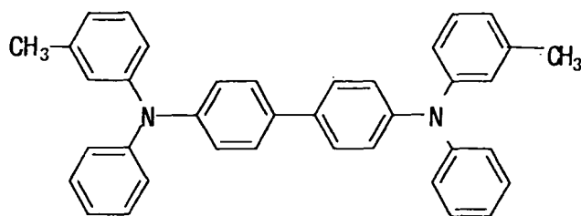
TPD
