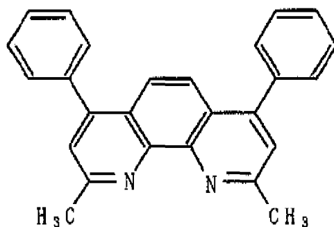
BCP
