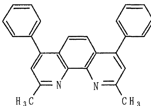
BCP
