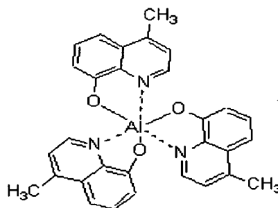
Almq3
