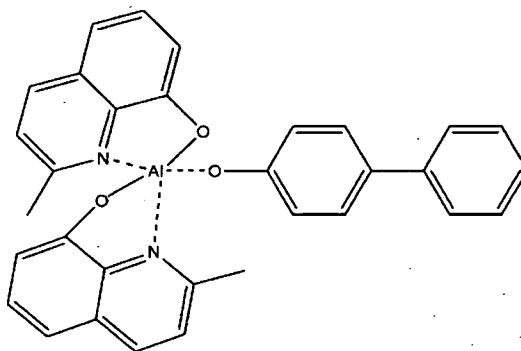
Balq
