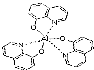
Alq3
