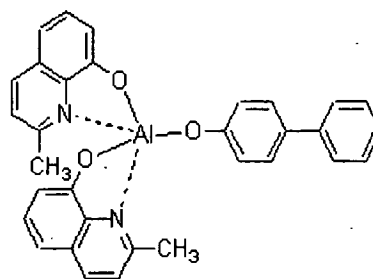
BAlq
