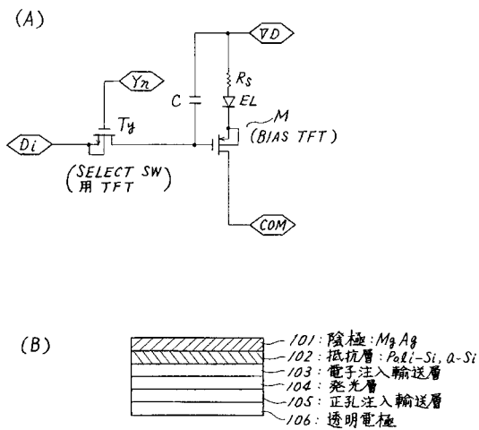
薄膜画素素子の寄生抵抗を用いる場合の説明図
