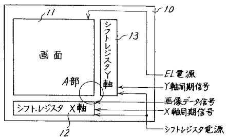
(A) パネルブロック図
