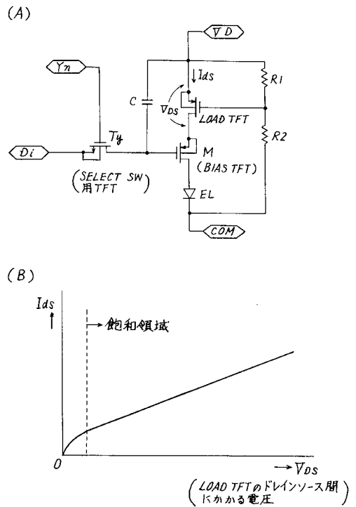
非線形素子の出力抵抗を用いる場合の説明図
