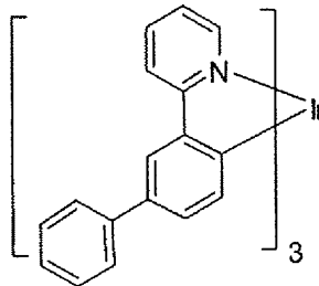
化合物 B
