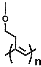
式(12)
