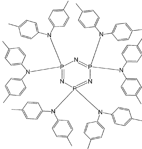
化合物 5
