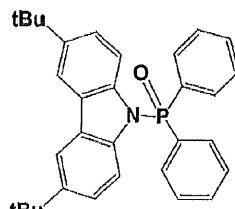
tBuCzPO
