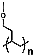
式(11)
