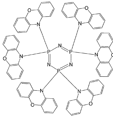
化合物 2
