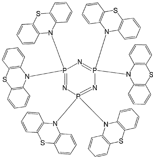
化合物 3
