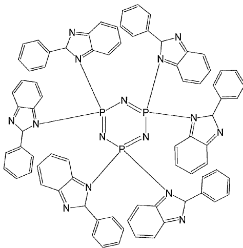
化合物 7
