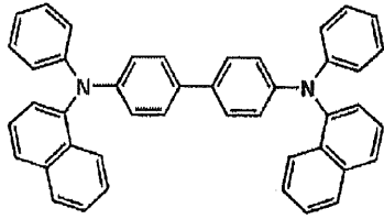
\alpha -NPD
