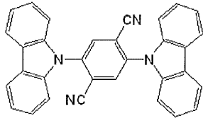
2CzCN
