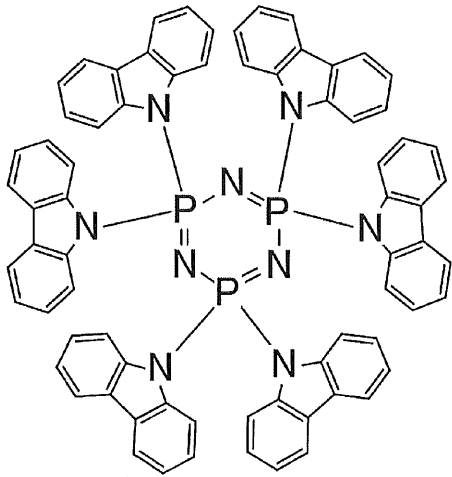
化合物 1
