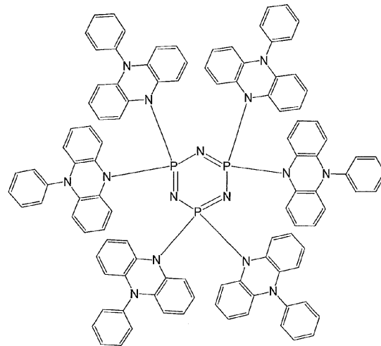
化合物 6
