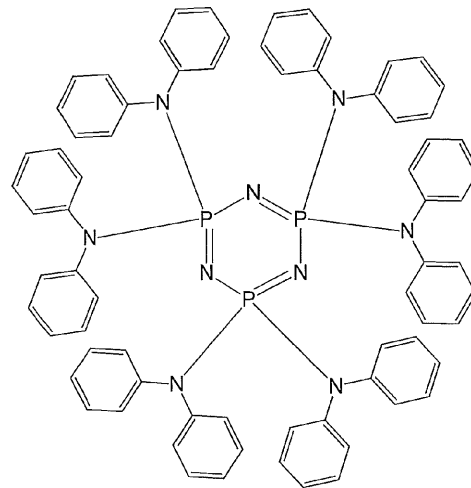
化合物 4
