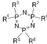
一般式(1)
