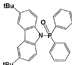
tBuCzPO
