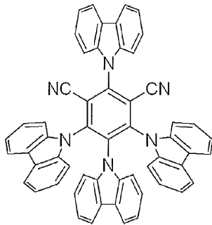
4CzIPN
