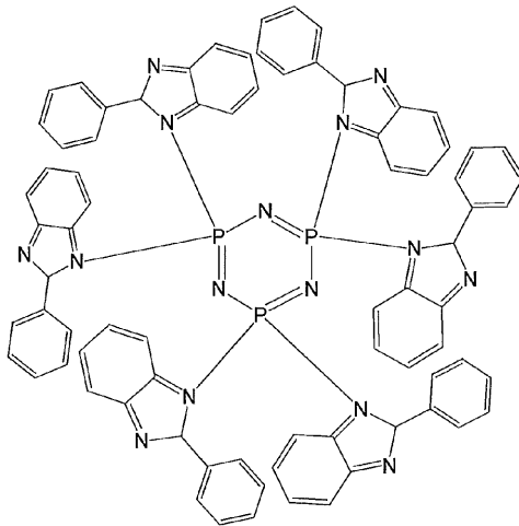
化合物 7
