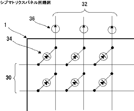
パッシブマトリクスパネル回路図
