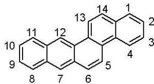
ベンゾ [ b ] クリセン
