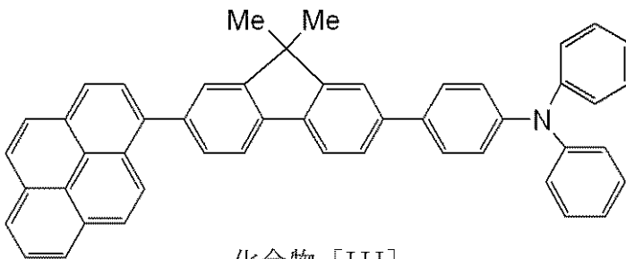
化合物 [III]
