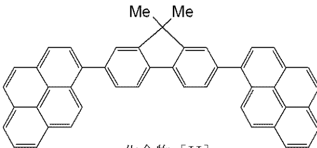
化合物 [II]
