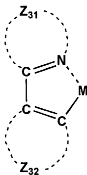
一般式(3)
