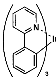
比較化合物2
