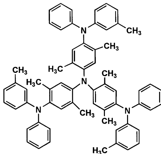
化合物1
