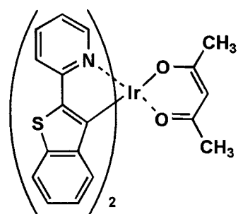
比較化合物3
