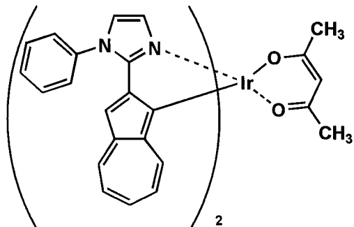
5-4
