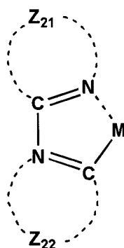
一般式(2)
