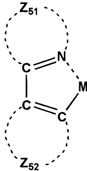
一般式(5)
