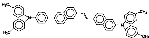
一般式 (4-5).
