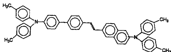
一般式 (4-2);
