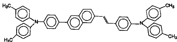
一般式 (4-4); 又は
