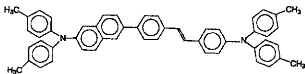
一般式 (4-3);
