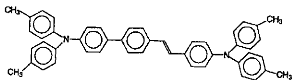
一般式 (4-1);
