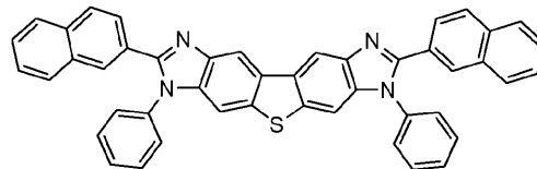
比較化合物4
