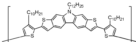
比較化合物3
