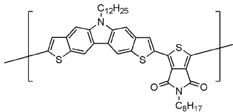
比較化合物3
