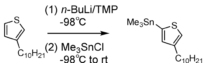
中間体2
