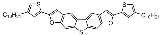
化合物 8
