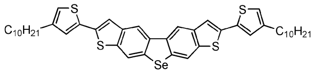
化合物 6
