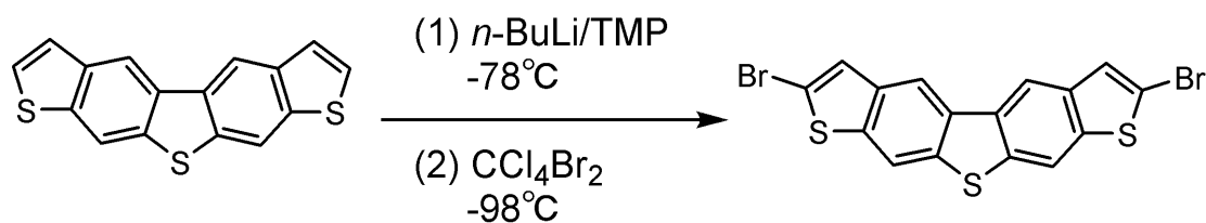
中間体1
