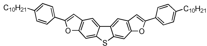
化合物 9
