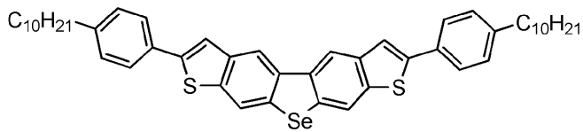
化合物 7
