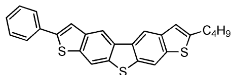
化合物 1 2
