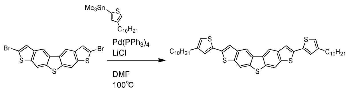
中間体1
