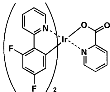
比較化合物1
