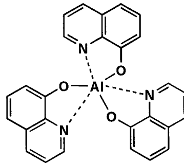
Alq 3
