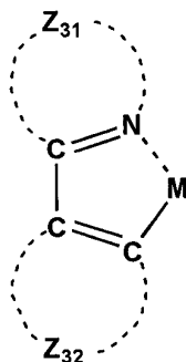
一般式(3)
