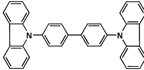
CBP
