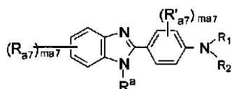
一般式 (A-VII)
