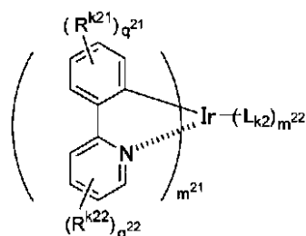
一般式(K-II)
