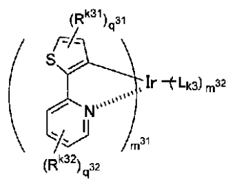
一般式(K-III)
