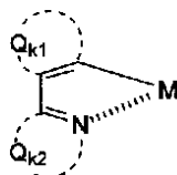
一般式(K-I)
