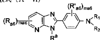
一般式 (A-VII)
