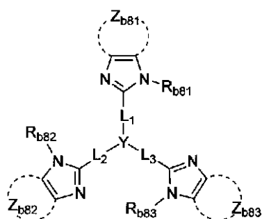
一般式(B-VII)
