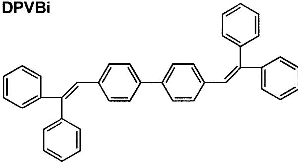
比較化合物1
