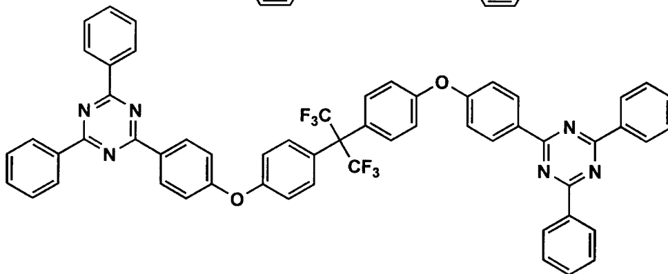
比較化合物2
