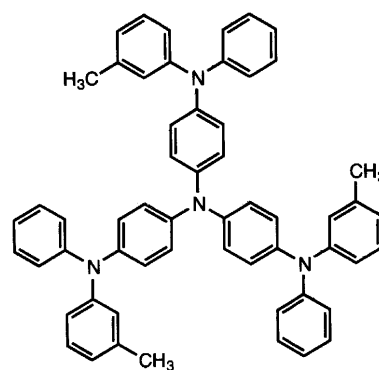
m - MTDATA
