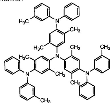
m - MTDATXA
