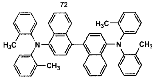
化合物H-2
