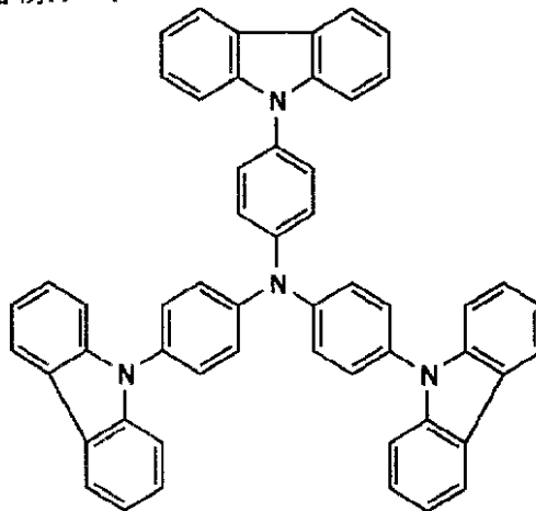
化合物H-4
