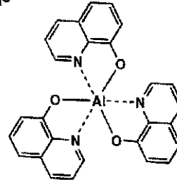
化合物E-1
