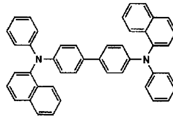
化合物H-1
