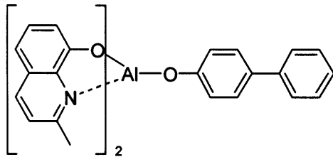
BAlq
