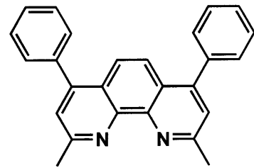
ET-5(BCP)
