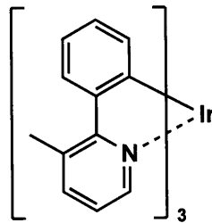
D-2(Ir(piq) 3 )
