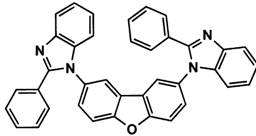
比較化合物4
