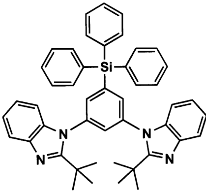
比較化合物1
