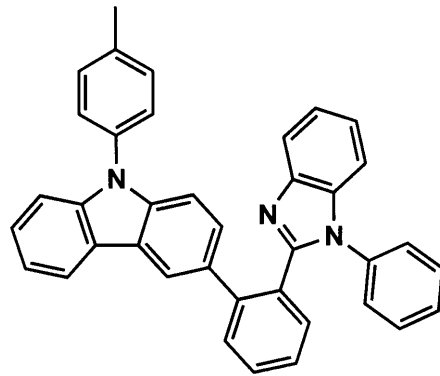
比較化合物2
