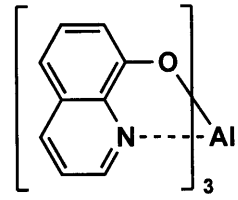
ET-2(Alq 3 )
