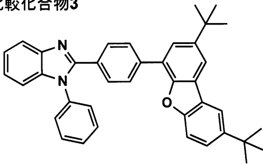
比較化合物3
