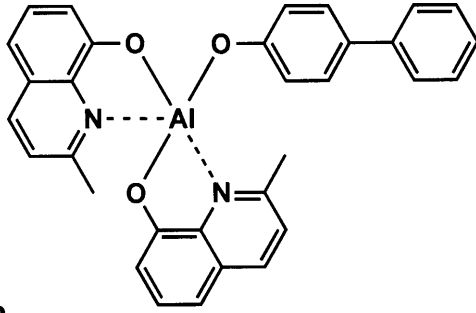
ET-1(BAlq)
