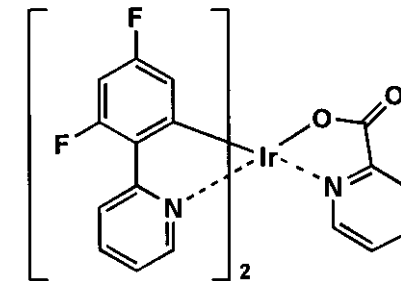
Ir-14
