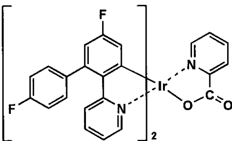
Ir-13
