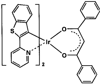
Ir-9
