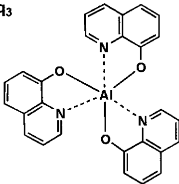
CB 4 -TPA
