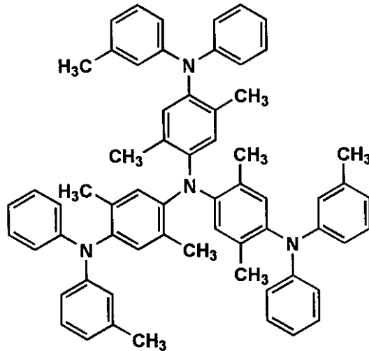
m-MTDATXA
