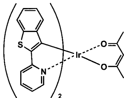
Btp2Ir(acac)
