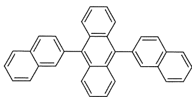
構造式(104) ADN
