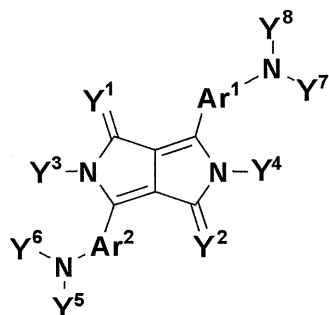
一般式(1)
