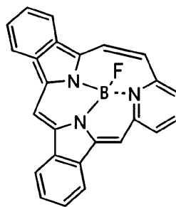
化合物(53)
