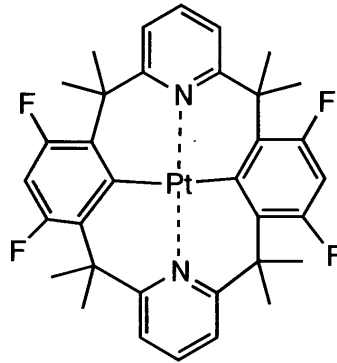
化合物(128)
