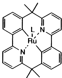
化合物(124)
