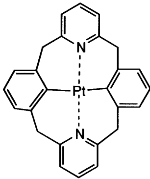
化合物(129)
