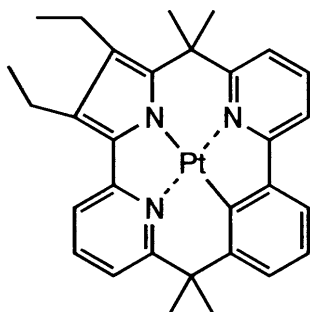
化合物(153)
