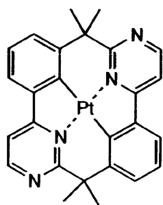
化合物(104)
