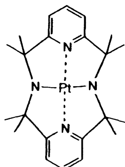
化合物 (159)
