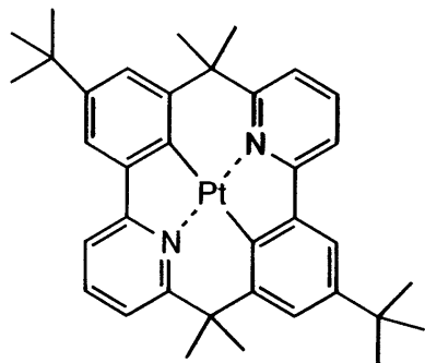
化合物(80)
