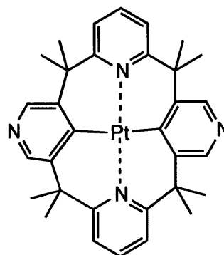
化合物(140)
