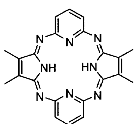
化合物(14)
