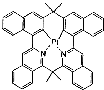
化合物(86)
