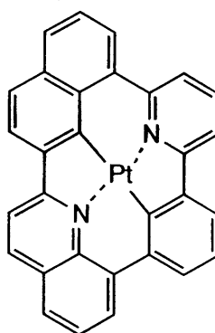
化合物(91)
