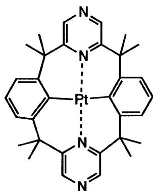
化合物(137)
