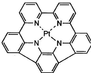
化合物(95)
