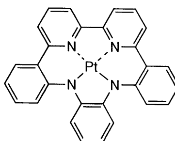
化合物(93)
