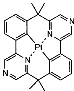
化合物(101)
