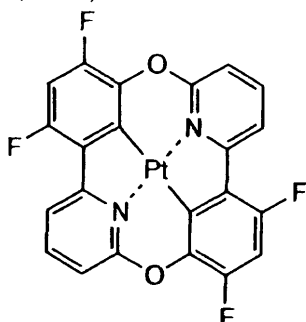
化合物 (157)
