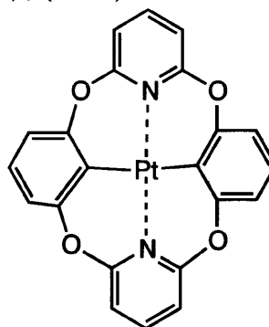
化合物(136)
