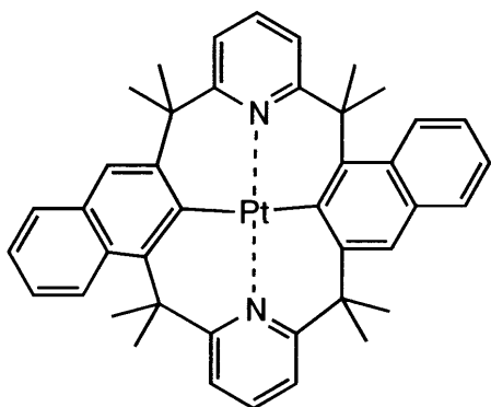
化合物(149)
