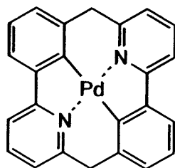
化合物(122)
