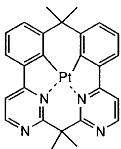
化合物(105)
