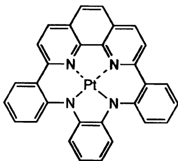
化合物(94)
