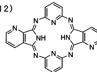
化合物(13)
