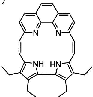
化合物(52)
