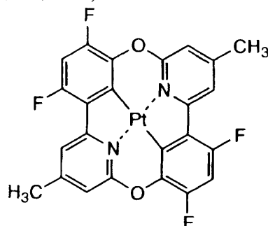
化合物 (158)
