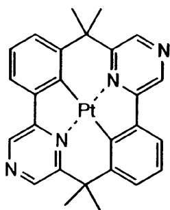
化合物(102)
