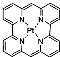
化合物(57)
