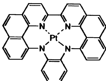
化合物(100)
