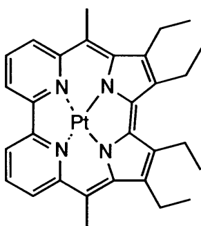
化合物(153)
