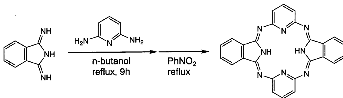
化合物(1)
