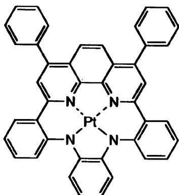
化合物(98)
