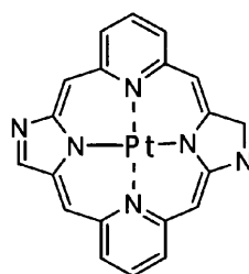
化合物(31)
