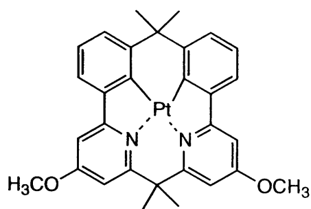
化合物(115)
