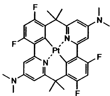
化合物(74)
