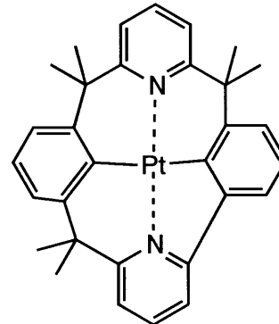
化合物(154)
