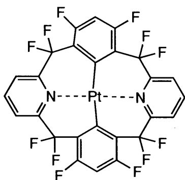
化合物(147)
