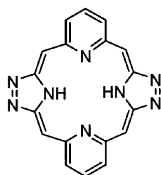
化合物(26)
