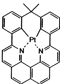
化合物(88)
