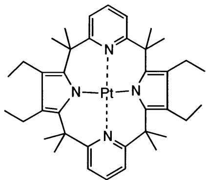
化合物(141)
