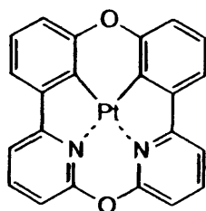
化合物 (157)
