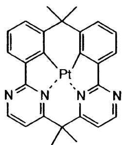
化合物(108)
