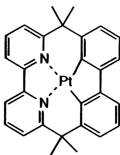
化合物(90)
