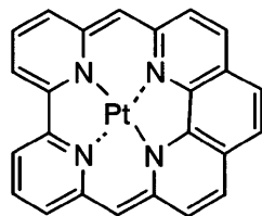
化合物(59)
