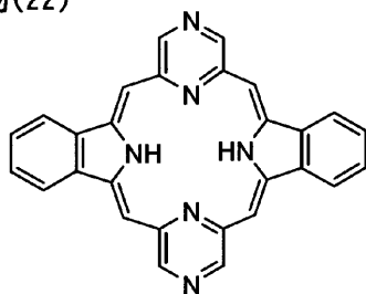
化合物(23)
