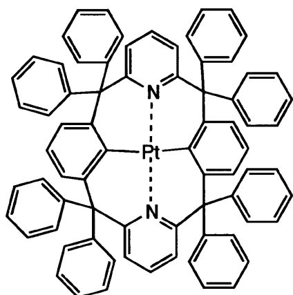
化合物(139)
