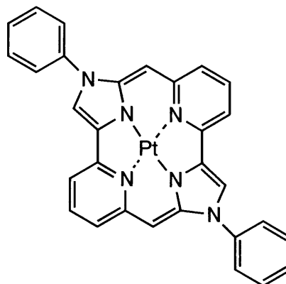
化合物(152)
