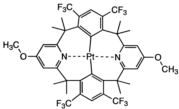
化合物(148)
