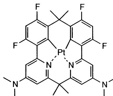
化合物(81)
