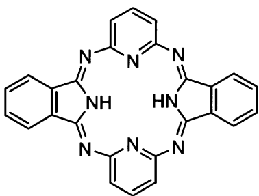
化合物(1)
