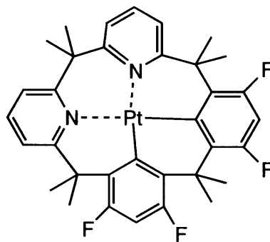
化合物(130)
