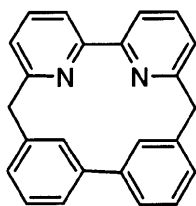
化合物(45)
