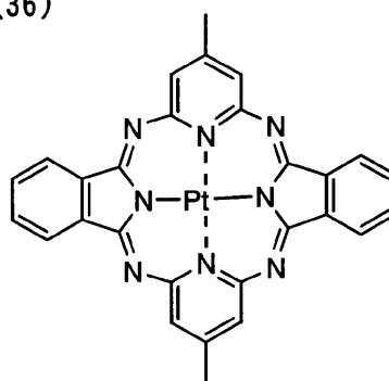
化合物(36)
