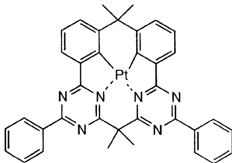
化合物(109)
