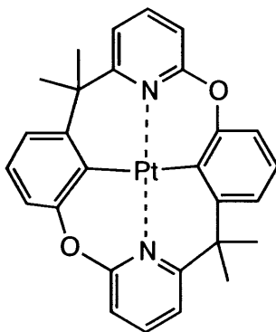
化合物(131)
