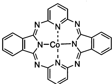
化合物(2)
