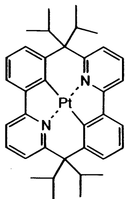
化合物(68)
