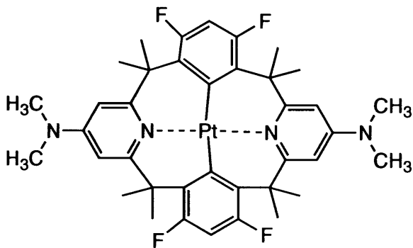
化合物(129)
