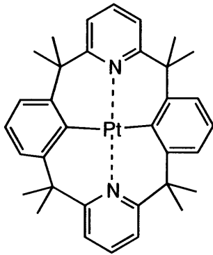
化合物(127)
