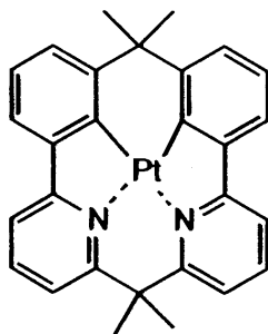
化合物(82)
