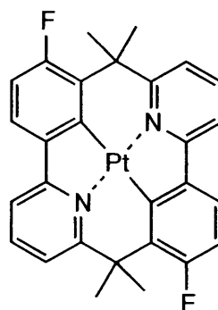
化合物(67)
