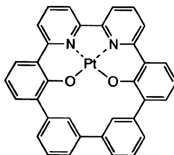
化合物(97)
