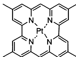
化合物(60)
