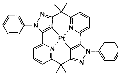
化合物 (158)
