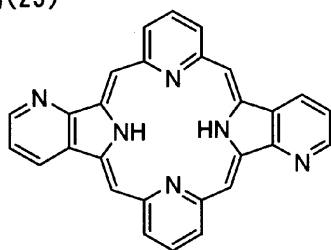
化合物(23)
