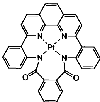
化合物(100)
