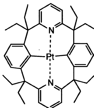
化合物(136)
