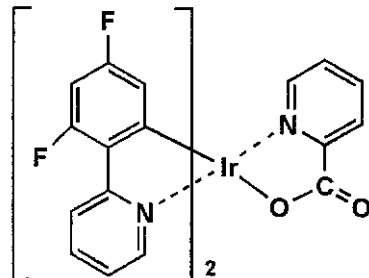
Ir-12
