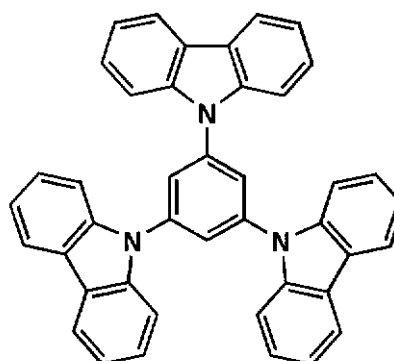
比較化合物2
