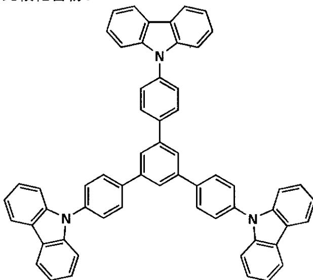
比較化合物1
