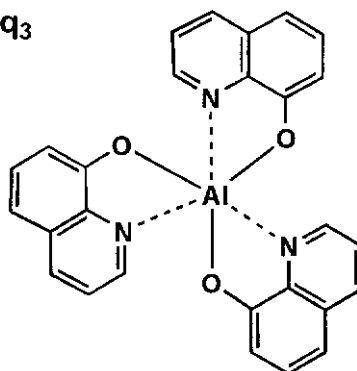
比較化合物2
