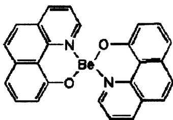
BeBq
