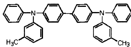
TPD
