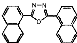
BND
