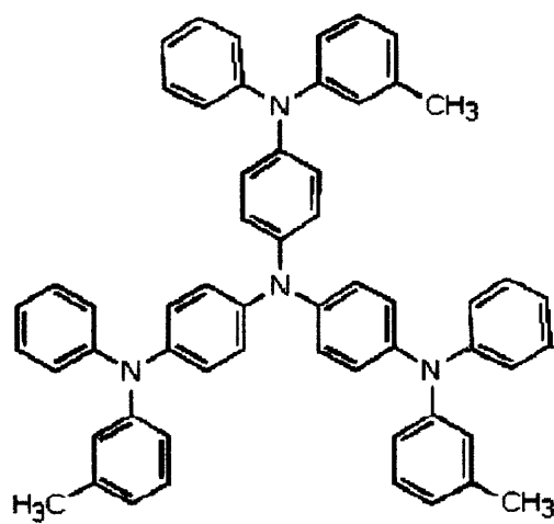
m-MTDATA
