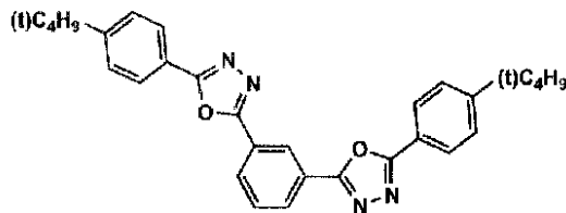
化合物E-2
