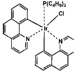
Ir-4
