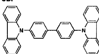
CBP
