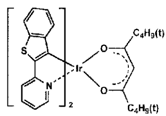
Ir-6
