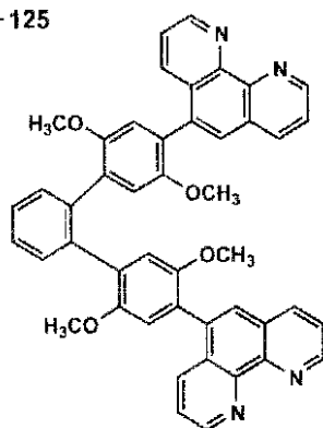
62 (I)-126
