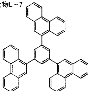
化合物 L-7
