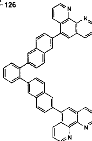
(I)-128
