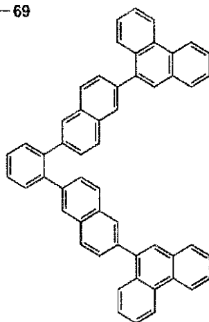
(I)-70
