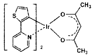
Ir-5
