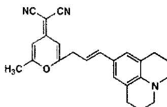
Qd-2
