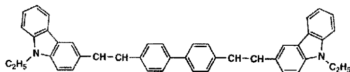
DCM-2
