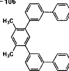
9a (II)-106
