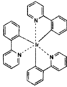
Ir-1
