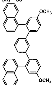
(II)-59
