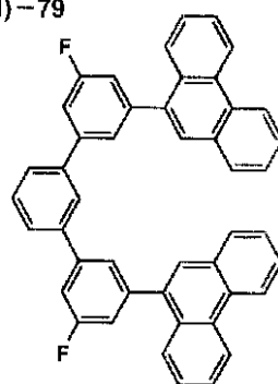
(II)-81
