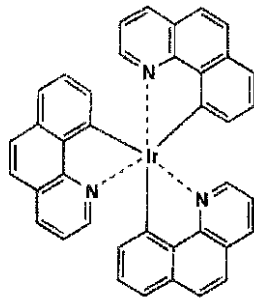
Ir-3
