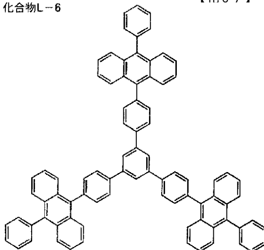
化合物 L-6
