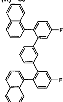
(II)-59
