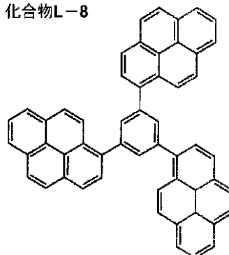
化合物 L-8
