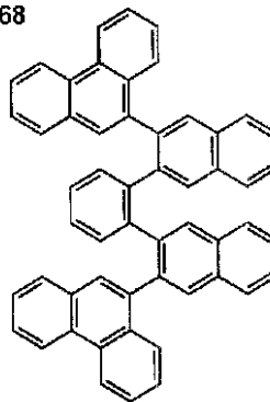
42 (I)-68
