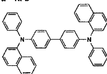
\alpha -NPD
