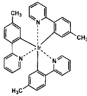
Ir-2
