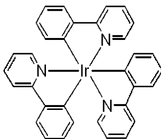
Ir(ppy) 3
