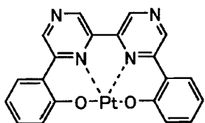
化合物 (191)
