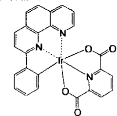
化合物 (122)
