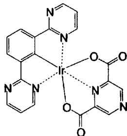
化合物 (129)
