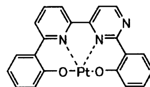
化合物 (195)
