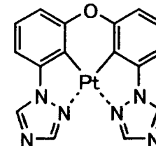
化合物 (232)
