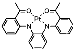
化合物 (87)
