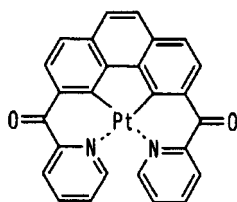
化合物(36)
