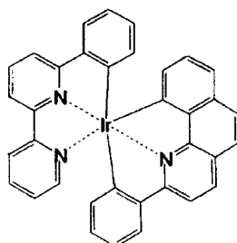
化合物 ( 1 0 2 )
