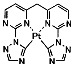
化合物 (225)
