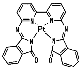
化合物(27)
