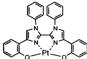
化合物 (75)
