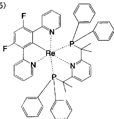
化合物(169)
