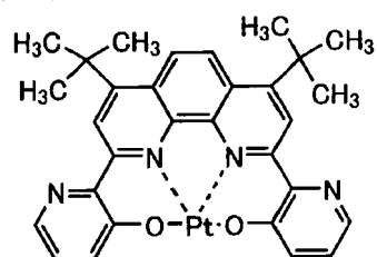
化合物 (208)
