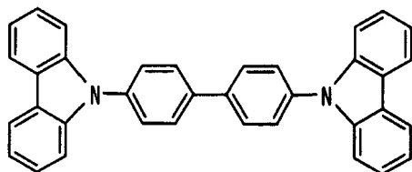
化合物A
