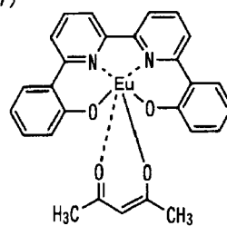
化合物(8)
