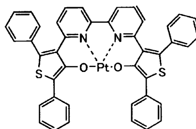
化合物 (210)
