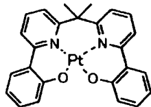
化合物 (66)
