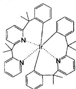
化合物 ( 1 0 2 )
