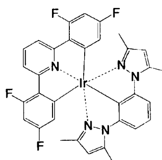
化合物 (176)
