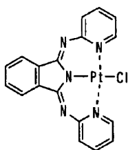
化合物(144)
