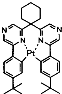
化合物 (81)
