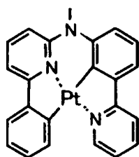
化合物 (138)
