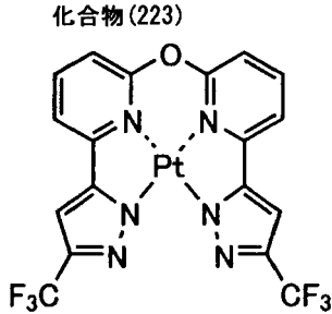
化合物 (223)
