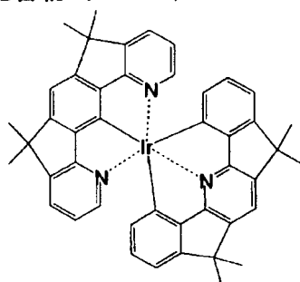
化合物 ( 1 0 0 )
