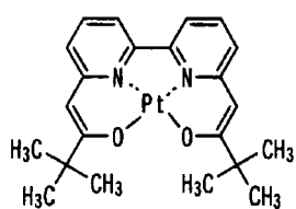
化合物(150)
