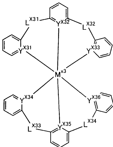
一般式(X3)
