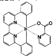
化合物 (120)
