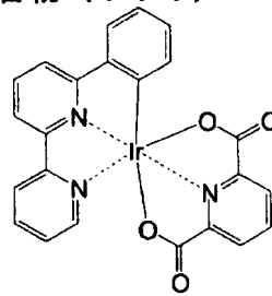
化合物 (115)
