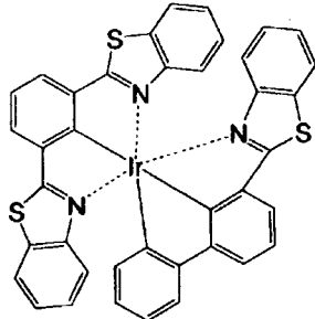
化合物 (130)
