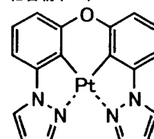
化合物 (229)
