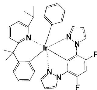
化合物(166)
