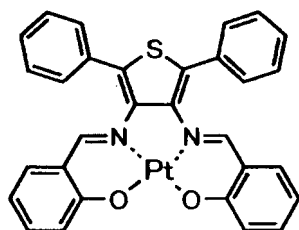
化合物 (91)
