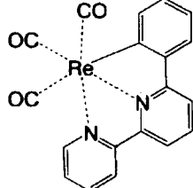
化合物 (131)
