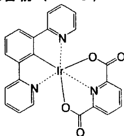
化合物 (114)
