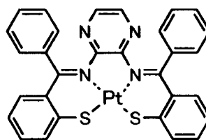
化合物 (95)
