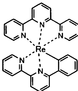
化合物 (142)
