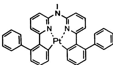
化合物 (86)
