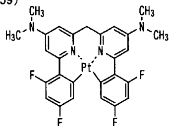
化合物(60)
