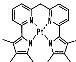
化合物(63)
