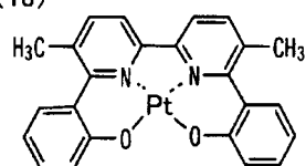
化合物(18)
