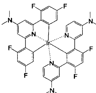
化合物 ( 1 0 5 )
