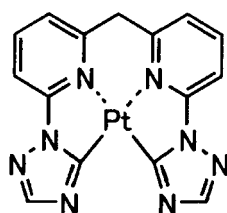
化合物 (216)
