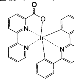
化合物 (117)
