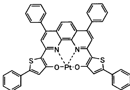
化合物 (206)
