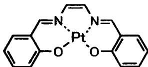
化合物 (90)
