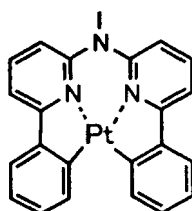
化合物 (85)
