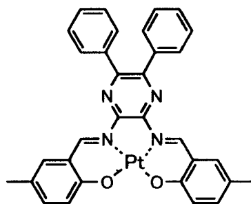
化合物 (94)
