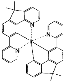
化合物 (125)
