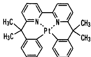
化合物(47)
