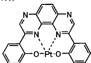
化合物 (191)
