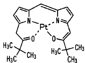
化合物(28)
