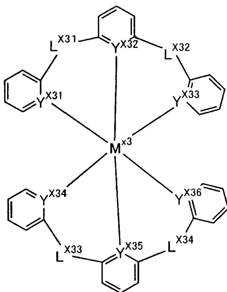
一般式 (X3)
