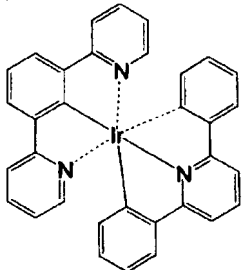
化合物 (110)
