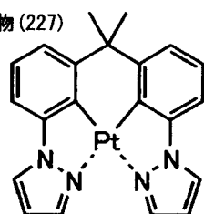
化合物 (230)
