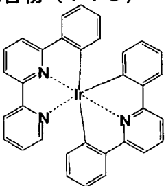
化合物 (111)
