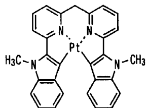
化合物(53)
