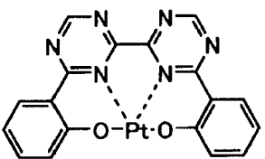
化合物 (192)
