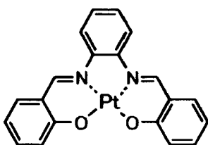
化合物 (88)
