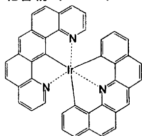
化合物 ( 9 9 )
