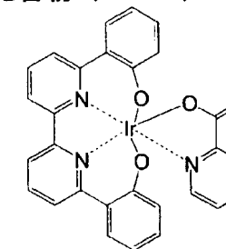
化合物 (117)
