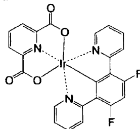
化合物 ( 1 0 6 )
