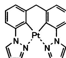
化合物 (228)
