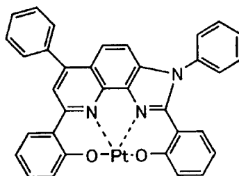
化合物 (201)
