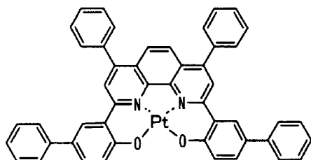
化合物(16)
