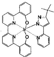
化合物 (118)
