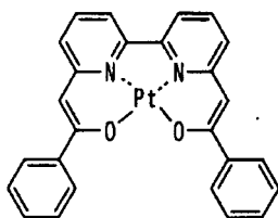
化合物(151)
