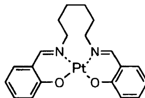
化合物 (97)
