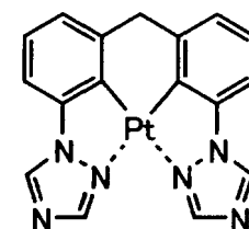
化合物 (231)
