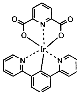
化合物 (143)
