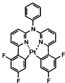
化合物 (81)
