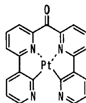
化合物(56)
