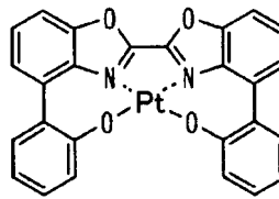
化合物(32)
