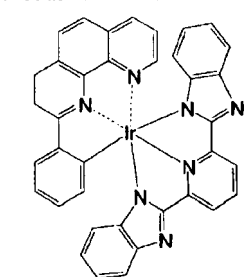
化合物 (122)
