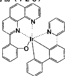
化合物 (124)
