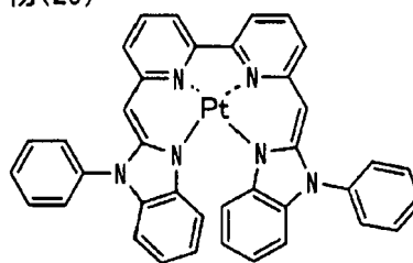
化合物(29)
