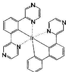
化合物 (125)
