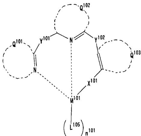
一般式(14)
