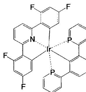
化合物 (175)
