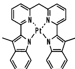
化合物(62)
