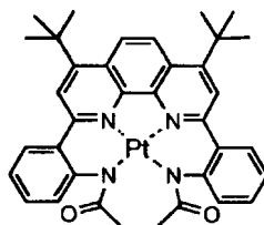
化合物 (75)
