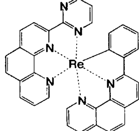
化合物 (132)
