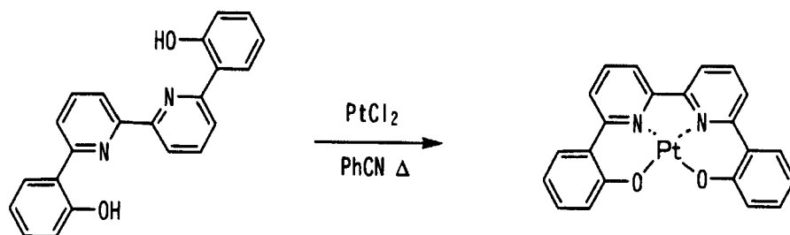
化合物(1)
