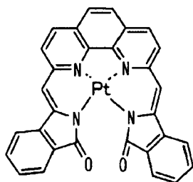
化合物(25)
