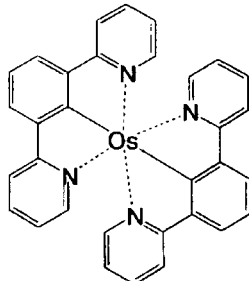
化合物 (132)
