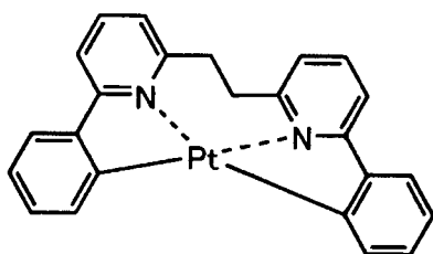
化合物 (240)
