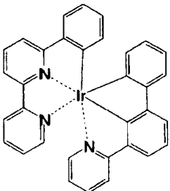
化合物 (112)
