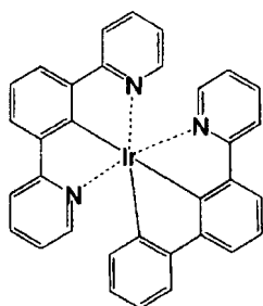
化合物 (109)
