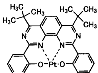
化合物 (193)
