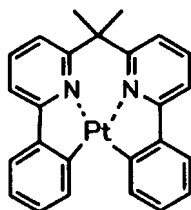
化合物 (79)
