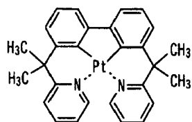
化合物(36)
