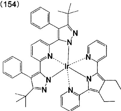
化合物(154)
