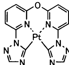
化合物 (217)
