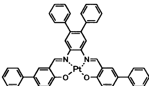
化合物 (89)
