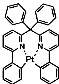
化合物 (78)
