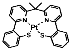
化合物 (69)
