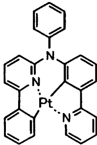
化合物 (140)
