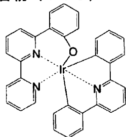
化合物 (116)
