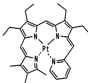
化合物(64)
