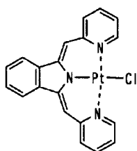
化合物(145)
