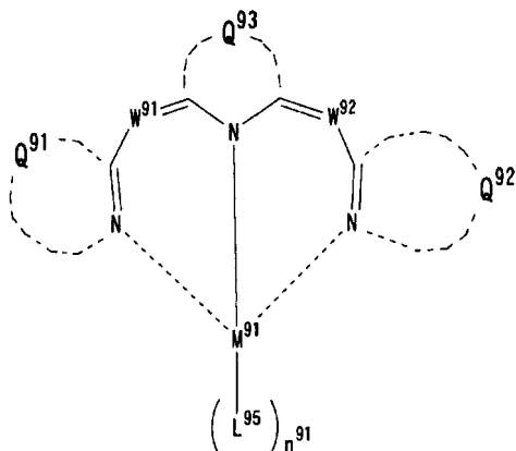
一般式(13)
