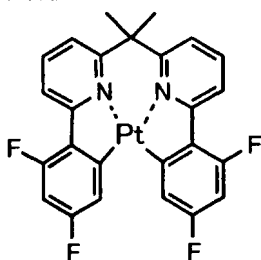
化合物 (83)
