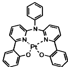
化合物 (69)
