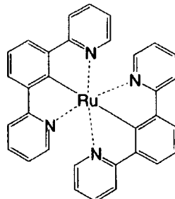
化合物 (133)
