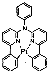
化合物 (82)
