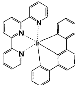
化合物 (112)
