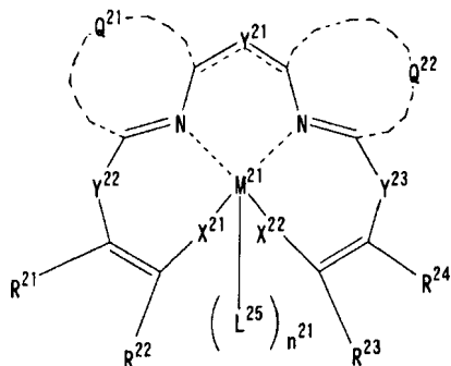
一般式(2)
