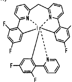
化合物(152)
