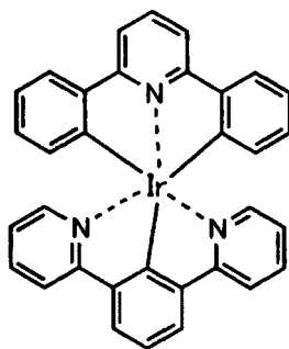
化合物 (141)
