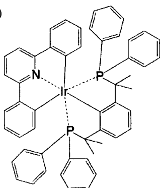
化合物 (171)
