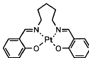
化合物 (96)
