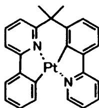
化合物 (139)
