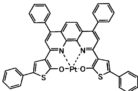
化合物 (205)
