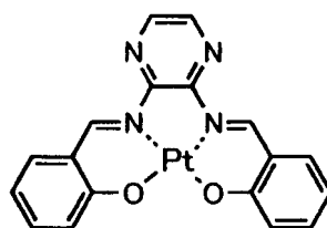
化合物 (93)
