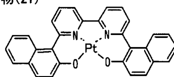
化合物(21)
