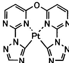
化合物 (226)
