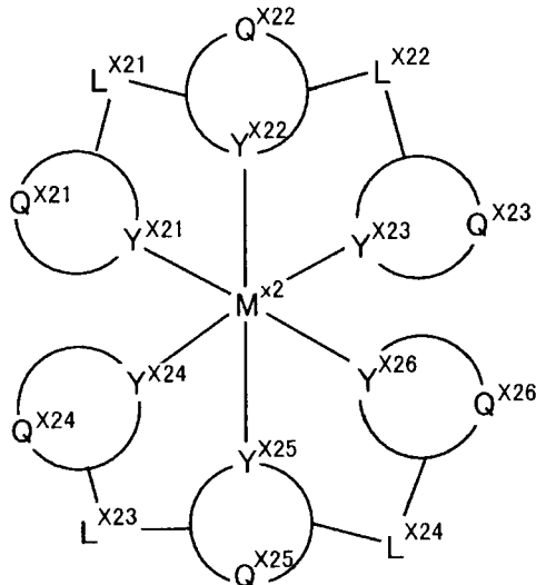
一般式 (X2)
