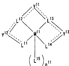
一般式(1)
