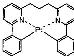
化合物 (241)
