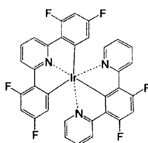
化合物 ( 1 0 4 )
