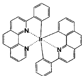
化合物 ( 1 0 1 )
