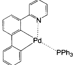
化合物 (137)
