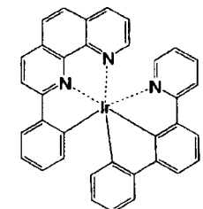
化合物 (121)
