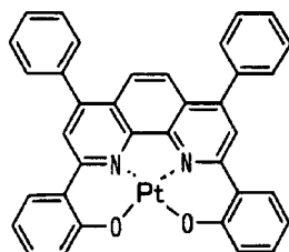
化合物(16)
