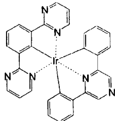
化合物 (127)
