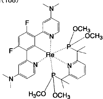
化合物(168)
