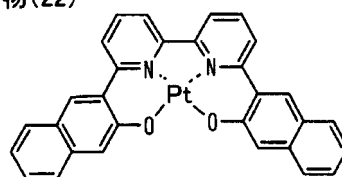
化合物(22)
