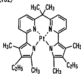
化合物(152)
