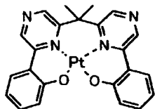
化合物 (67)
