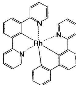
化合物 (135)
