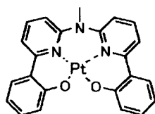
化合物 (70)
