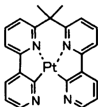
化合物 (84)
