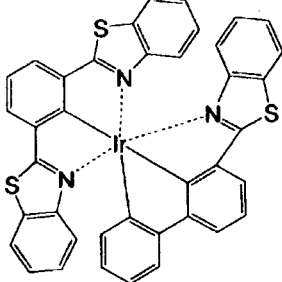
化合物 (130)
