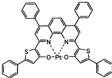
化合物 (206)
