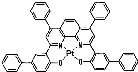
化合物(16)
