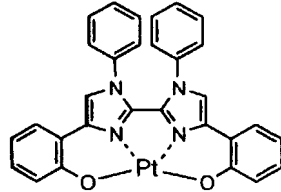
化合物 (76)
