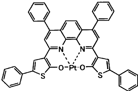
化合物 (205)
