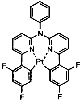
化合物 (81)
