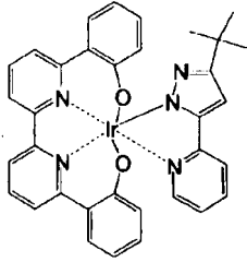
化合物 (118)
