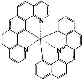
化合物 ( 9 9 )
