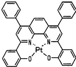
化合物(16)
