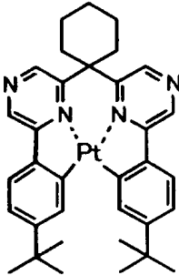
化合物 (81)
