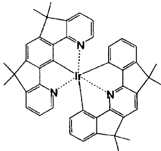
化合物 ( 1 0 0 )
