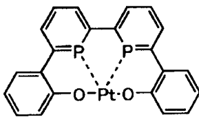
化合物 (194)
