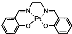
化合物 (92)
