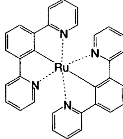
化合物 (133)
