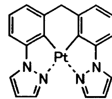
化合物 (228)
