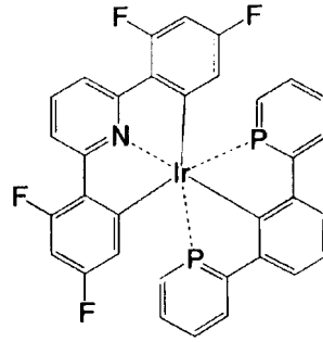
化合物 (175)
