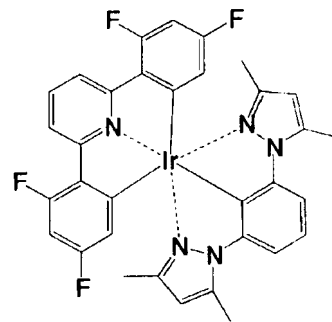
化合物 (176)
