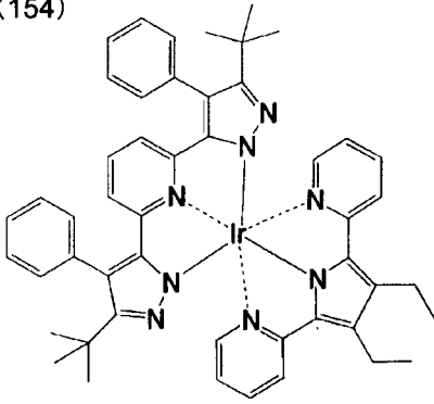
化合物(154)
