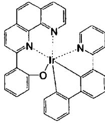
化合物 (124)
