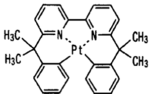
化合物(47)
