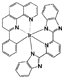
化合物 (122)
