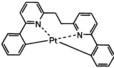
化合物(240)
