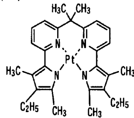
化合物(152)
