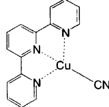
化合物 (136)
