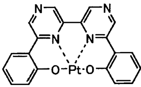
化合物 (191)
