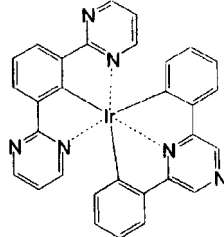
化合物 (127)
