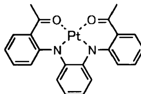
化合物 (87)
