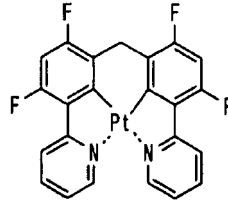
化合物(39)
