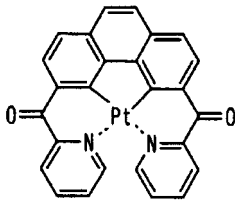
化合物(36)
