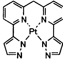
化合物 (219)
