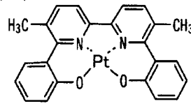
化合物(18)
