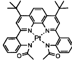
化合物 (75)
