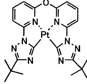
化合物 (217)
