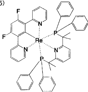
化合物(169)
