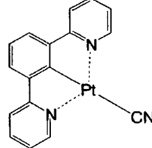
化合物 (135)
