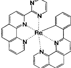
化合物 (132)
