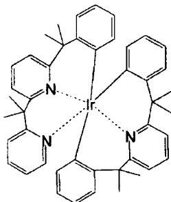
化合物 ( 1 0 2 )
