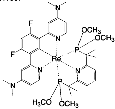
化合物(168)
