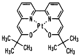
化合物(150)
