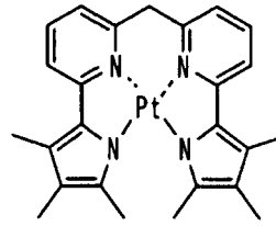
化合物(63)
