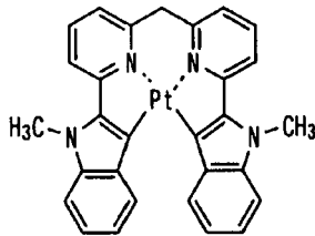
化合物(54)
