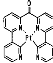
化合物(56)
