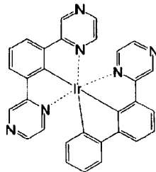
化合物 (125)
