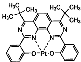
化合物 (193)
