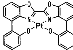
化合物(32)
