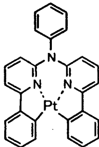
化合物 (82)
