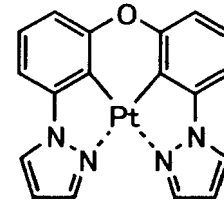
化合物 (229)
