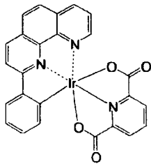
化合物 (122)
