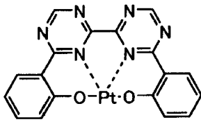
化合物 (192)
