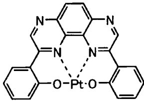
化合物 (191)
