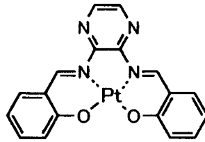
化合物 (93)
