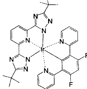
化合物 ( 1 0 7 )
