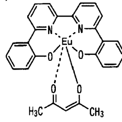
化合物(8)
