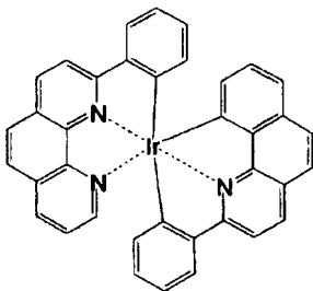
化合物 ( 1 0 1 )
