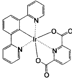
化合物 (114)
