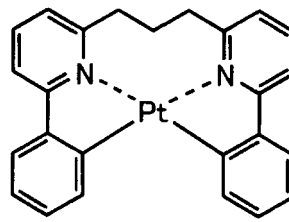
化合物(241)
