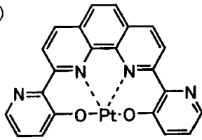
化合物 (203)
