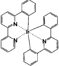
化合物 (111)
