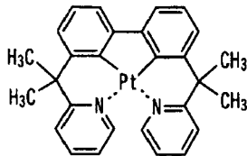
化合物(36)
