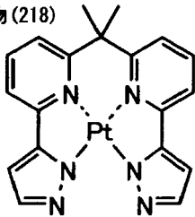
化合物 (221)
