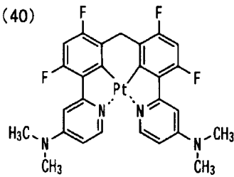
化合物(41)
