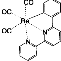
化合物 (131)
