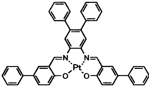
化合物 (89)
