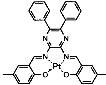
化合物 (94)
