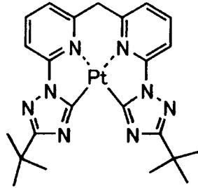
化合物 (216)
