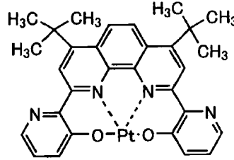
化合物 (208)
