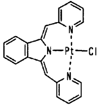
化合物(145)
