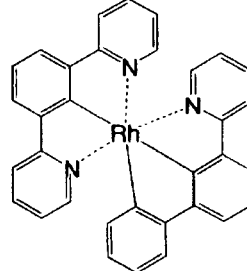
化合物 (134)
