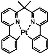
化合物 (79)
