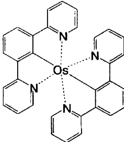
化合物 (132)
