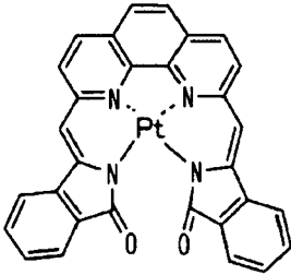
化合物(25)
