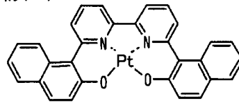
化合物(21)
