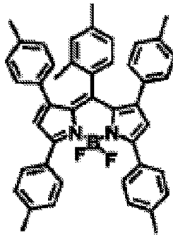
化合物(7)-46
