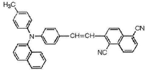
化合物(9)-10
