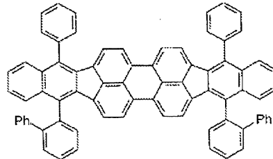
化合物(5)-8
