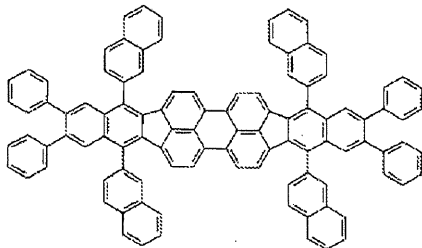
化合物(5)-5
