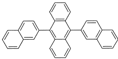
構造式(103) ADN
