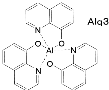
構造式(105)
