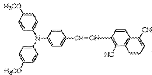
化合物(9)-8
