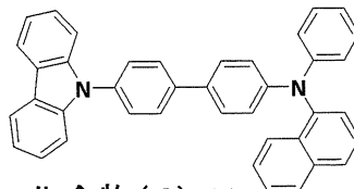
化合物(4)-11
