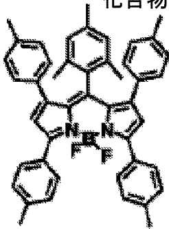
化合物(7)-45
