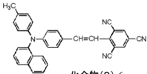
化合物(9)-6
