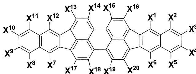
一般式 (5)
