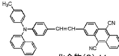
化合物(9)-14
