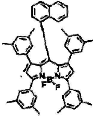
化合物(7)-65
