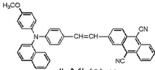
化合物(9)-13
