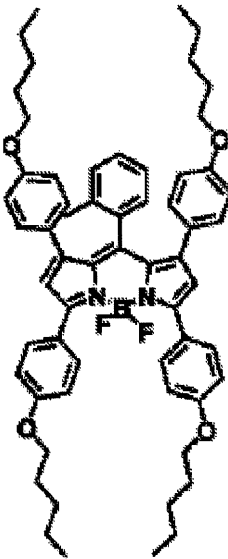
化合物(7)-40
