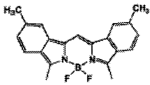
化合物(7)-7
