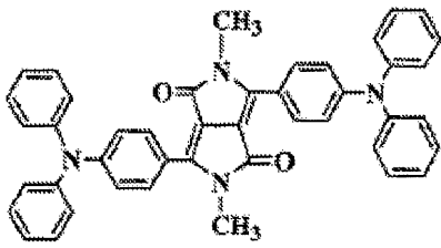
化合物(6)-1
