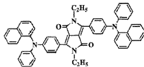
化合物(6)-8
