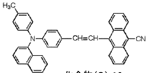
化合物(9)-15
