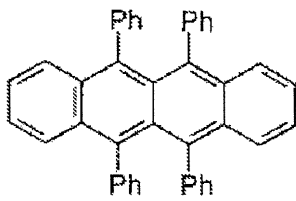
化合物(1)-1
