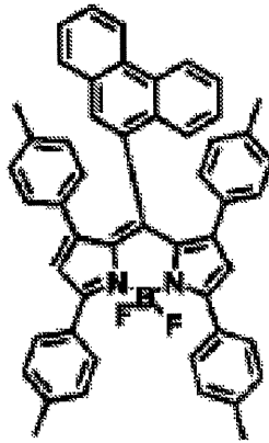
化合物(7)-53
