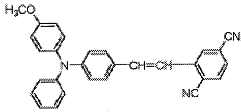
化合物(9)-1
