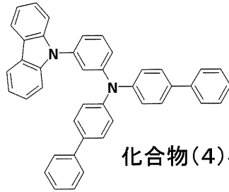
化合物(4)-4
