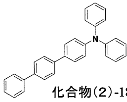
化合物(2)-19
