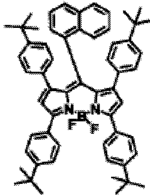
化合物(7)-67
