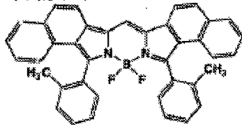
化合物(7)-11
