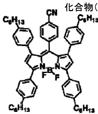
化合物(7)-26
