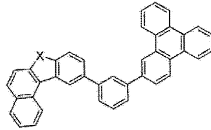
化合物 52
