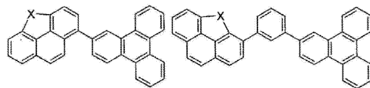
化合物 63
