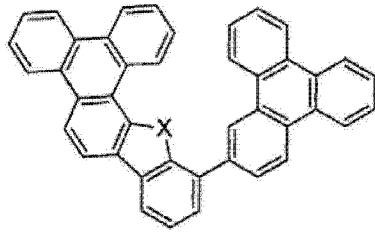
化合物 57
