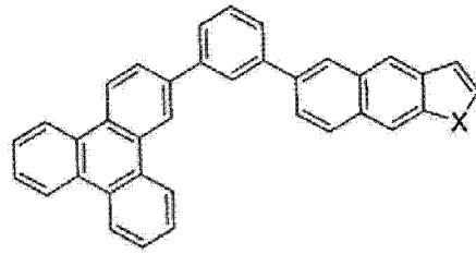
化合物 26
