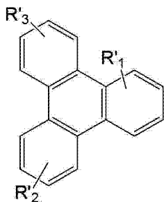
式 I。
