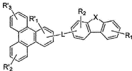
式 4
