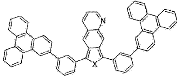
化合物 18
