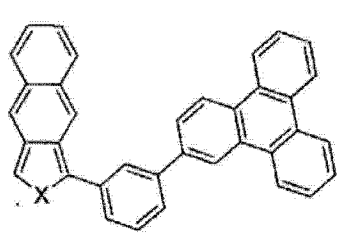
化合物 11
