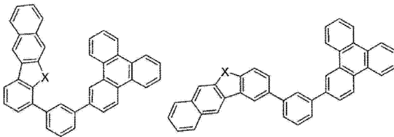
化合物 47
