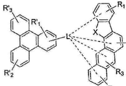
式 4-13
