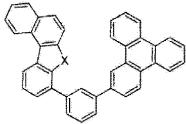
化合物 51
