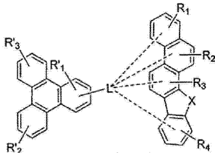
式 4-12
