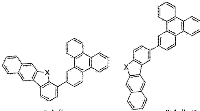
化合物 45
