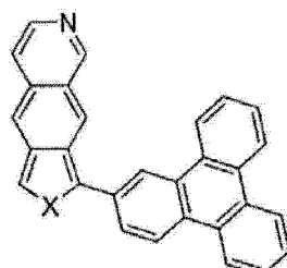
化合物 9
