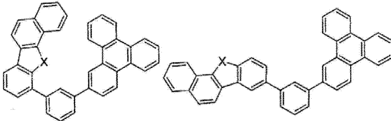
化合物 44
