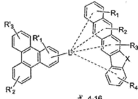
式 4-16
