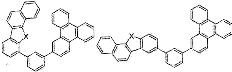
化合物 43
