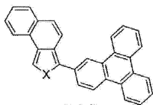
化合物 5
