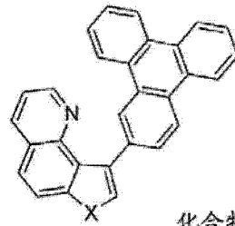
化合物 30
