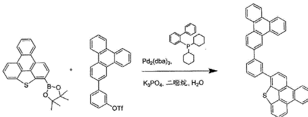
化合物 67S
