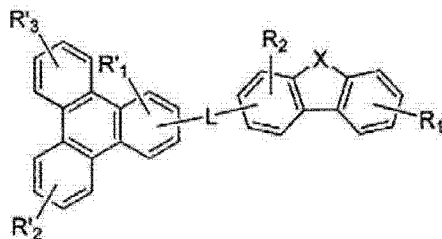
式 4
