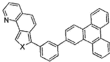
化合物 19
