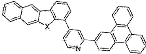
化合物 34
