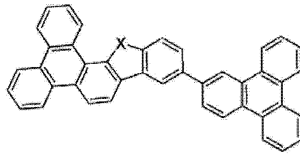
化合物 58
