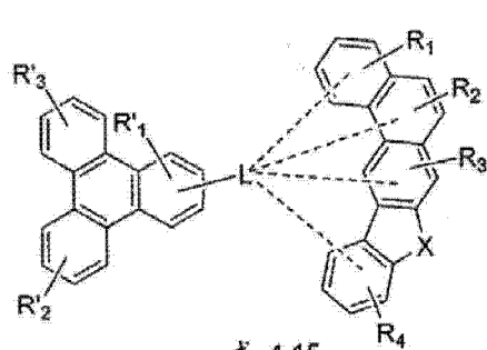
式 4-15
