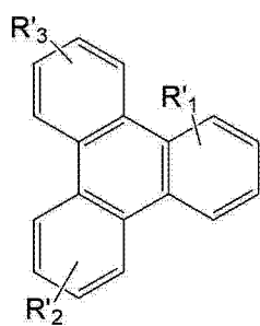
式 I。
