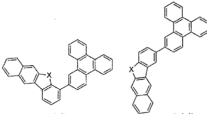
化合物 45
