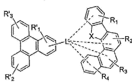
式 4-14
