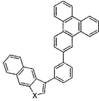
化合物 25
