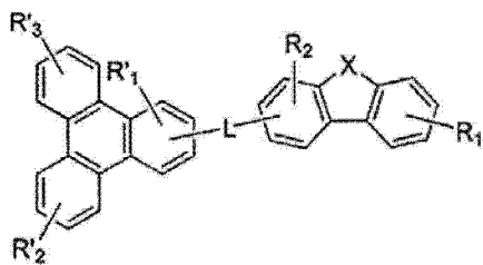
式 4
