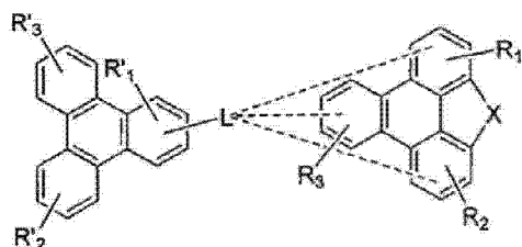
式 4-28
