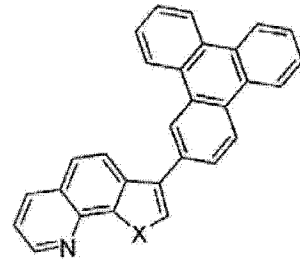
化合物 29
