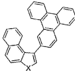
化合物 24
