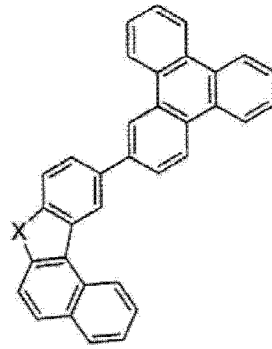
化合物 50
