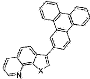
化合物 29
