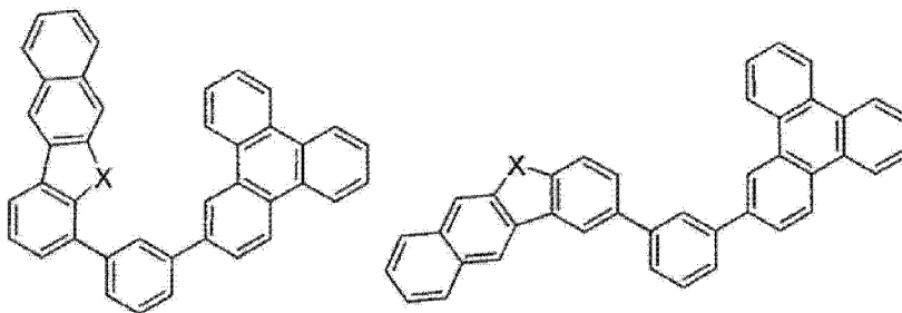
化合物 47
