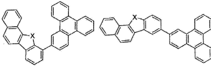
化合物 41
