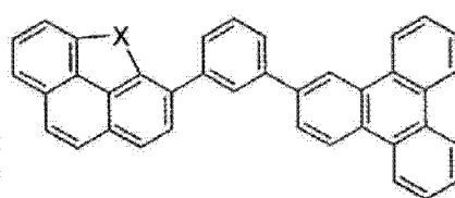
化合物 63
