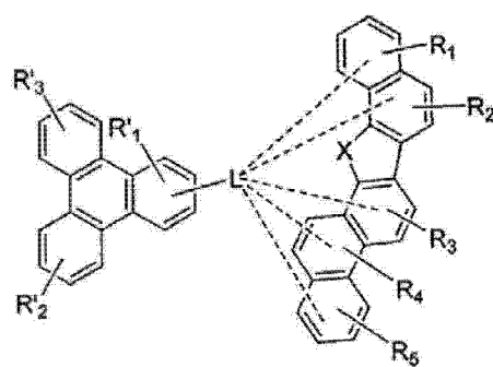
式 4-26
