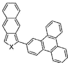
化合物 3
