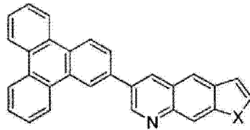
化合物 27
