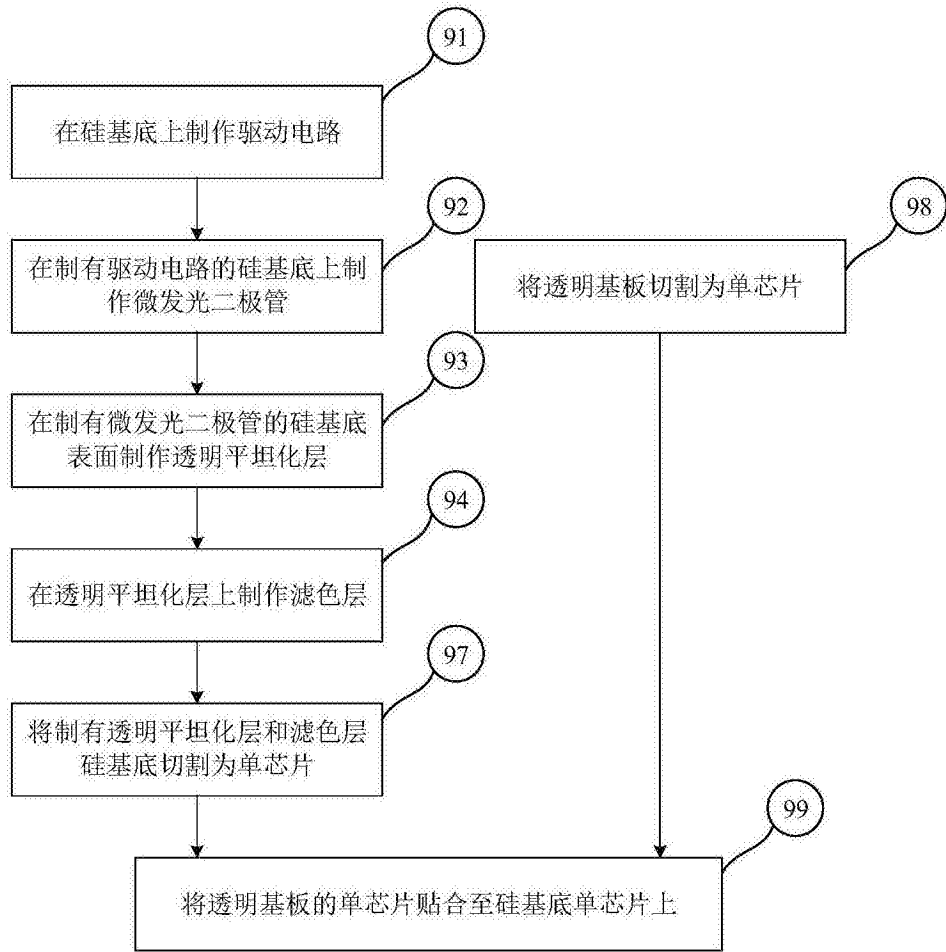
图10 (b)
