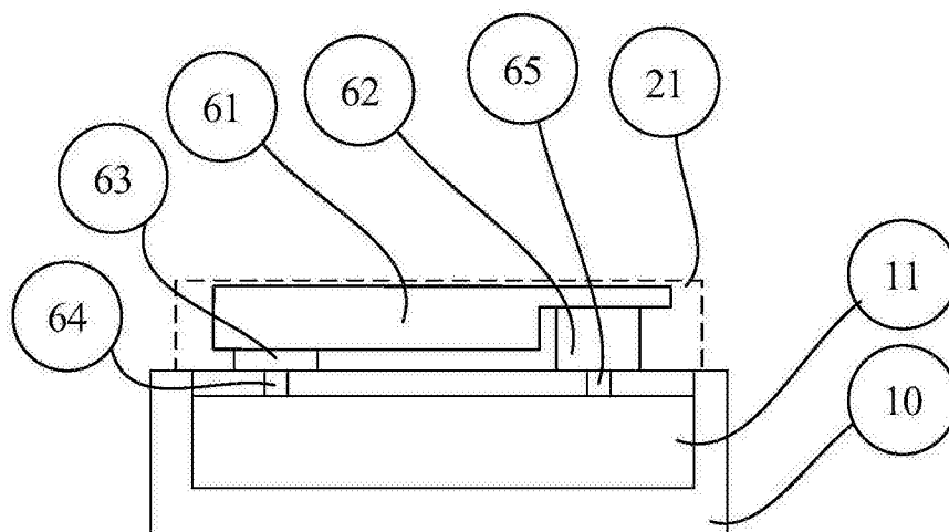
图8(a)
