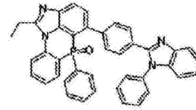
化学式 2-9-9
