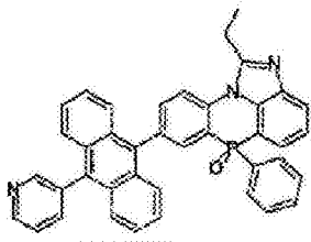
化学式 2-3-10
