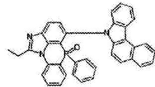
化学式 2-9-15
