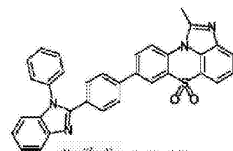
化学式 1-2-45
