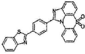
化学式 1-5-46
