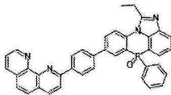
化学式 2-3-47
