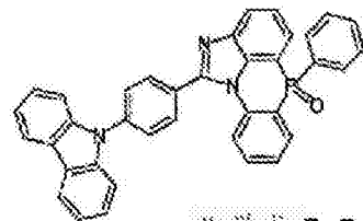
化学式 2-5-42
