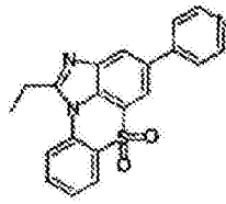
化学式 1-10-2
