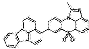
化学式 1-2-30
