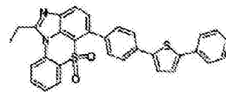
化学式 1-9-3
