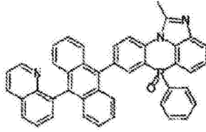
化学式 2-2-11
