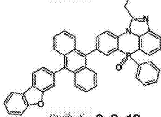
化学式 2-3-13
