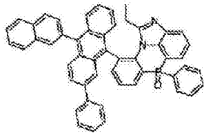
化学式 2-8-16
