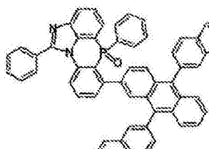
化学式 2-6-20
