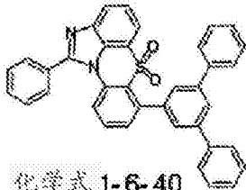
化学式 1-6-37
