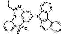
化学式 1-10-15
