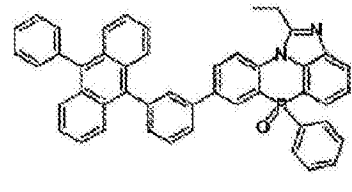
化学式 2-3-18
