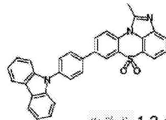
化学式 1-2-42
