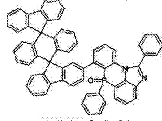
化学式 2-6-36
