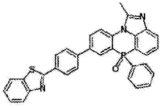
化学式 2-2-46
