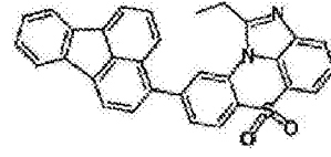
化学式 1-7-30
