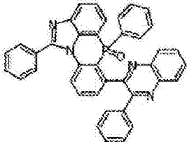
化学式 2-6-49
