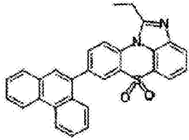
化学式 1-3-31
