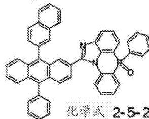
化学式 2-5-20
