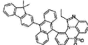
化学式 1-8-5
