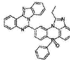
化学式 2-7-53
