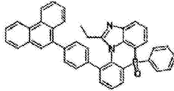
化学式 2-8-32
