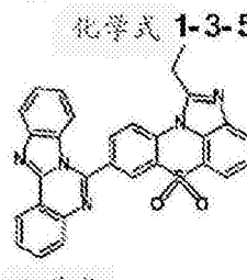
化学式 1-3-53
