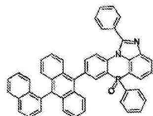
化学式 2-4-3
