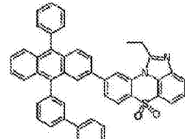
化学式 1-7-24
