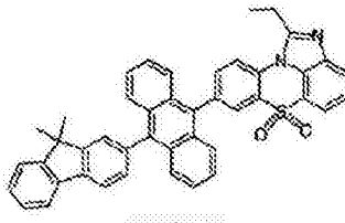
化学式 1-3-5
