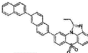
化学式 1-7-44
