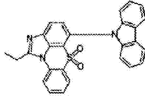
化学式 1-9-14
