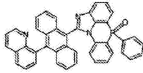
化学式 2-5-11
