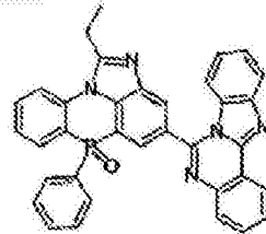
化学式 2-10-17
