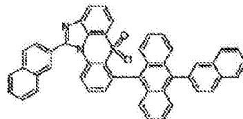
化学式 1-6-2
