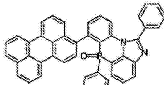
化学式 2-6-29
