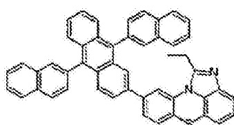
化学式 1-7-20
