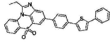
化学式 1-10-3
