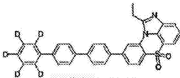
化学式 1-7-52
