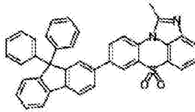
化学式 1-2-35
