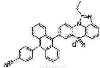
化学式 1-3-12
