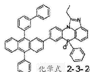
化学式 2-3-21
