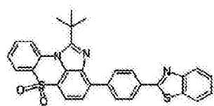
化学式 1-11-10
