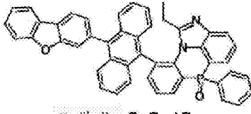
化学式 2-8-13
