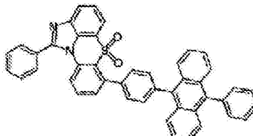
化学式 1-6-17
