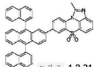
化学式 1-2-21
