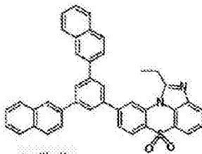
化学式 1-7-43
