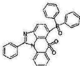
化学式 1-12-7
