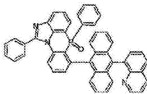
化学式 2-6-11
