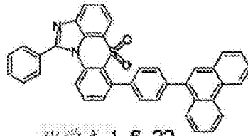
化学式 1-6-32
