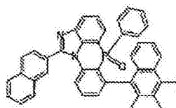
化学式 2-6-4
