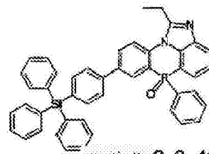
化学式 2-3-48
