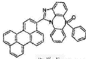
化学式 2-5-29
