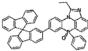
化学式 2-3-34
