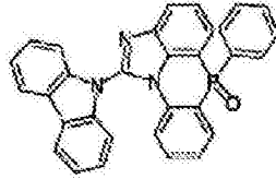
化学式 2-5-50
