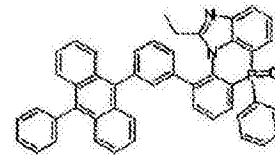
化学式 2-8-18
