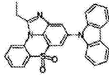
化学式 1-10-14
