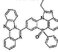
化学式 2-3-53
