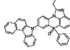
化学式 2-3-51
