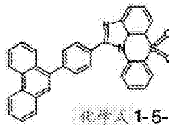
化学式 1-5-29
