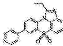
化学式 1-3-38
