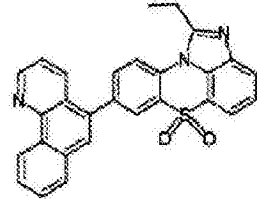
化学式 1-3-33
