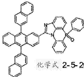
化学式 2-5-19
