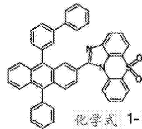
化学式 1-5-21
