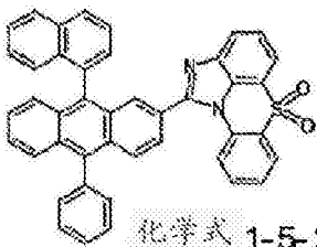
化学式 1-5-19
