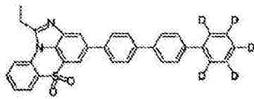
化学式 1-10-16
