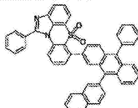
化学式 1-6-23
