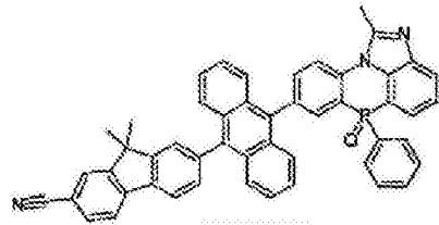
化学式 2-2-15
