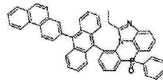
化学式 2-8-9
