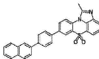
化学式 1-2-26
