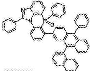
化学式 2-6-22
