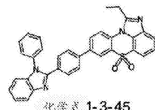
化学式 1-3-45
