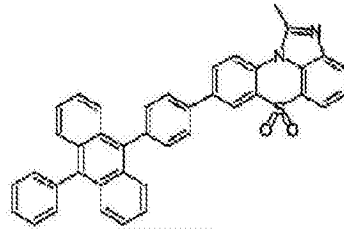
化学式 1-2-17
