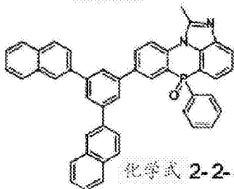
化学式 2-2-40
