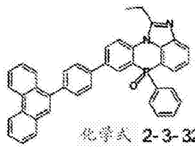
化学式 2-3-29
