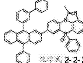
化学式 2-2-21
