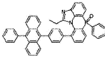
化学式 2-8-17
