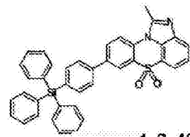
化学式 1-2-48
