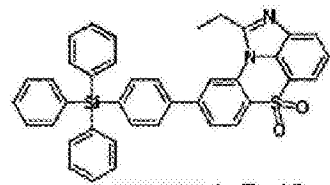
化学式 1-7-48
