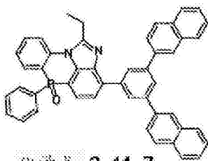
化学式 2-11-7
