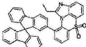
化学式 1-8-34
