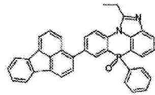
化学式 2-3-30
