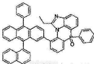
化学式 2-8-22
