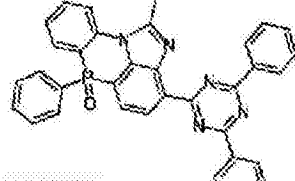
化学式 2-11-5
