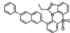
化学式 1-8-27
