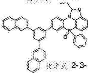
化学式 2-3-40
