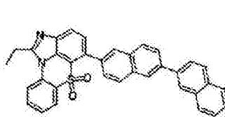
化学式 1-9-8
