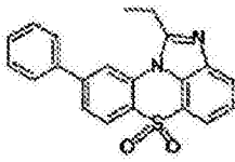
化学式 1-7-37
