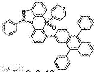
化学式 2-6-19
