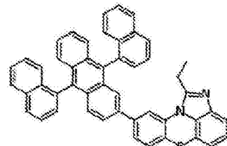
化学式 1-7-21
