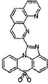
化学式 1-1-6
