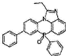
化学式 2-3-37
