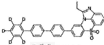
化学式 1-7-52
