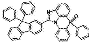
化学式 2-5-35
