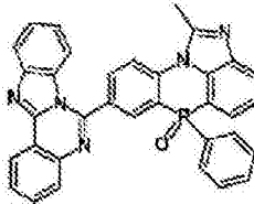
化学式 2-2-53
