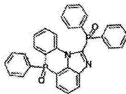
化学式 2-12-5
