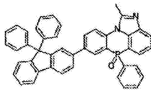
化学式 2-2-35
