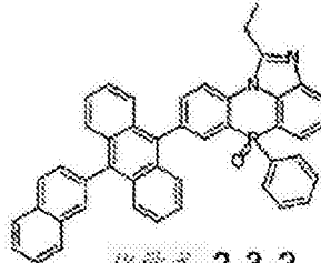
化学式 2-3-2
