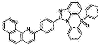
化学式 2-5-47
