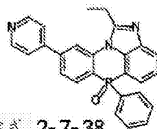
化学式 2-7-38
