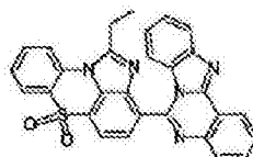
化学式 1-11-17
