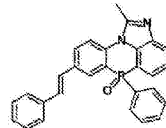
化学式 2-2-54
