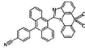
化学式 1-5-12
