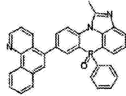
化学式 2-2-33
