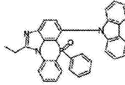
化学式 2-9-14
