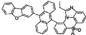
化学式 1-8-13
