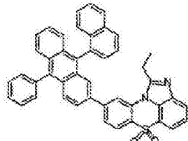
化学式 1-7-22
