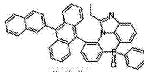
化学式 2-8-2
