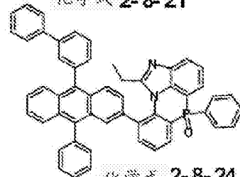
化学式 2-8-24
