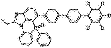
化学式 2-9-16
