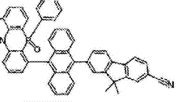
化学式 2-6-15
