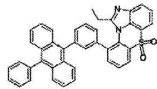
化学式 1-8-18
