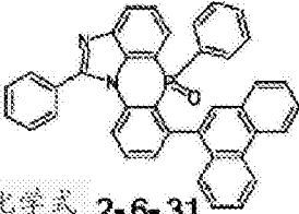
化学式 2-6-31
