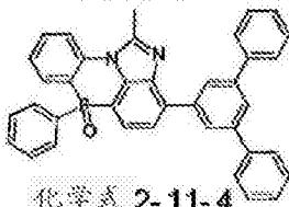
化学式 2-11-4
