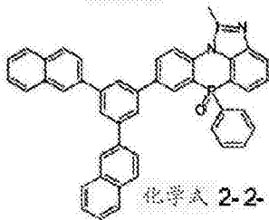
化学式 2-2-40
