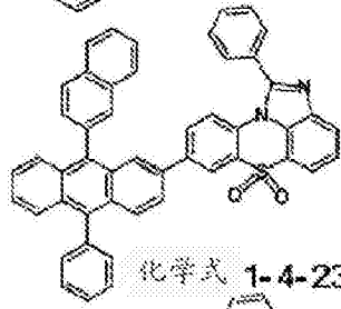
化学式 1-4-20
