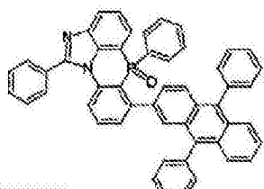
化学式 2-6-19
