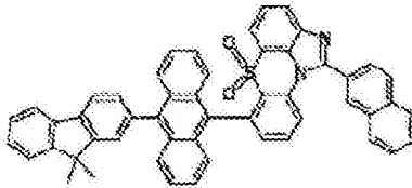
化学式 1-6-5
