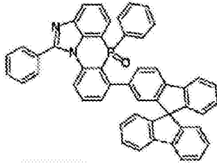
化学式 2-6-34
