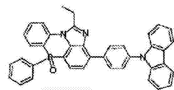
化学式 2-11-6
