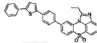
化学式 1-7-39
