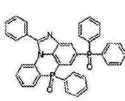
化学式 2-12-8
