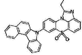
化学式 1-3-51
