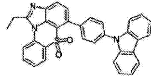
化学式 1-9-6
