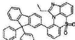
化学式 1-8-35
