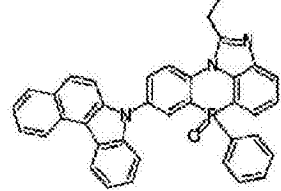
化学式 2-3-51
