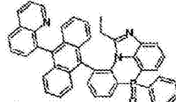
化学式 2-8-11
