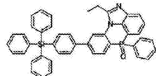
化学式 2-7-48
