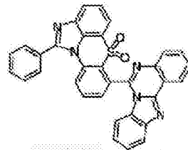
化学式 1-6-53
