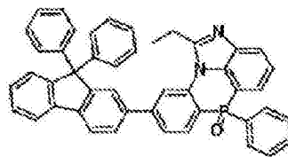
化学式 2-7-35
