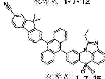
化学式 1-7-15
