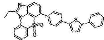
化学式 1-9-3
