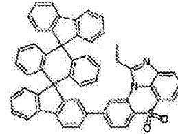
化学式 1-7-36
