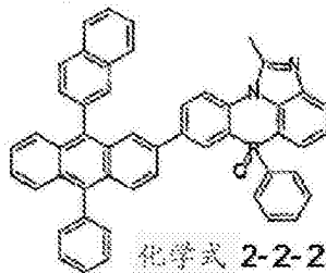
化学式 2-2-20
