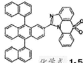
化学式 1-5-21
