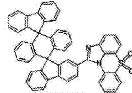
化学式 1-5-36
