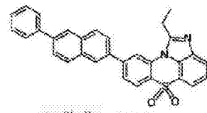
化学式 1-7-27
