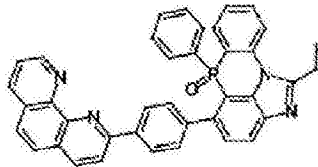
化学式 2-9-11
