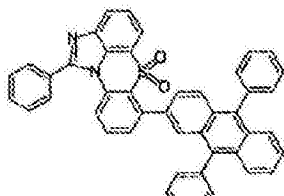
化学式 1-6-19
