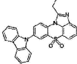
化学式 1-3-50
