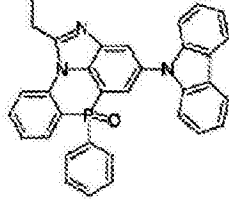
化学式 2-10-14
