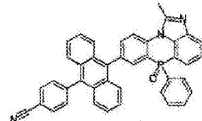
化学式 2-2-12
