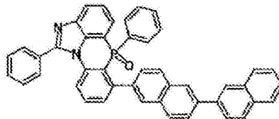
化学式 2-6-44
