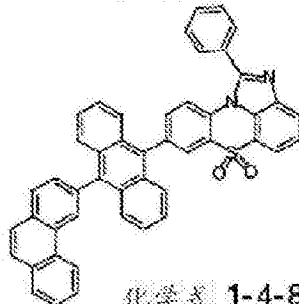
化学式 1-4-5
