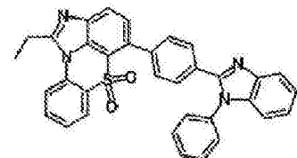
化学式 1-9-9
