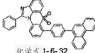
化学式 1-6-32
