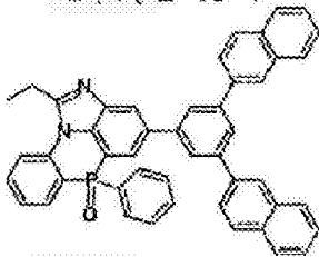
化学式 2-10-7
