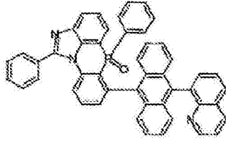
化学式 2-6-11
