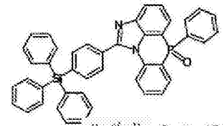
化学式 2-5-48
