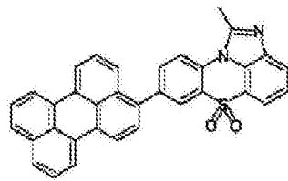
化学式 1-2-29
