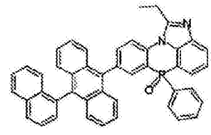
化学式 2-3-3
