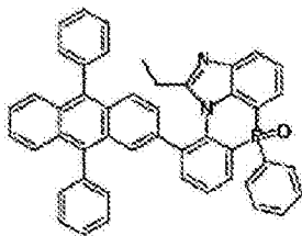
化学式 2-8-19
