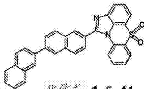
化学式 1-5-44
