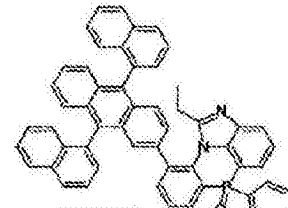
化学式 2-8-21
