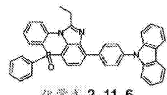
化学式 2-11-6
