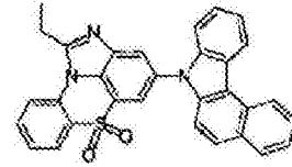
化学式 1-10-15
