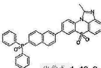
化学式 1-12-2
