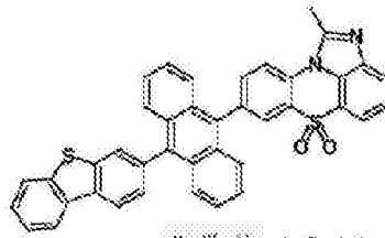
化学式 1-2-14
