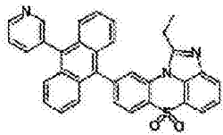
化学式 1-7-10
