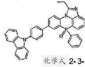
化学式 2-3-39
