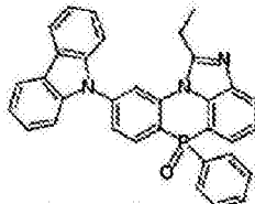
化学式 2-7-50
