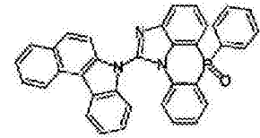
化学式 2-5-51
