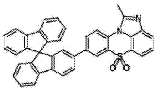
化学式 1-2-34
