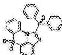
化学式 1-12-5
