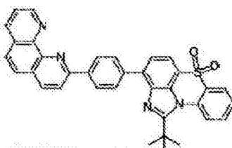
化学式 1-11-11
