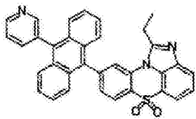
化学式 1-7-10
