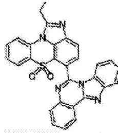
化学式 1-9-17
