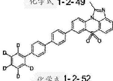
化学式 1-2-52
