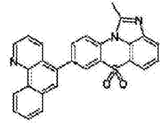
化学式 1-2-33
