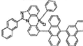
化学式 2-6-7
