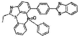
化学式 2-9-10
