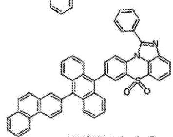
化学式 1-4-9
