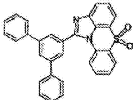
化学式 1-5-40
