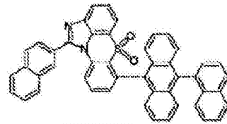
化学式 1-6-3
