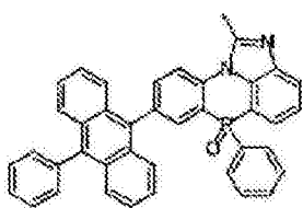
化学式 2-2-1
