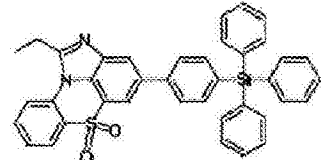
化学式 1-10-12
