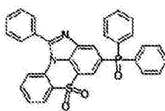
化学式 1-12-8
