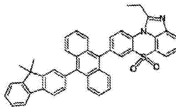
化学式 1-3-5
