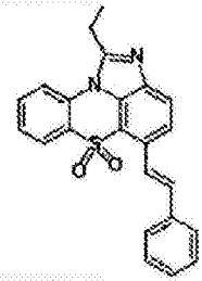
化学式 1-9-18
