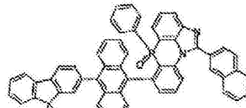
化学式 2-6-5
