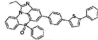
化学式 2-10-3
