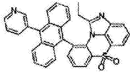
化学式 1-8-10
