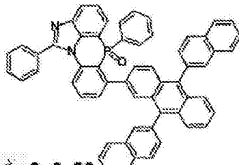
化学式 2-6-20
