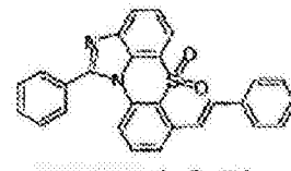
化学式 1-6-54
