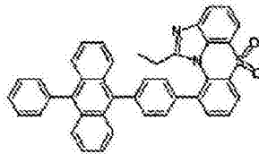
化学式 1-8-17
