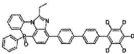
化学式 2-11-16
