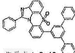
化学式 1-6-40
