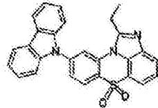
化学式 1-7-50
