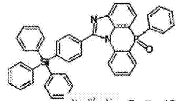
化学式 2-5-48
