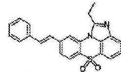
化学式 1-7-54
