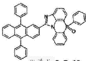
化学式 2-5-19
