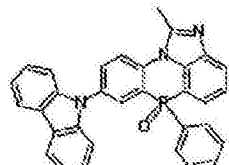
化学式 2-2-50
