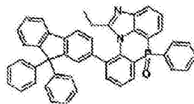
化学式 2-8-35
