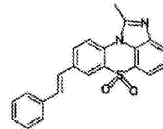
化学式 1-2-54
