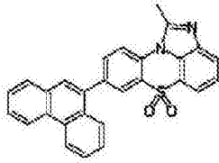
化学式 1-2-31
