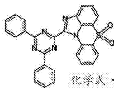
化学式 1-5-38
