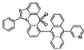
化学式 1-6-10
