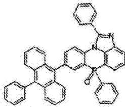
化学式 2-4-1
