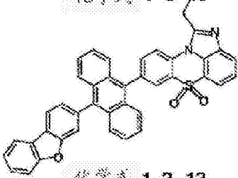
化学式 1-3-13
