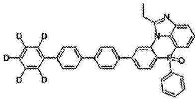
化学式 2-7-52
