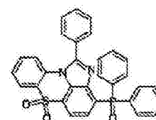
化学式 1-12-6
