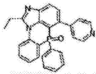
化学式 2-9-2
