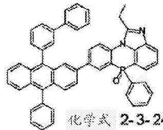
化学式 2-3-21
