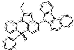
化学式 2-11-15
