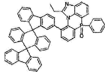
化学式 2-8-36
