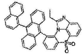
化学式 1-8-3
