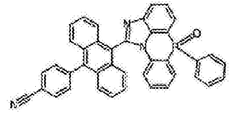
化学式 2-5-12
