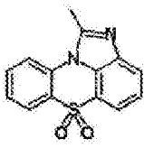
化学式 1-1-1
