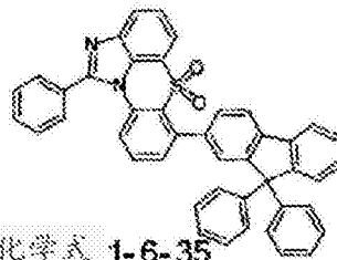
化学式 1-6-35
