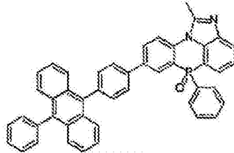
化学式 2-2-17
