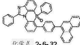
化学式 2-6-32
