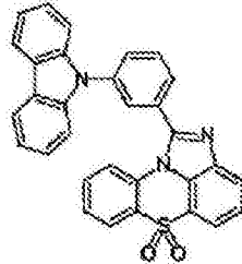
化学式 1-1-7
