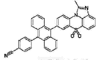
化学式 1-2-12
