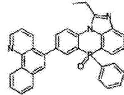
化学式 2-3-33
