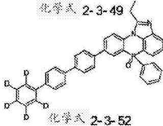
化学式 2-3-52
