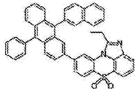
化学式 1-7-23
