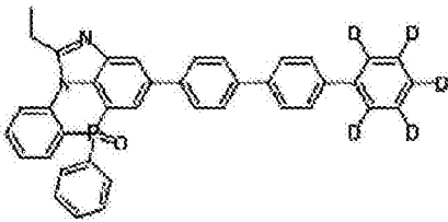
化学式 2-10-16
