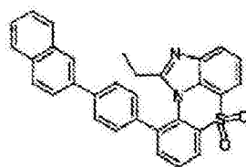
化学式 1-8-26
