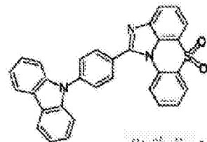
化学式 1-5-42
