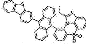
化学式 1-8-14
