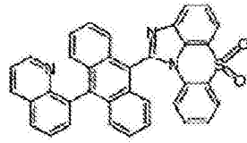
化学式 1-5-11
