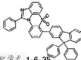
化学式 1-6-35
