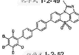
化学式 1-2-52
