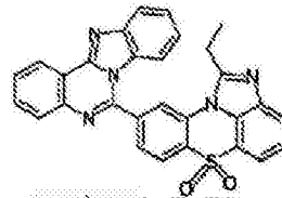
化学式 1-7-53
