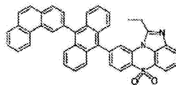
化学式 1-7-8
