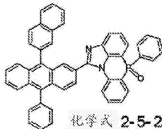
化学式 2-5-20
