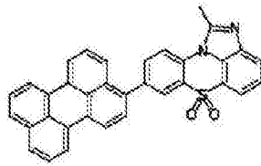
化学式 1-2-29
