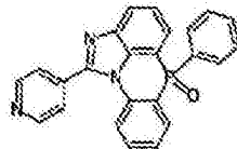
化学式 2-5-38
