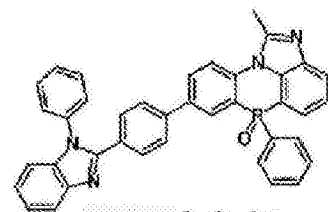
化学式 2-2-45
