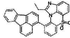
化学式 1-8-30
