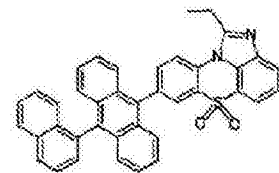
化学式 1-3-3
