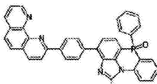
化学式 2-11-11
