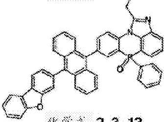
化学式 2-3-13
