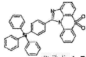
化学式 1-5-48
