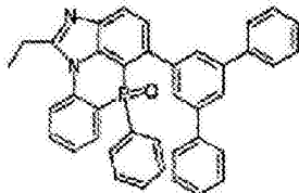
化学式 2-9-4
