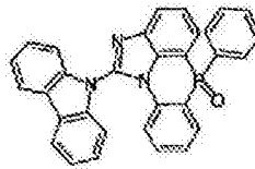
化学式 2-5-50
