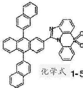
化学式 1-5-19
