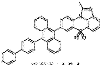
化学式 1-2-4
