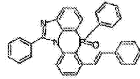
化学式 2-6-54
