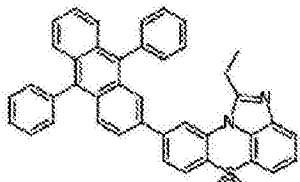
化学式 1-7-19
