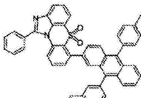
化学式 1-6-20
