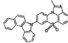
化学式 1-2-51
