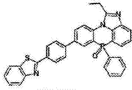
化学式 2-3-46
