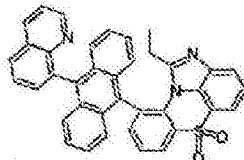
化学式 1-8-11
