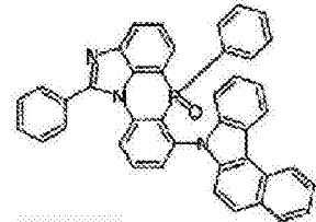
化学式 2-6-51
