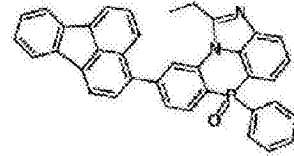
化学式 2-7-30
