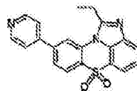
化学式 1-7-38
