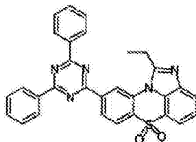
化学式 1-7-41
