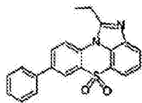
化学式 1-3-37
