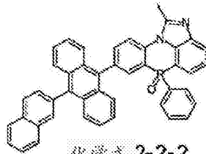
化学式 2-2-2
