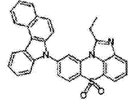
化学式 1-7-51
