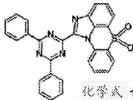
化学式 1-5-38
