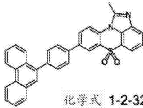
化学式 1-2-29
