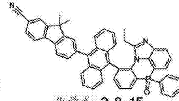
化学式 2-8-15
