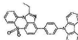
化学式 1-11-6
