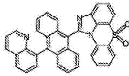
化学式 1-5-11
