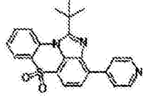
化学式 1-11-2
