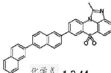
化学式 1-2-44
