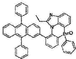
化学式 2-8-19
