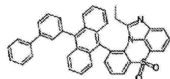
化学式 1-8-6
