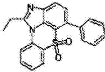
化学式 1-9-1
