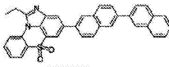
化学式 1-10-8
