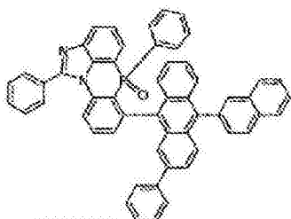
化学式 2-6-16
