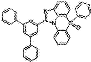
化学式 2-5-40
