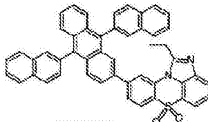
化学式 1-7-20
