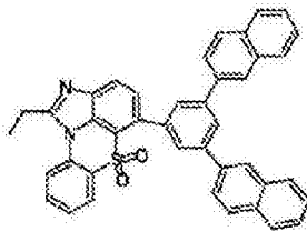
化学式 1-9-7
