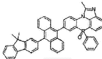
化学式 2-2-5
