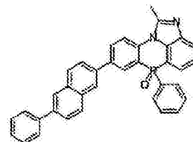
化学式 2-2-27
