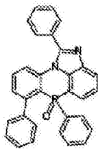
化学式 2-6-37
