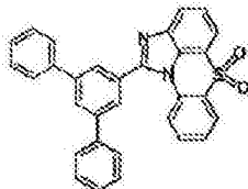
化学式 1-5-40
