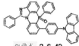
化学式 2-6-42
