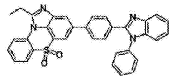
化学式 1-10-9
