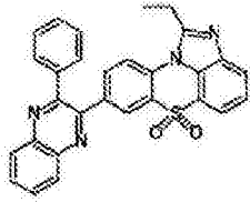
化学式 1-3-49
