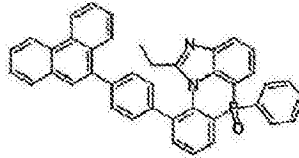
化学式 2-8-32
