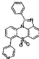
化学式 1-6-38
