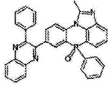
化学式 2-2-49
