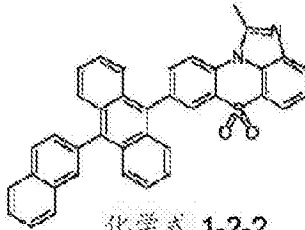
化学式 1-2-2
