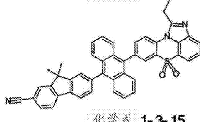
化学式 1-3-15
