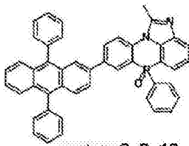
化学式 2-2-19
