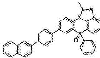
化学式 2-2-26
