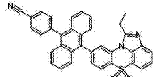
化学式 1-7-12
