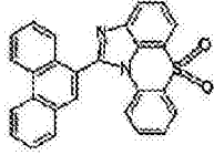
化学式 1-5-31
