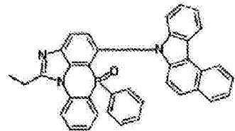
化学式 2-9-15
