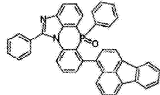
化学式 2-6-30
