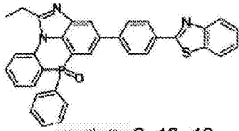
化学式 2-10-10
