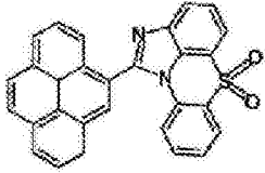
化学式 1-5-28
