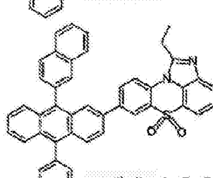
化学式 1-3-23
