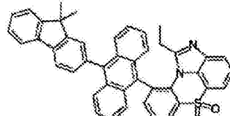
化学式 1-8-5
