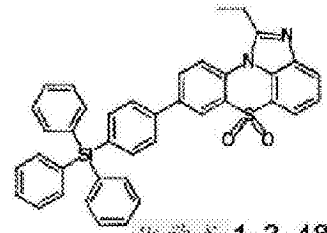
化学式 1-3-48
