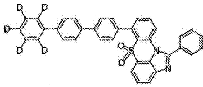
化学式 1-6-52
