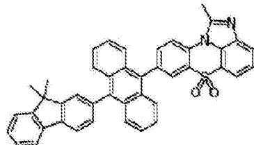
化学式 1-2-5
