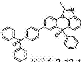
化学式 2-12-1
