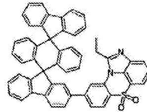
化学式 1-7-36
