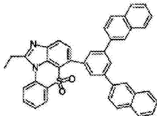
化学式 1-9-7
