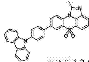
化学式 1-2-42
