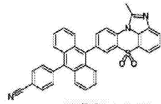
化学式 1-2-12
