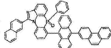
化学式 2-6-9
