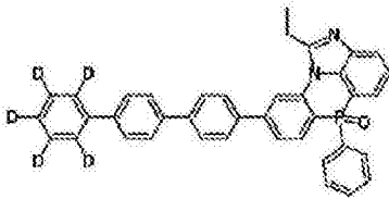
化学式 2-7-52
