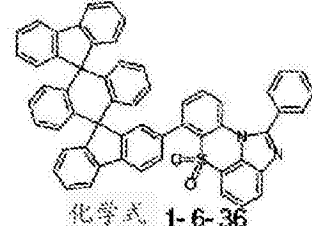
化学式 1-6-36
