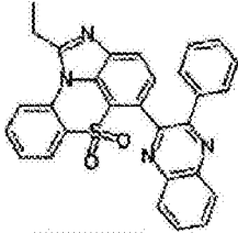
化学式 1-9-13
