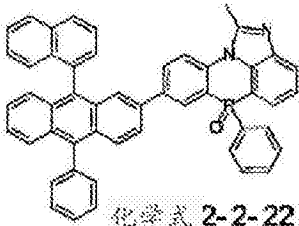
化学式 2-2-22
