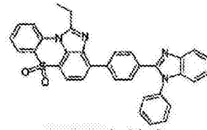
化学式 1-11-9
