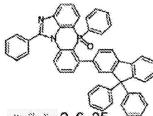
化学式 2-6-35
