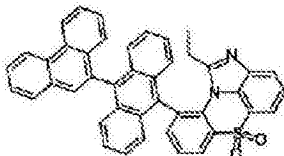
化学式 1-8-7
