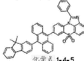
化学式 1-4-5
