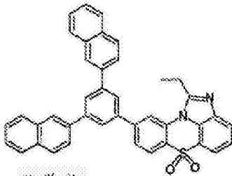
化学式 1-7-43
