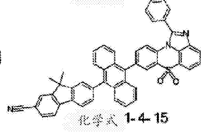
化学式 1-4-12
