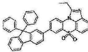
化学式 1-3-35
