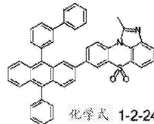
化学式 1-2-21
