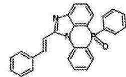
化学式 2-5-54
