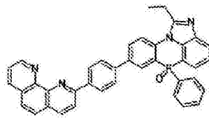
化学式 2-3-47
