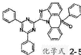
化学式 2-5-38
