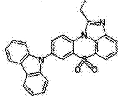
化学式 1-3-50
