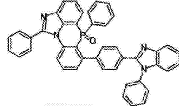
化学式 2-6-45
