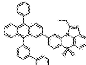
化学式 1-7-24
