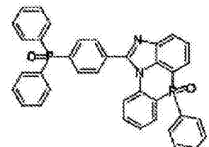
化学式 2-12-3
