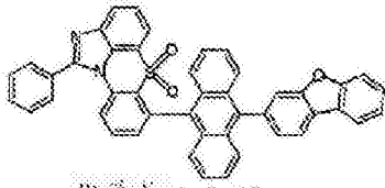
化学式 1-6-13
