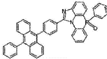
化学式 2-5-17
