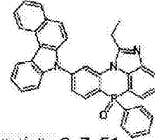
化学式 2-7-51
