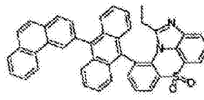
化学式 1-8-8
