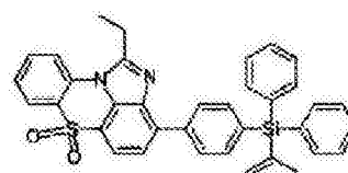
化学式 1-11-12
