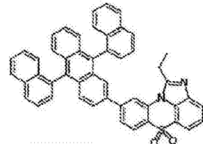
化学式 1-7-21
