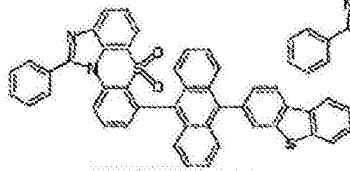
化学式 1-6-14
