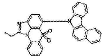
化学式 1-9-15
