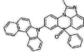
化学式 2-2-51
