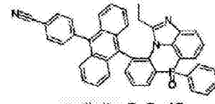
化学式 2-8-12
