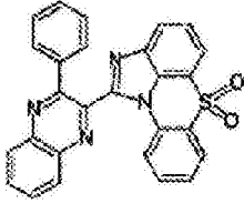
化学式 1-5-49
