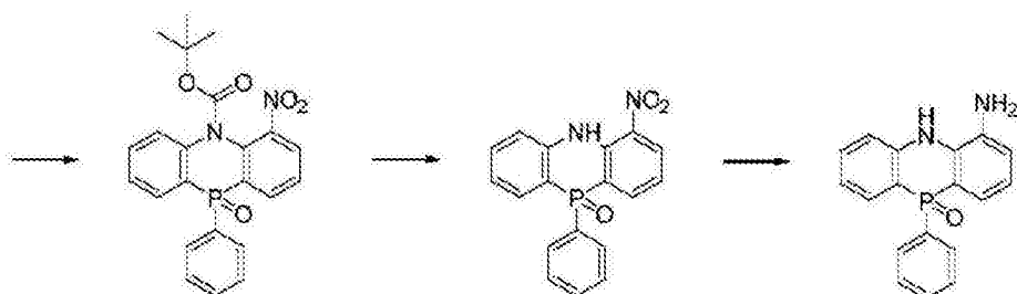
[化合物 2-1-A]
