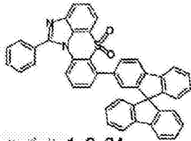
化学式 1-6-34
