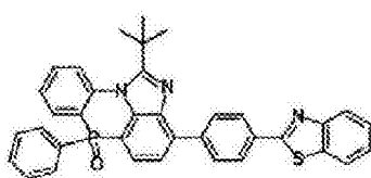
化学式 2-11-10
