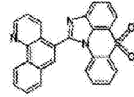
化学式 1-5-33
