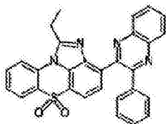
化学式 1-11-13
