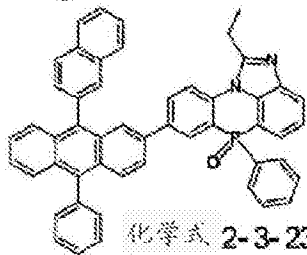
化学式 2-3-20
