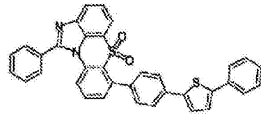
化学式 1-6-39
