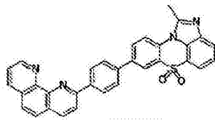
化学式 1-2-47
