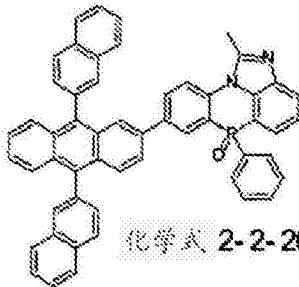
化学式 2-2-17
