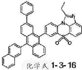
化学式 1-3-13
