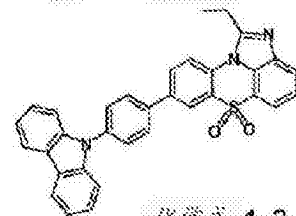
化学式 1-3-42
