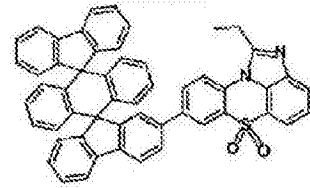
化学式 1-3-36
