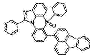
化学式 2-6-30
