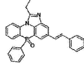
化学式 2-10-18
