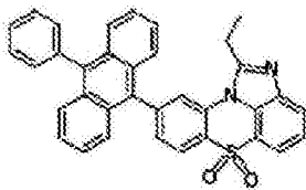
化学式 1-7-1
