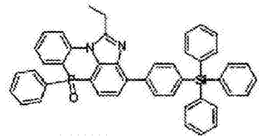
化学式 2-11-12
