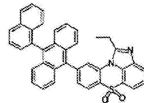
化学式 1-7-3
