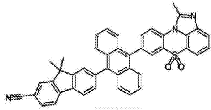
化学式 1-2-15
