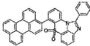
化学式 1-6-29
