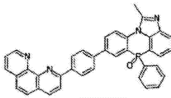
化学式 2-2-47
