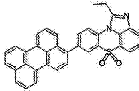
化学式 1-3-29
