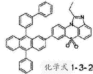
化学式 1-3-21
