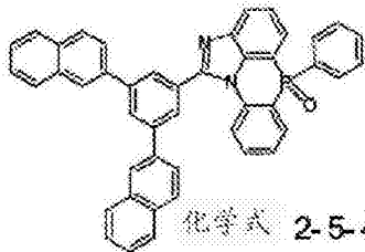
化学式 2-5-40
