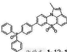
化学式 1-12-1
