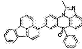
化学式 2-2-30
