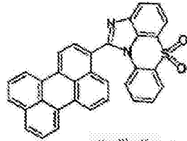
化学式 1-5-29
