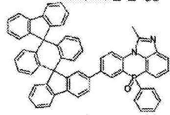
化学式 2-2-36
