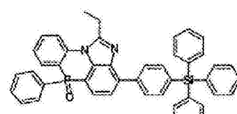
化学式 2-11-12
