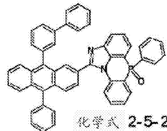
化学式 2-5-21
