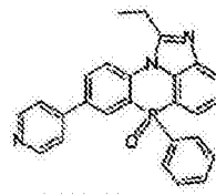
化学式 2-3-38
