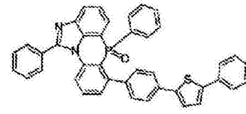
化学式 2-6-39
