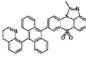
化学式 1-2-11
