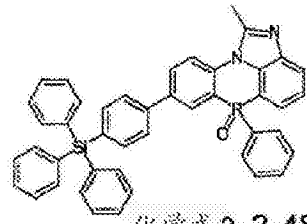
化学式 2-2-48
