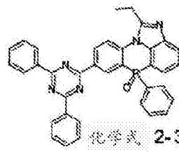
化学式 2-3-38
