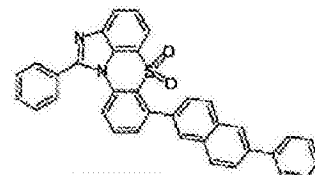
化学式 1-6-27
