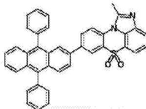
化学式 1-2-19
