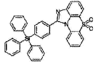
化学式 1-1-4
