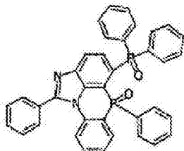
化学式 2-12-7
