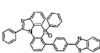
化学式 2-6-46
