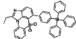
化学式 1-9-12
