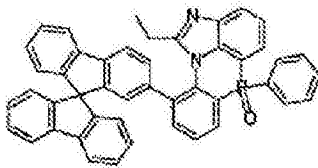
化学式 2-8-34
