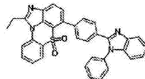
化学式 1-9-9
