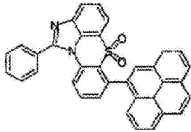
化学式 1-6-28
