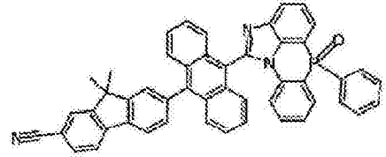
化学式 2-5-15
