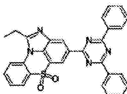
化学式 1-10-5
