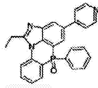
化学式 2-10-2
