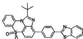
化学式 1-11-10
