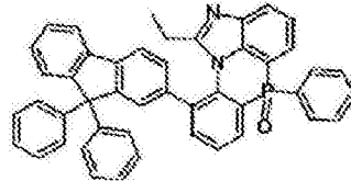
化学式 2-8-35
