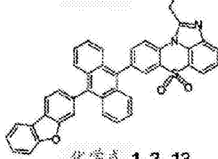
化学式 1-3-13
