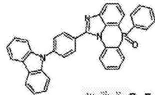
化学式 2-5-42
