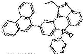
化学式 2-7-31
