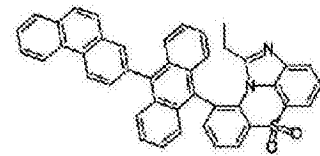
化学式 1-8-9
