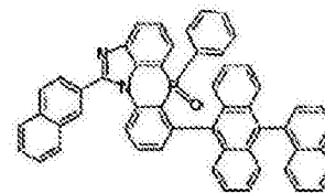
化学式 2-6-3
