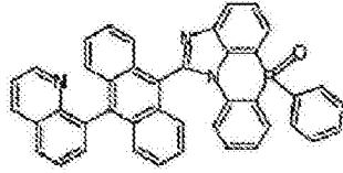
化学式 2-5-11
