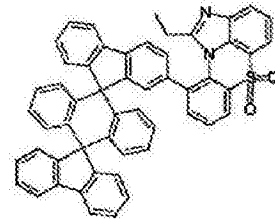
化学式 1-8-36
