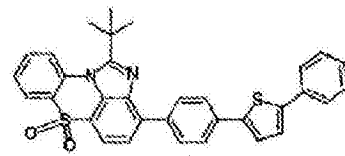
化学式 1-11-3
