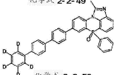
化学式 2-2-52
