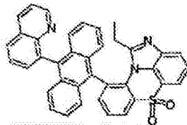
化学式 1-8-11
