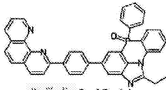
化学式 2-10-11
