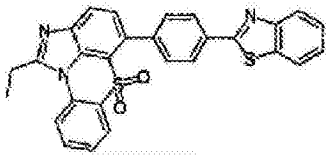
化学式 1-9-10
