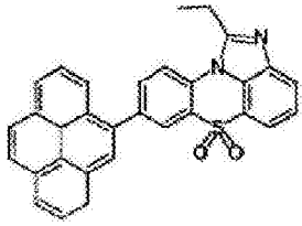
化学式 1-3-28
