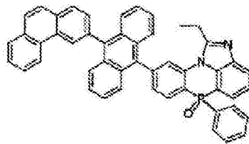
化学式 2-7-8
