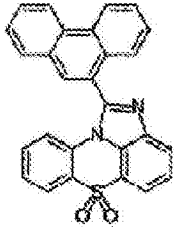
化学式 1-1-5
