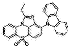
化学式 1-11-14
