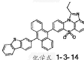
化学式 1-3-14
