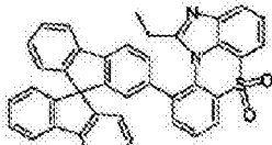
化学式 1-8-34
