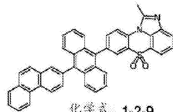
化学式 1-2-9
