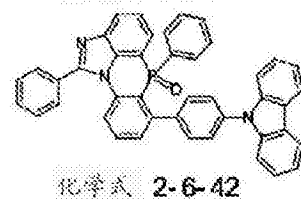
化学式 2-6-39
