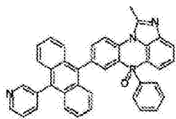
化学式 2-2-10
