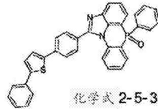
化学式 2-5-36
