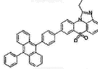
化学式 1-3-17
