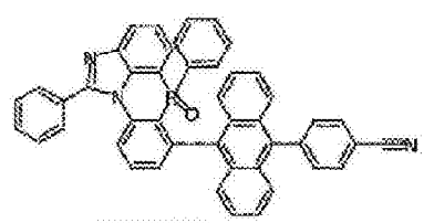
化学式 2-6-12
