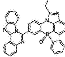
化学式 2-3-53
