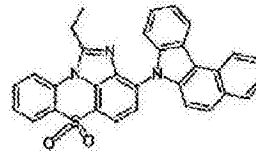
化学式 1-11-15
