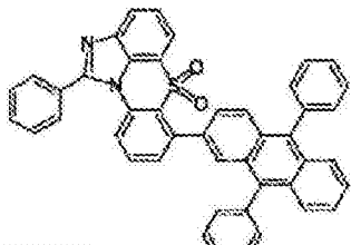
化学式 1-6-19
