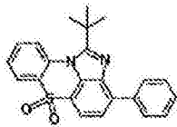
化学式 1-11-1
