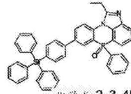
化学式 2-3-48
