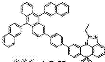
化学式 1-7-25
