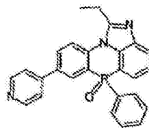
化学式 2-3-38
