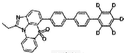
化学式 1-9-16
