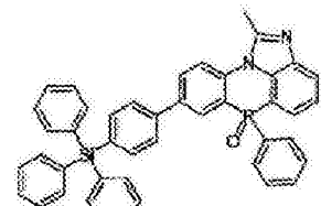
化学式 2-2-48
