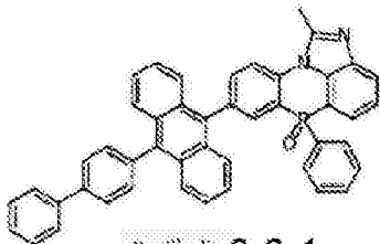
化学式 2-2-4
