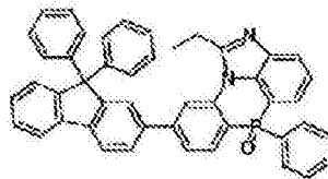
化学式 2-7-35
