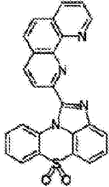
化学式 1-1-6
