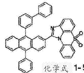
化学式 1-5-21
