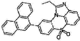
化学式 1-7-31
