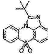
化学式 1-1-3
