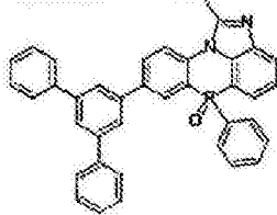
化学式 2-3-40
