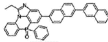
化学式 12-10-8
