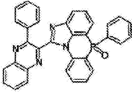
化学式 2-5-49
