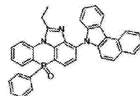
化学式 2-11-15
