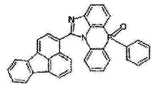
化学式 2-5-30
