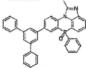
化学式 2-2-40
