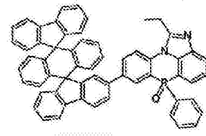
化学式 2-3-36
