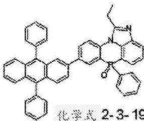
化学式 2-3-16
