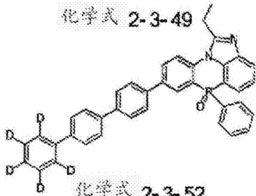
化学式 2-3-52
