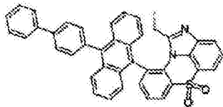
化学式 1-8-4
