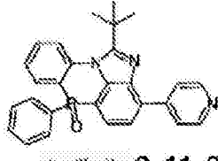
化学式 2-11-2
