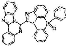
化学式 2-5-53
