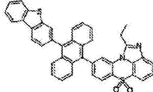
化学式 1-7-14
