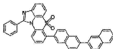
化学式 1-6-44
