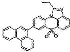
化学式 1-3-31
