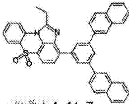
化学式 1-11-7
