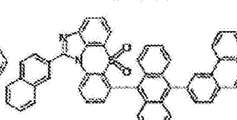
化学式 1-6-8
