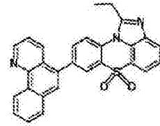
化学式 1-3-33
