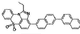
化学式 1-11-8
