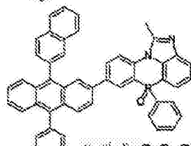
化学式 2-2-23
