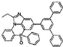
化学式 2-10-4
