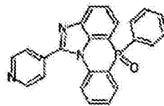
化学式 2-5-38
