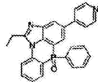
化学式 2-10-2
