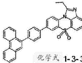
化学式 1-3-29
