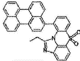
化学式 1-8-29
