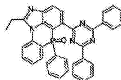
化学式 2-9-5
