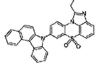
化学式 1-3-51
