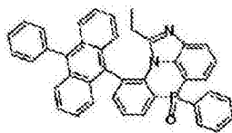
化学式 2-8-1
