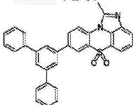
化学式 1-2-40
