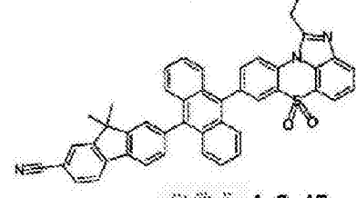
化学式 1-3-15
