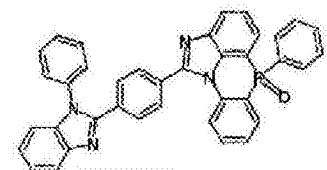
化学式 2-5-45
