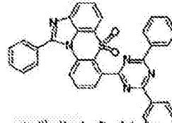
化学式 1-6-41
