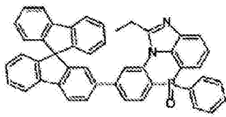
化学式 2-7-34
