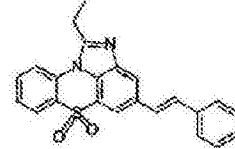
化学式 1-10-15
