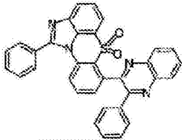
化学式 1-6-49
