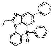
化学式 2-10-1
