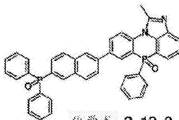
化学式 2-12-2
