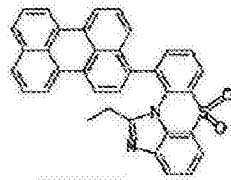
化学式 1-8-29
