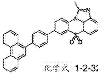
化学式 1-2-29
