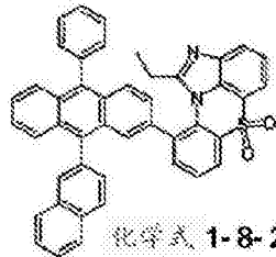
化学式 1-8-20
