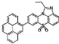
化学式 1-3-28
