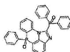
化学式 2-12-5
