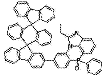
化学式 2-7-36
