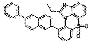
化学式 1-8-27
