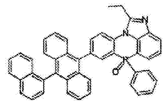
化学式 2-3-3
