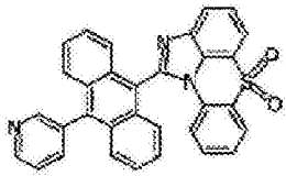
化学式 1-5-10
