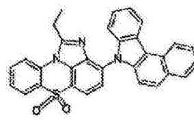
化学式 1-11-15
