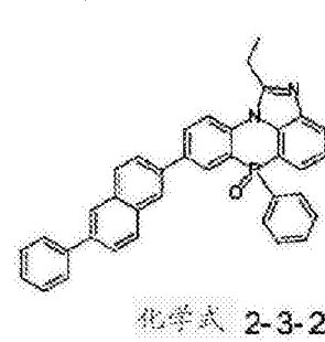
化学式 2-3-24
