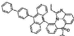
化学式 2-8-4
