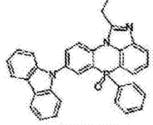
化学式 2-3-50
