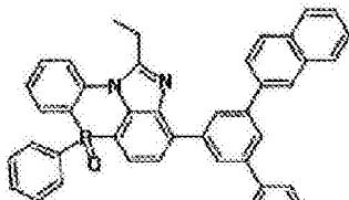
化学式 2-11-7
