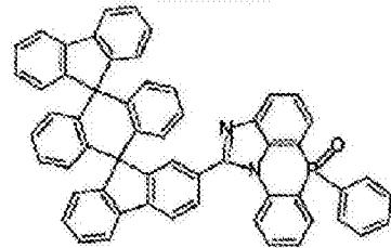
化学式 2-5-36
