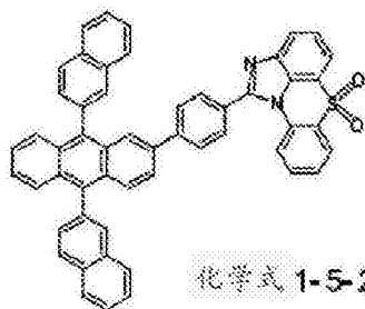
化学式 1-5-22
