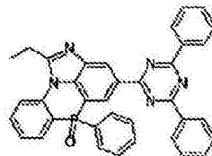
化学式 2-10-5
