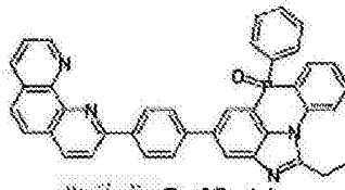
化学式 2-10-11
