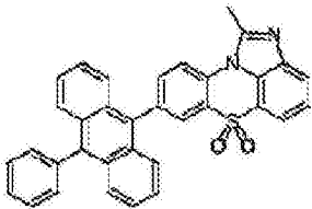
化学式 1-2-1
