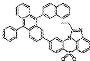
化学式 1-7-23
