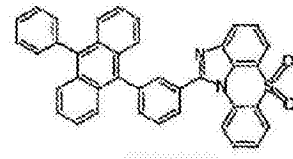
化学式 1-5-18
