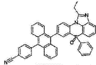
化学式 2-3-12
