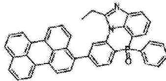
化学式 2-7-29
