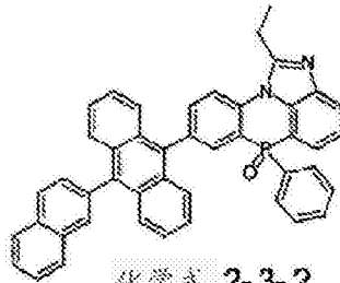
化学式 2-3-2
