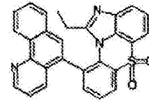
化学式 1-8-33
