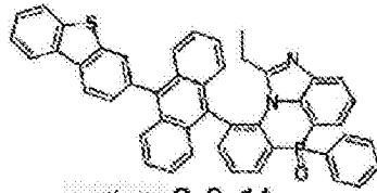
化学式 2-8-14
