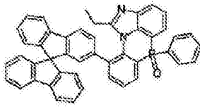
化学式 2-8-34
