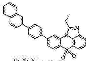
化学式 1-7-26
