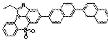
化学式 1-10-8
