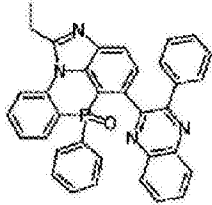
化学式 2-9-13
