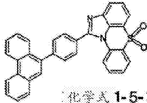
化学式 1-5-29
