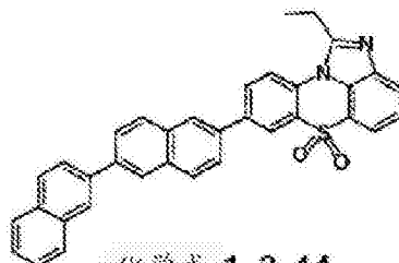
化学式 1-3-44
