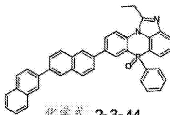
化学式 2-3-44
