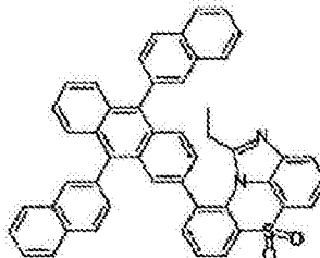
化学式 1-8-20
