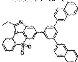
化学式 1-10-7
