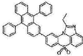
化学式 1-7-19
