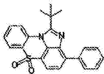
化学式 1-11-1
