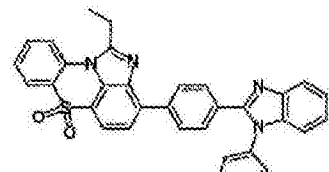
化学式 1-11-9
