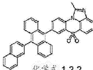
化学式 1-2-2
