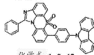
化学式 1-6-42
