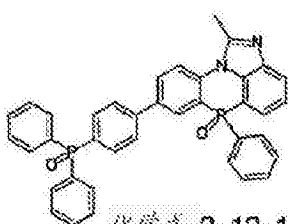
化学式 2-12-1
