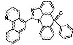
化学式 2-5-33
