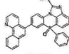
化学式 2-3-33
