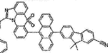
化学式 1-6-15
