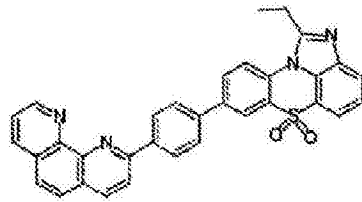
化学式 1-3-47
