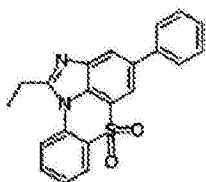
化学式 1-10-1
