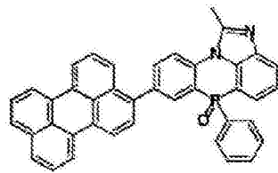
化学式 2-2-29
