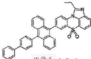
化学式 1-3-4
