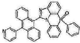
化学式 2-5-10
