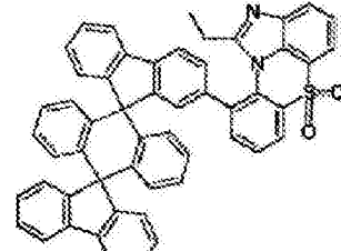
化学式 1-8-36
