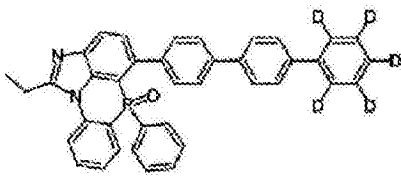
化学式 2-9-16
