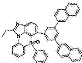
化学式 2-9-7
