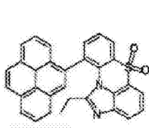
化学式 1-8-28
