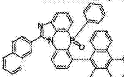
化学式 2-6-7
