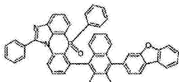
化学式 2-6-13
