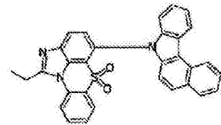
化学式 1-9-15
