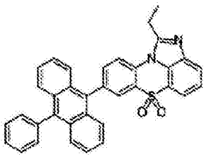
化学式 1-3-1
