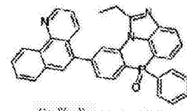
化学式 2-7-33
