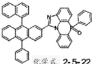
化学式 2-5-22
