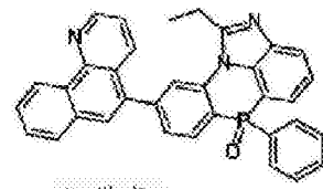
化学式 2-7-33
