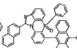
化学式 2-6-8
