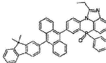
化学式 2-3-5
