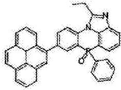
化学式 2-3-28
