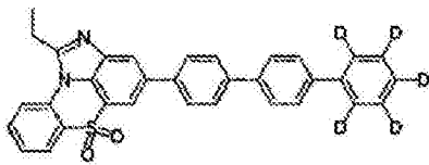
化学式 1-10-16
