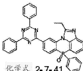
化学式 2-7-38
