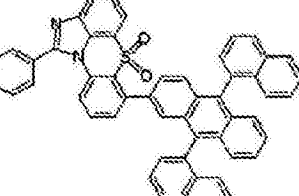
化学式 1-6-21
