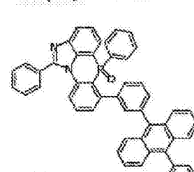
化学式 2-6-18
