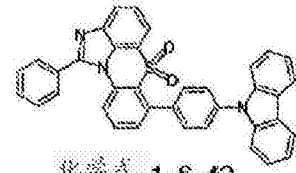
化学式 1-6-42
