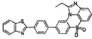
化学式 1-7-46
