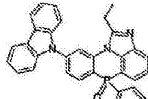
化学式 2-7-50
