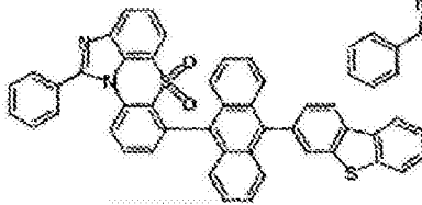
化学式 1-6-14
