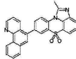
化学式 1-2-33
