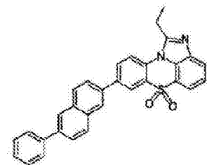
化学式 1-3-27
