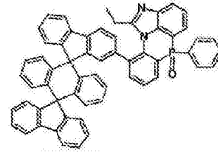
化学式 2-8-36
