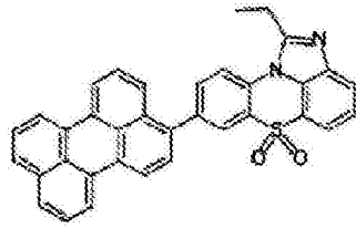
化学式 1-3-29
