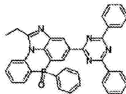
化学式 2-10-5
