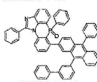
化学式 2-6-24
