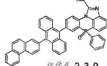
化学式 2-3-9
