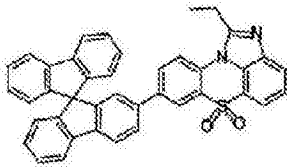
化学式 1-3-34
