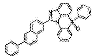
化学式 2-5-27
