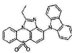
化学式 1-11-14
