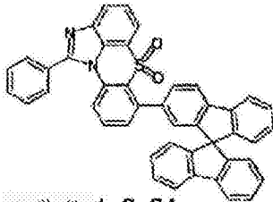
化学式 1-6-34
