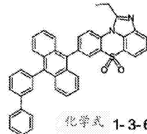
化学式 1-3-3
