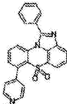
化学式 1-6-38
