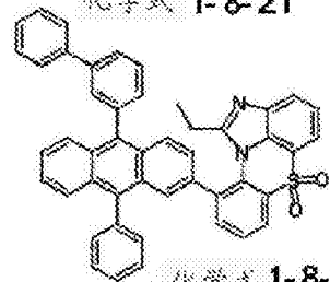
化学式 1-8-24
