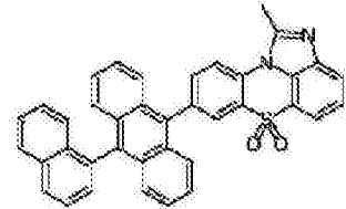
化学式 1-2-3
