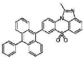
化学式 1-2-1
