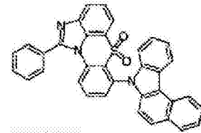
化学式 1-6-51
