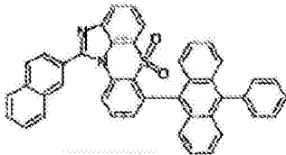
化学式 1-6-1
