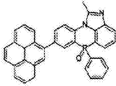
化学式 2-2-28
