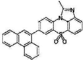
化学式 1-2-31
