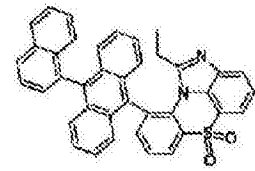
化学式 1-8-3
