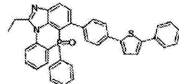
化学式 2-9-3
