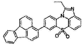
化学式 1-3-30
