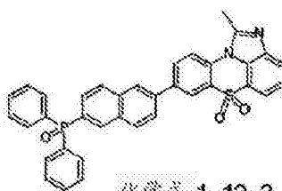
化学式 1-12-2
