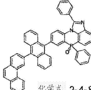
化学式 2-4-5
