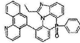
化学式 2-8-33
