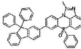
化学式 2-2-35
