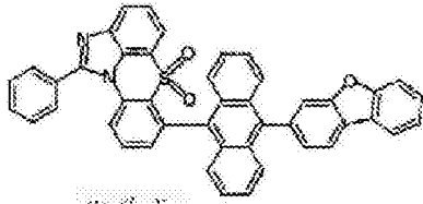
化学式 1-6-13
