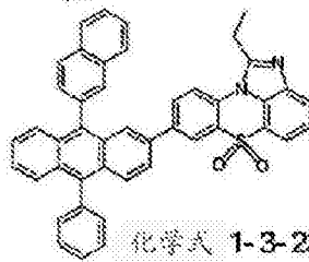
化学式 1-3-20
