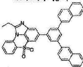
化学式 1-10-7
