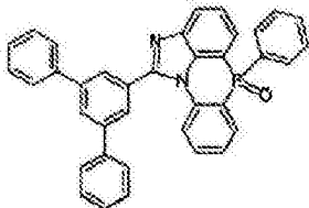
化学式 2-5-40
