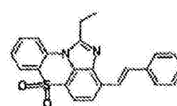
化学式 1-11-18
