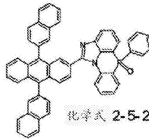
化学式 2-5-17
