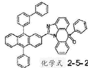
化学式 2-5-21
