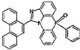
化学式 2-5-31
