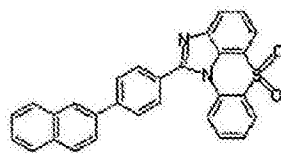
化学式 1-5-26
