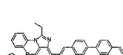
化学式 2-11-8
