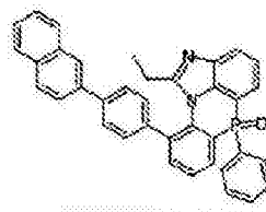
化学式 2-8-26
