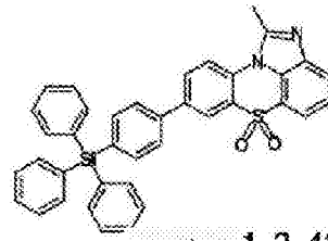
化学式 1-2-48
