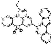
化学式 1-10-17
