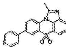
化学式 1-2-38
