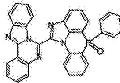
化学式 2-5-53
