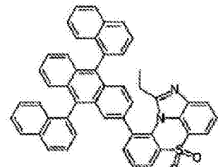
化学式 1-8-21
