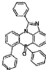
化学式 2-6-38
