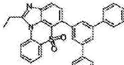
化学式 1-9-4
