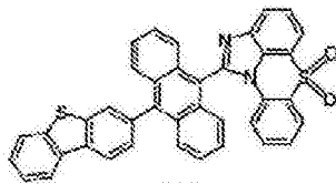
化学式 1-5-14
