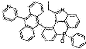
化学式 2-8-10
