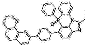
化学式 2-9-11
