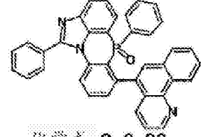
化学式 2-6-33
