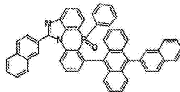
化学式 2-6-2
