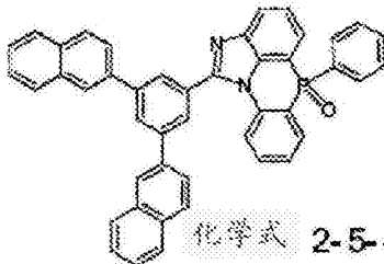
化学式 2-5-40
