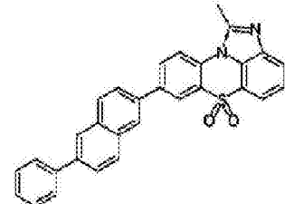
化学式 1-2-27
