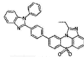
化学式 1-7-45
