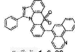
化学式 1-6-33
