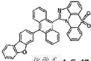
化学式 1-5-13
