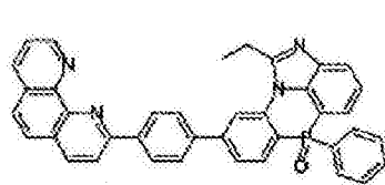
化学式 2-7-47
