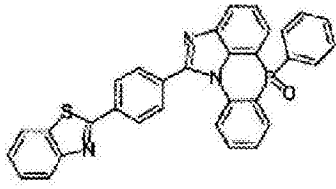
化学式 2-5-46
