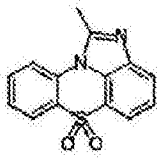
化学式 1-1-1
