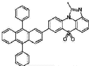
化学式 1-2-19
