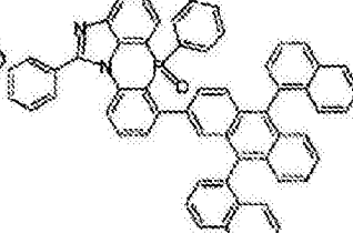
化学式 2-6-21
