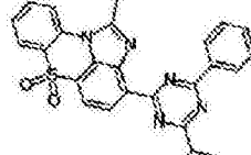
化学式 1-11-5
