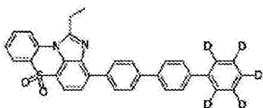
化学式 1-11-16
