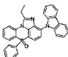
化学式 2-11-14
