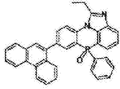
化学式 2-3-31
