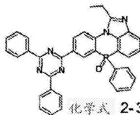
化学式 2-3-38
