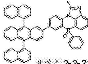
化学式 2-2-21
