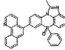
化学式 2-2-33
