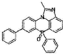
化学式 2-2-37
