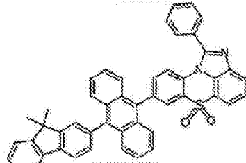
化学式 1-4-5
