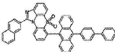
化学式 1-6-4
