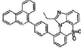
化学式 1-8-32
