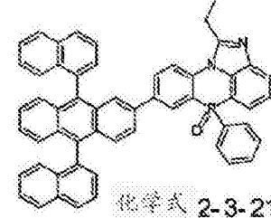
化学式 2-3-18
