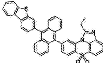
化学式 1-7-14
