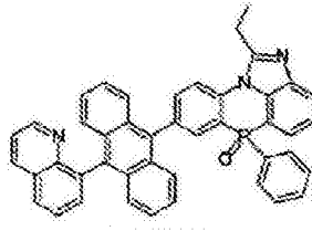
化学式 2-3-11
