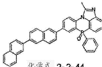
化学式 2-2-41
