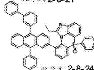
化学式 2-8-24
