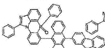
化学式 2-6-14
