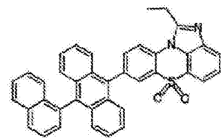
化学式 1-3-3
