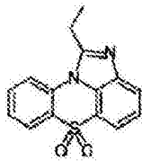
化学式 1-1-2
