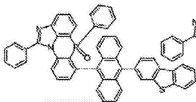
化学式 2-6-14
