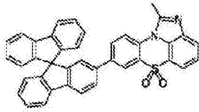
化学式 1-2-34
