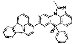
化学式 2-2-30
