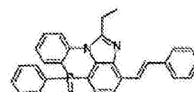
化学式 2-11-18
