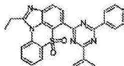
化学式 1-9-5
