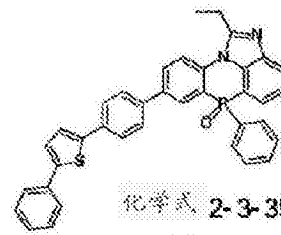
化学式 2-3-36
