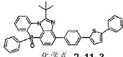
化学式 2-11-3
