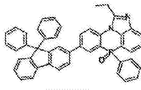
化学式 2-3-35
