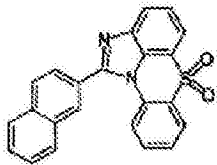
化学式 1-5-37
