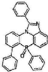
化学式 2-6-37
