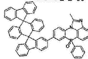
化学式 2-2-36
