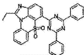
化学式 1-9-5
