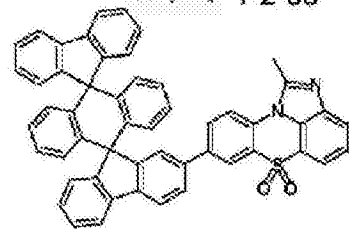
化学式 1-2-36
