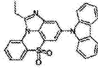
化学式 1-10-14
