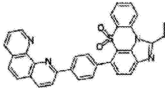
化学式 1-9-11
