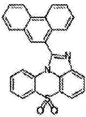
化学式 1-1-5
