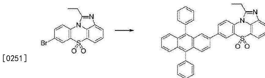
[化合物 2-B]
