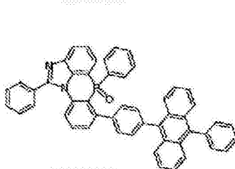
化学式 2-6-17
