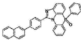
化学式 2-5-26
