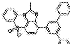
化学式 1-11-4
