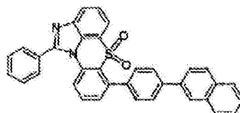
化学式 1-6-26
