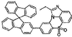
化学式 1-7-34
