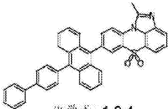
化学式 1-2-4
