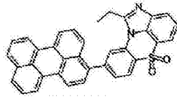
化学式 1-7-29
