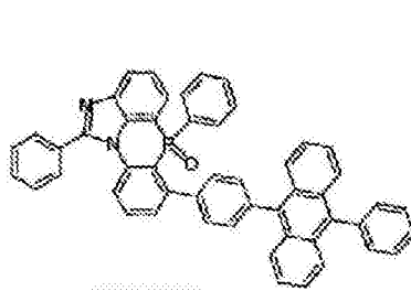
化学式 2-6-17
