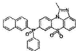
化学式 1-12-4
