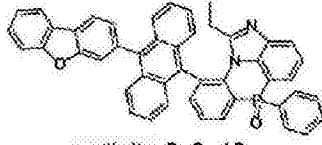
化学式 2-8-13
