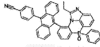
化学式 2-8-12
