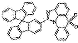
化学式 1-5-34
