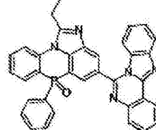
化学式 2-10-17
