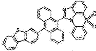
化学式 1-5-14
