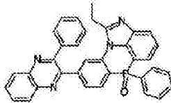
化学式 2-7-49
