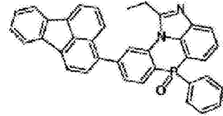
化学式 2-7-30
