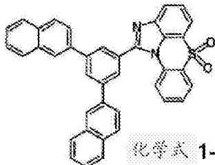
化学式 1-5-40
