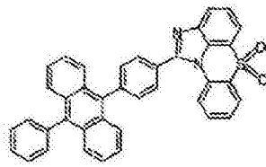
化学式 1-5-17
