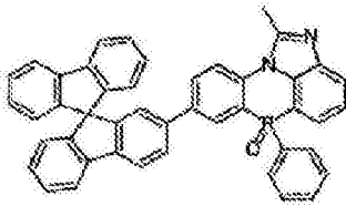
化学式 2-2-34
