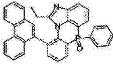
化学式 2-8-31
