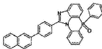
化学式 2-5-26
