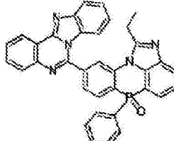
化学式 2-7-53
