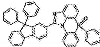
化学式 2-5-35
