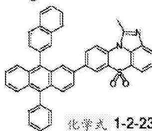
化学式 1-2-20
