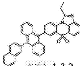
化学式 1-3-2
