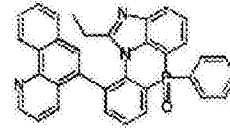
化学式 2-8-33
