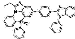
化学式 2-10-9
