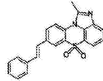
化学式 1-2-54
