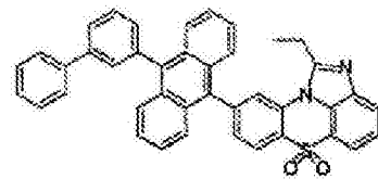
化学式 1-7-6
