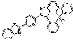
化学式 2-5-46
