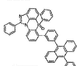
化学式 2-6-18
