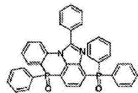
化学式 2-12-6
