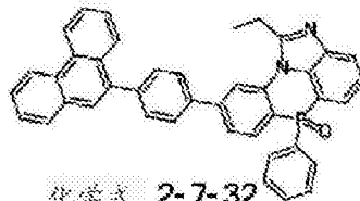
化学式 2-7-32
