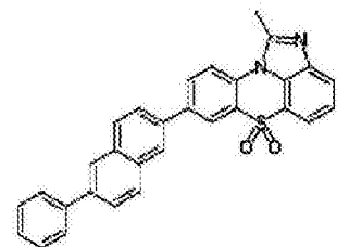
化学式 1-2-27
