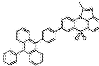
化学式 1-2-17
