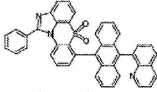
化学式 1-6-11
