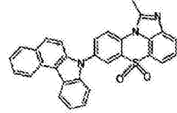
化学式 1-2-51
