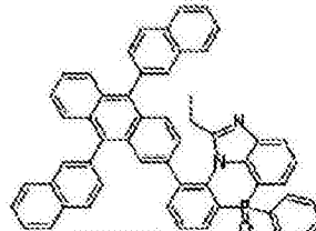
化学式 2-8-20
