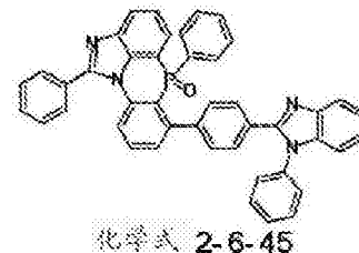
化学式 2-6-42
