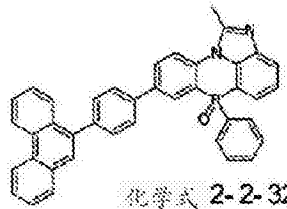
化学式 2-2-29
