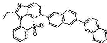
化学式 1-9-8
