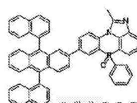
化学式 2-2-21
