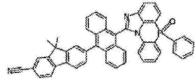
化学式 2-5-15
