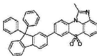
化学式 1-2-35
