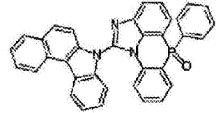
化学式 2-5-51
