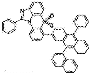
化学式 1-6-22
