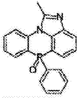
化学式 2-1-1
