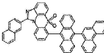
化学式 1-6-7
