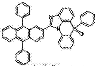
化学式 2-5-19
