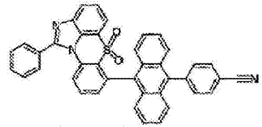
化学式 1-6-12
