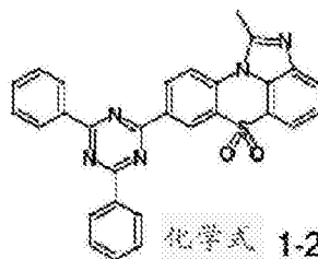
化学式 1-2-38
