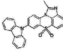
化学式 1-2-50
