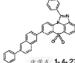
化学式 1-4-24
