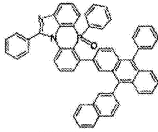
化学式 2-6-23
