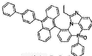
化学式 2-8-4
