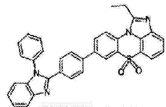
化学式 1-3-45
