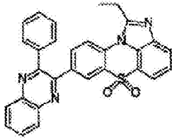
化学式 1-3-49
