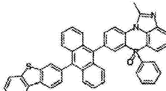
化学式 2-2-14
