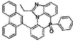
化学式 2-8-31
