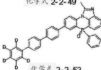
化学式 2-2-52
