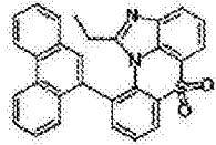
化学式 1-8-31
