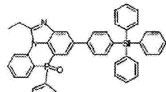
化学式 2-10-12
