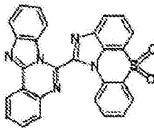
化学式 1-5-53
