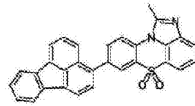
化学式 1-2-30
