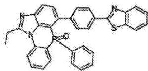
化学式 2-9-10
