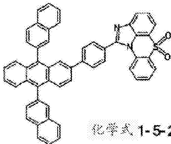
化学式 1-5-22
