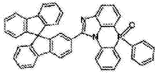
化学式 2-5-34
