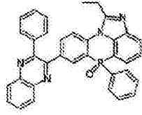
化学式 2-3-49
