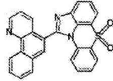
化学式 1-5-33
