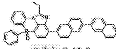
化学式 2-11-8
