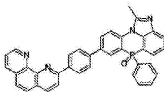
化学式 2-2-47
