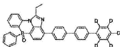
化学式 2-11-16
