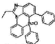
化学式 2-9-1
