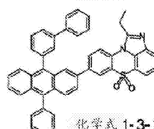
化学式 1-3-24
