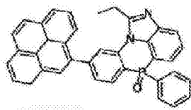
化学式 2-7-28
