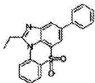
化学式 1-10-1
