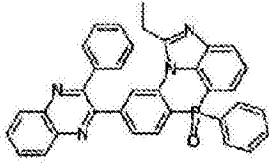
化学式 2-7-49
