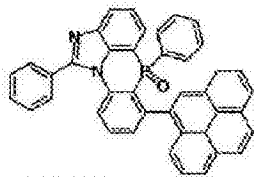
化学式 2-6-28
