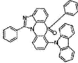
化学式 2-6-50
