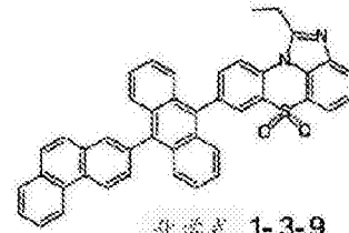
化学式 1-3-9
