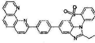
化学式 1-10-11
