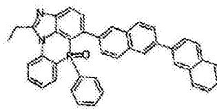
化学式 2-9-8
