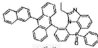
化学式 2-8-2
