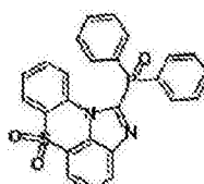
化学式 1-12-5
