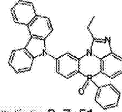
化学式 2-7-51
