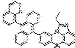
化学式 1-7-11
