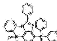
化学式 1-12-6
