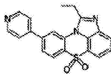
化学式 1-7-38
