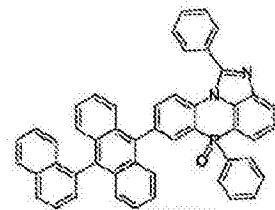
化学式 2-4-3
