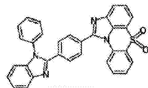
化学式 1-5-45
