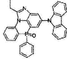
化学式 2-10-14
