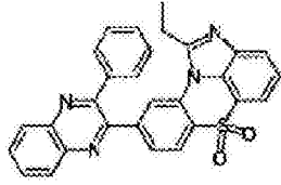
化学式 1-7-49
