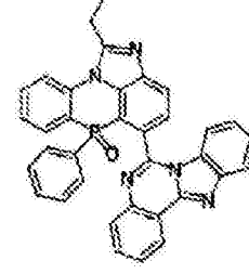
化学式 2-9-17
