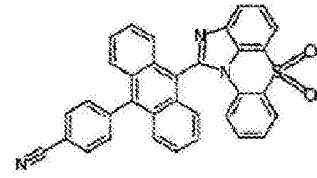
化学式 1-5-12
