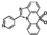
化学式 1-5-38
