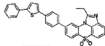
化学式 1-7-39
