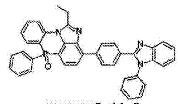
化学式 2-11-9
