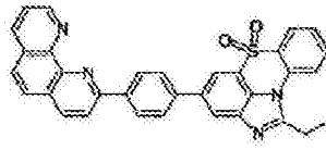
化学式 1-10-11
