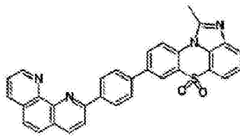
化学式 1-2-47
