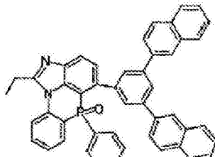
化学式 2-9-7
