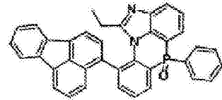
化学式 2-8-30
