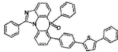
化学式 2-6-39
