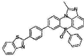
化学式 2-2-46
