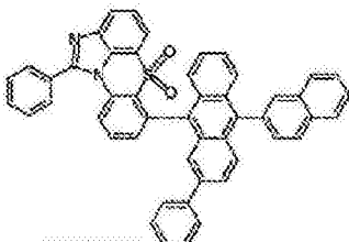
化学式 1-6-16
