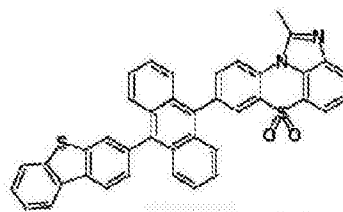
化学式 1-2-14
