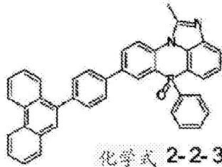
化学式 2-2-29
