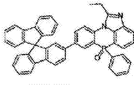
化学式 2-3-34
