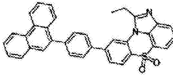
化学式 1-7-32
