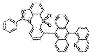
化学式 1-6-11
