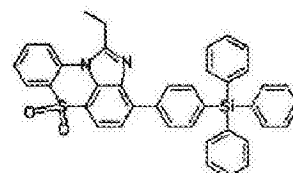
化学式 1-11-12
