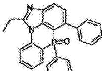
化学式 2-9-1
