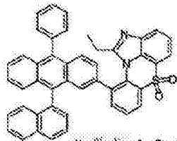
化学式 1-8-22
