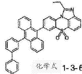
化学式 1-3-3
