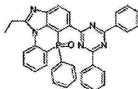
化学式 2-9-5
