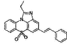
化学式 1-10-15
