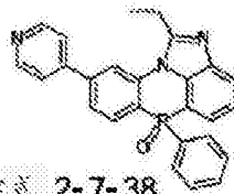
化学式 2-7-35
