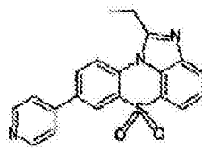
化学式 1-3-38
