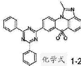
化学式 1-2-38
