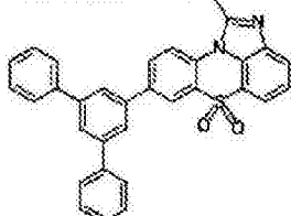
化学式 1-3-40
