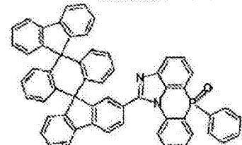
化学式 2-5-36
