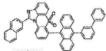
化学式 1-6-6
