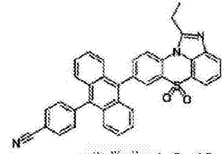
化学式 1-3-12
