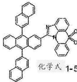
化学式 1-5-17
