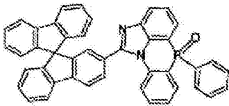
化学式 2-5-34
