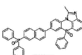
化学式 2-12-2
