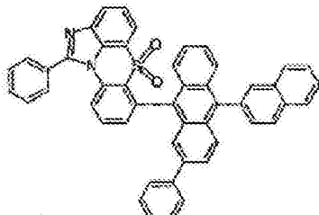
化学式 1-6-16
