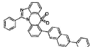
化学式 1-6-27
