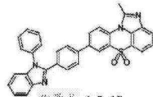
化学式 1-2-45
