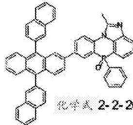
化学式 2-2-17
