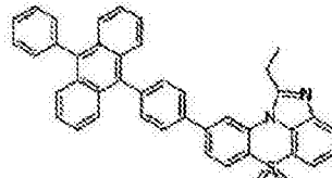
化学式 1-7-17
