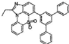
化学式 1-9-4
