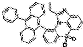
化学式 1-8-1
