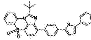
化学式 1-11-3
