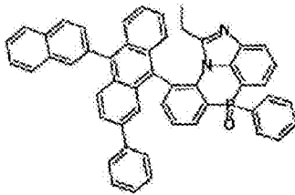
化学式 2-8-16
