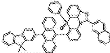
化学式 2-6-5
