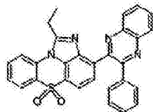
化学式 1-11-13
