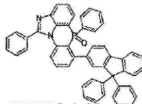
化学式 2-6-35
