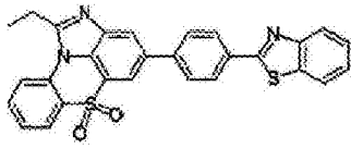
化学式 1-10-10
