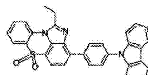
化学式 1-11-6
