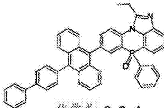
化学式 2-3-4
