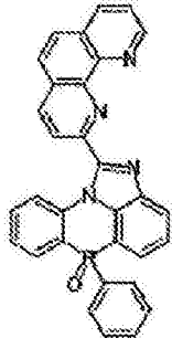
化学式 2-1-6
