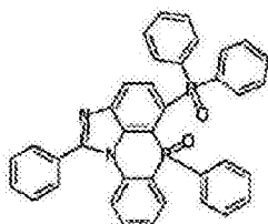
化学式 2-12-7
