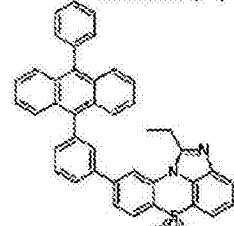
化学式 1-7-18
