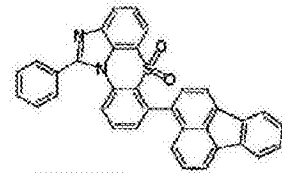
化学式 1-6-30
