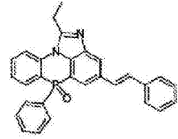
化学式 2-10-18
