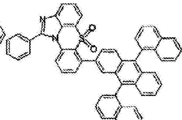
化学式 1-6-21
