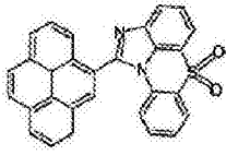
化学式 1-5-28
