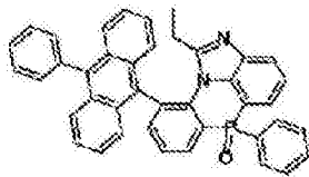
化学式 2-8-1
