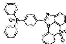
化学式 1-12-3
