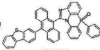
化学式 2-5-14
