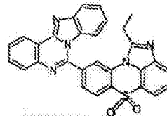
化学式 1-7-53
