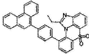
化学式 1-8-32
