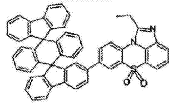
化学式 1-3-36
