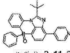
化学式 2-11-2
