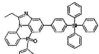
化学式 2-10-12
