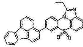
化学式 1-3-30
