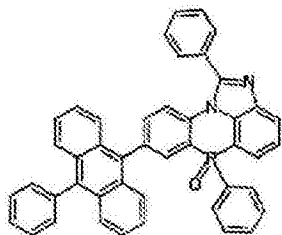
化学式 2-4-1
