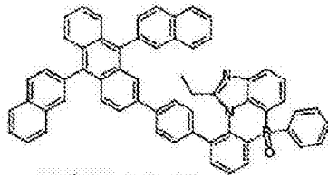
化学式 2-8-25
