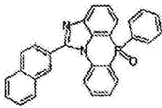
化学式 2-5-37
