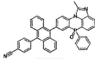
化学式 2-2-12
