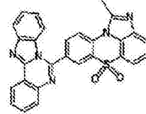
化学式 1-2-53
