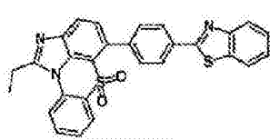
化学式 1-9-10
