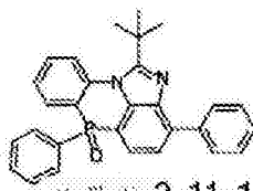
化学式 2-11-1
