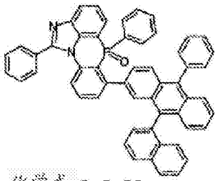
化学式 2-6-22
