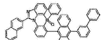
化学式 2-6-6
