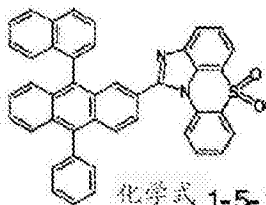
化学式 1-5-19
