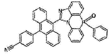
化学式 2-5-12
