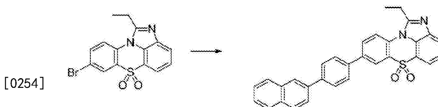
[化合物 2-B]
