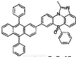
化学式 2-2-19
