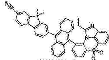
化学式 1-8-15
