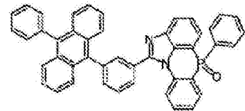
化学式 2-5-18
