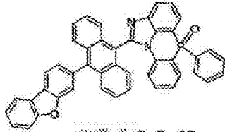
化学式 2-5-13
