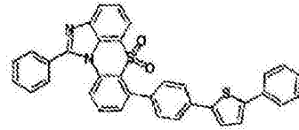
化学式 1-6-39
