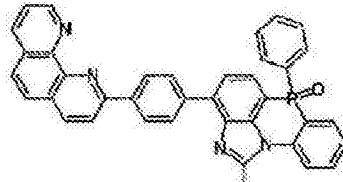
化学式 2-11-11
