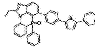
化学式 2-9-3
