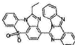
化学式 1-11-17
