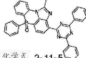
化学式 2-11-5
