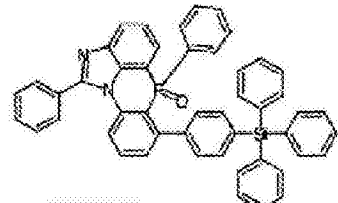
化学式 2-6-48
