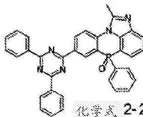
化学式 2-2-38
