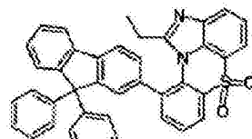
化学式 1-8-35
