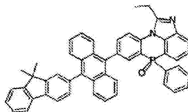
化学式 2-3-5
