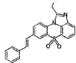
化学式 1-3-54
