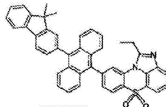
化学式 1-7-5
