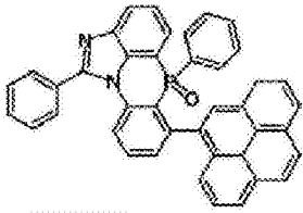
化学式 2-6-28
