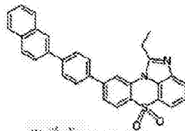
化学式 1-7-26
