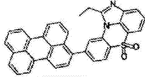
化学式 1-7-29
