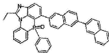
化学式 2-9-8
