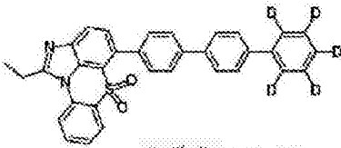
化学式 1-9-16
