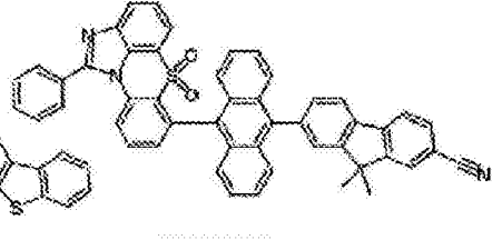
化学式 1-6-15
