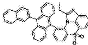
化学式 1-8-2
