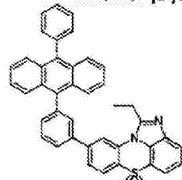
化学式 1-7-18
