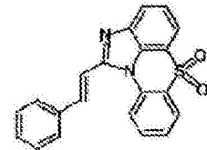
化学式 1-5-54
