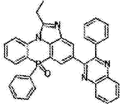
化学式 2-10-13
