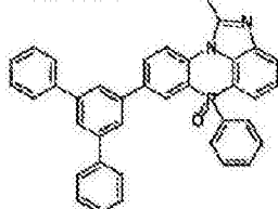
化学式 2-2-40
