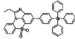
化学式 1-10-12
