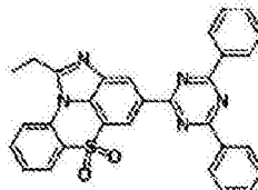
化学式 1-10-5
