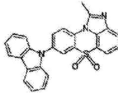
化学式 1-2-50
