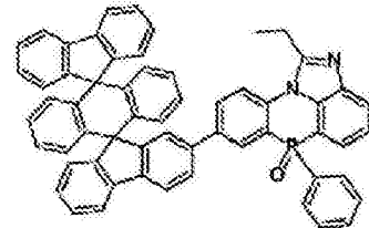
化学式 2-3-36
