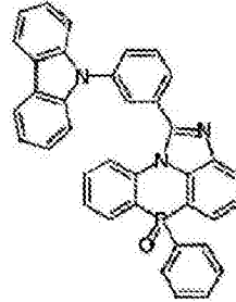
化学式 2-1-7
