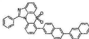
化学式 1-6-44
