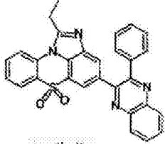
化学式 1-10-13
