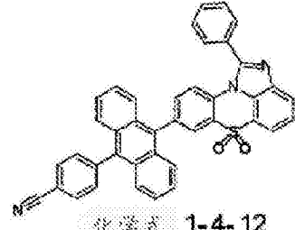
化学式 1-4-12
