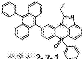
化学式 2-7-1
