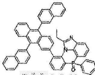
化学式 2-8-20
