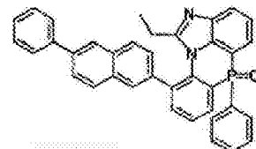
化学式 2-8-27
