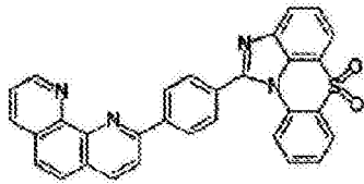
化学式 1-5-47
