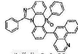
化学式 2-6-33
