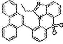
化学式 1-8-31
