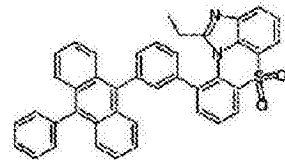
化学式 1-8-18
