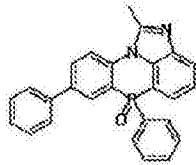
化学式 2-2-37
