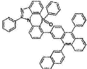
化学式 2-6-23
