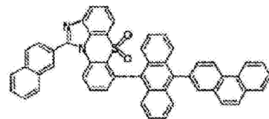
化学式 1-6-9
