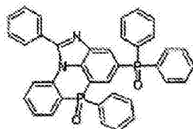
化学式 2-12-8
