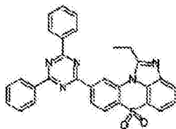
化学式 1-7-41
