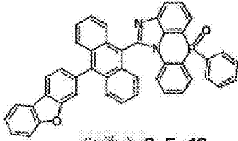
化学式 2-5-13
