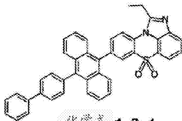
化学式 1-3-4
