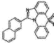
化学式 1-5-37
