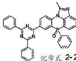
化学式 2-2-38
