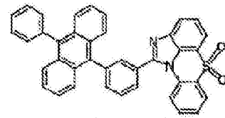
化学式 1-5-18
