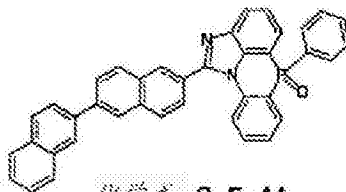
化学式 2-5-44
