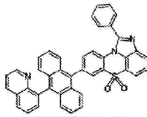
化学式 1-4-11
