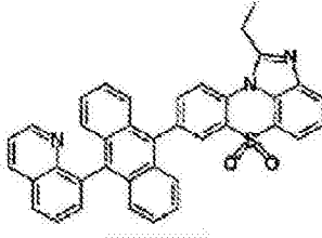
化学式 1-3-11
