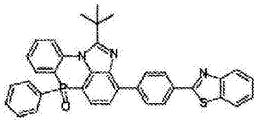
化学式 2-11-10
