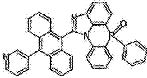
化学式 2-5-10
