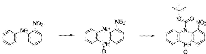
[化合物 2-1-A]
