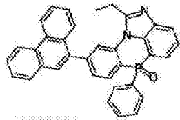
化学式 2-7-31
