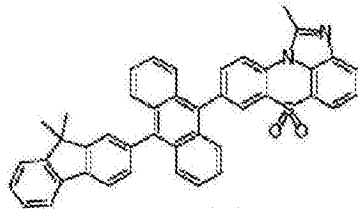
化学式 1-2-5
