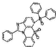
化学式 1-12-7
