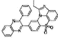
化学式 1-7-49
