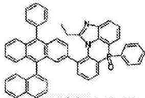
化学式 2-8-22
