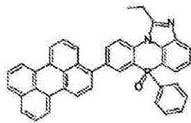
化学式 2-3-29
