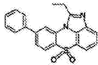
化学式 1-7-37
