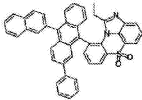
化学式 1-8-16
