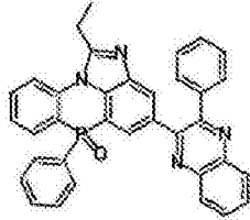
化学式 2-10-13
