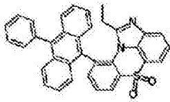
化学式 1-8-1
