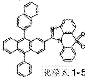
化学式 1-5-20
