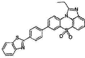
化学式 1-3-46
