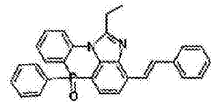
化学式 2-11-18
