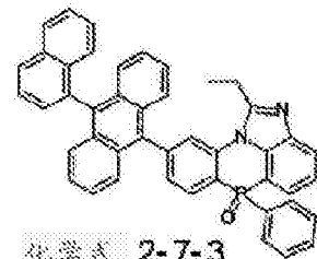
化学式 2-7-3
