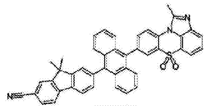
化学式 1-2-15
