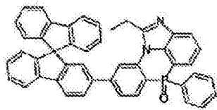
化学式 2-7-34
