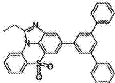
化学式 1-10-4
