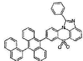
化学式 1-4-3
