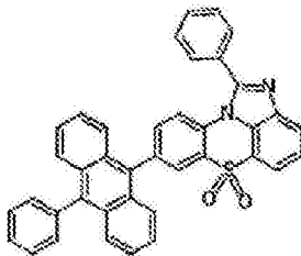
化学式 1-4-1
