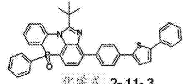
化学式 2-11-3
