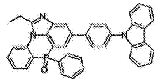
化学式 2-10-6
