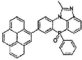
化学式 2-2-28
