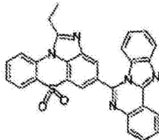
化学式 1-10-17
