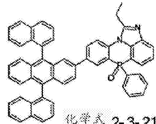
化学式 2-3-21
