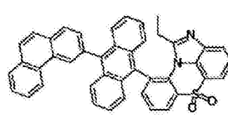
化学式 1-8-8
