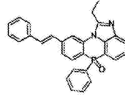
化学式 2-7-54
