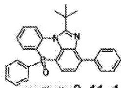
化学式 2-11-1
