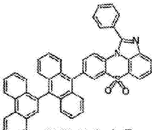
化学式 1-4-7
