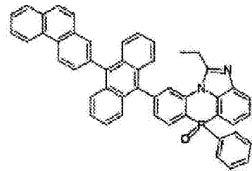
化学式 2-7-9
