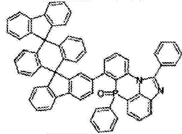
化学式 2-6-36
