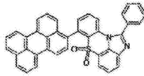
化学式 1-6-29
