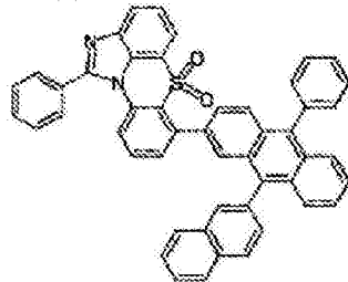
化学式 1-6-23
