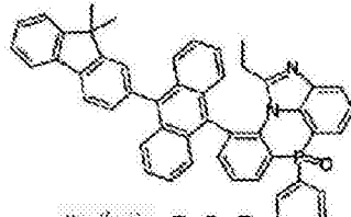
化学式 2-8-5
