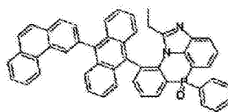
化学式 2-8-8
