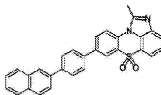
化学式 1-2-26
