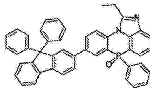
化学式 2-3-35
