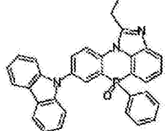
化学式 2-3-50
