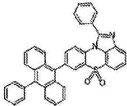
化学式 1-4-1
