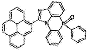
化学式 2-5-28
