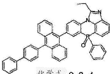
化学式 2-3-4
