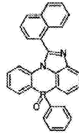
化学式 2-1-4
