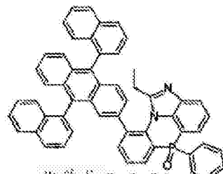
化学式 2-8-21
