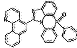
化学式 2-5-33
