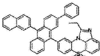
化学式 1-7-16
