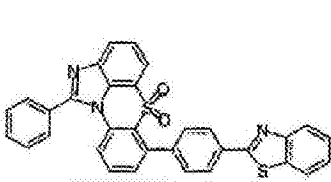
化学式 1-6-46
