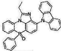
化学式 2-11-14
