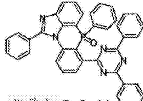
化学式 2-6-41
