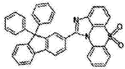
化学式 1-5-35
