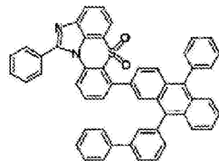
化学式 1-6-24
