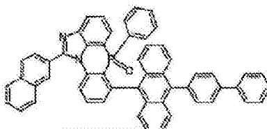
化学式 2-6-4
