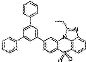
化学式 1-7-40
