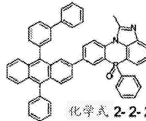
化学式 2-2-21
