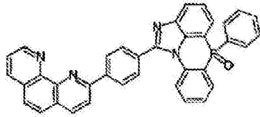
化学式 2-5-47
