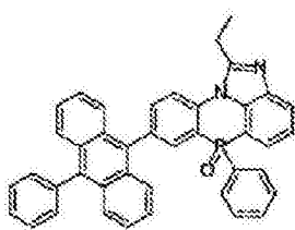
化学式 2-3-1
