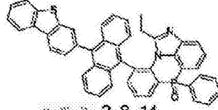
化学式 2-8-14
