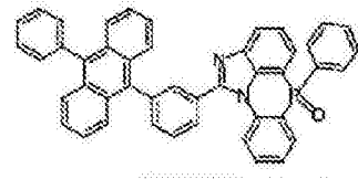
化学式 2-5-18
