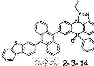
化学式 2-3-14
