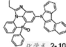
化学式 2-10-15
