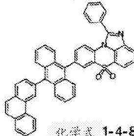
化学式 1-4-5
