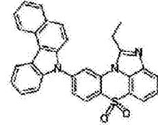
化学式 1-7-51
