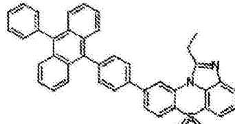
化学式 1-7-17
