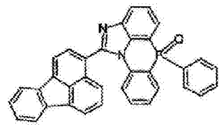
化学式 2-5-30
