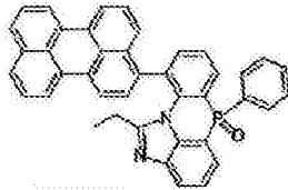
化学式 2-8-29
