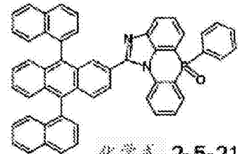
化学式 2-5-21
