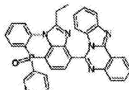
化学式 2-11-17
