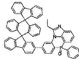
化学式 2-7-36
