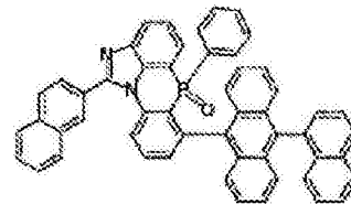
化学式 2-6-3
