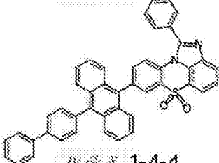
化学式 1-4-4
