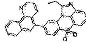
化学式 1-7-33
