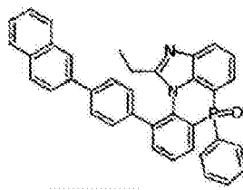
化学式 2-8-26
