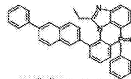
化学式 2-8-27
