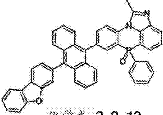
化学式 2-2-13
