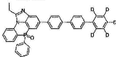
化学式 2-10-16
