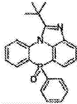
化学式 2-1-3
