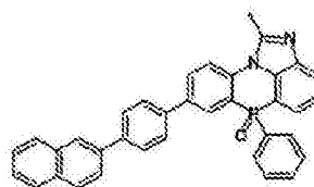
化学式 2-2-26
