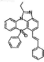
化学式 2-9-18
