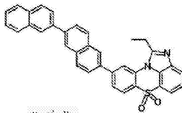
化学式 1-7-44
