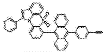
化学式 1-6-12
