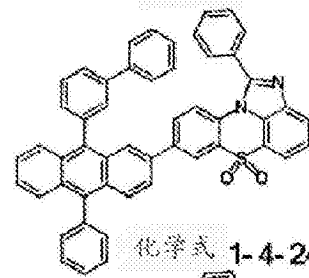
化学式 1-4-21
