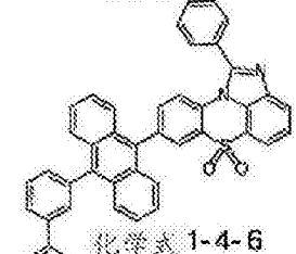
化学式 1-4-6
