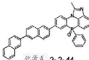
化学式 2-2-44
