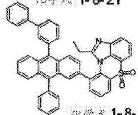
化学式 1-8-24
