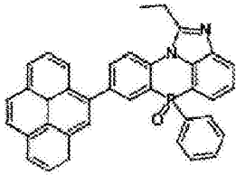
化学式 2-3-28
