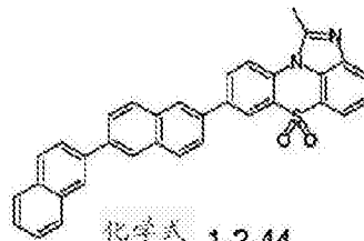
化学式 1-2-44
