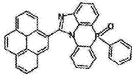
化学式 2-5-28
