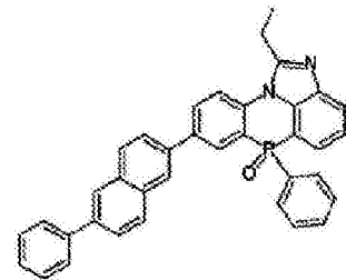
化学式 2-3-27
