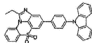
化学式 1-10-6
