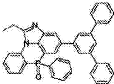
化学式 2-10-4
