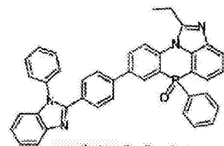
化学式 2-3-45
