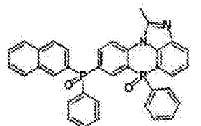
化学式 2-12-4
