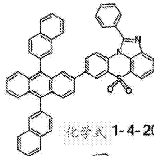
化学式 1-4-17
