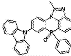
化学式 2-2-50
