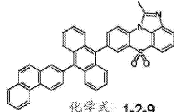
化学式 1-2-9
