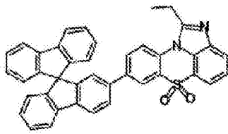
化学式 1-3-34
