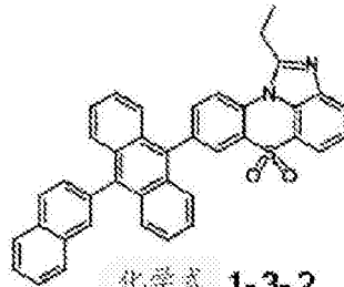
化学式 1-3-2
