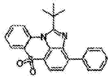
化学式 1-11-2
