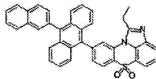
化学式 1-7-2
