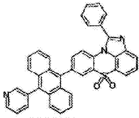
化学式 1-4-10
