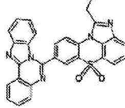
化学式 1-3-53
