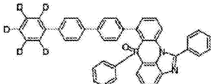
化学式 2-6-52
