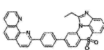
化学式 1-7-47
