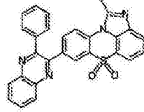
化学式 1-2-49
