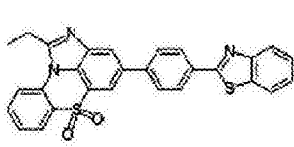
化学式 1-10-10
