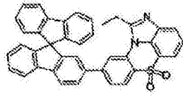
化学式 1-7-34
