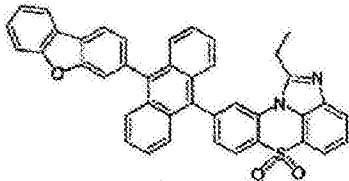
化学式 1-7-13
