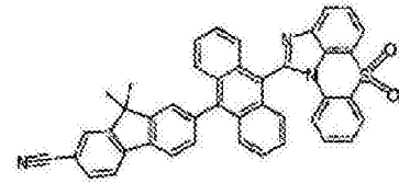
化学式 1-5-15
