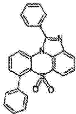
化学式 1-6-37
