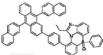
化学式 2-8-25
