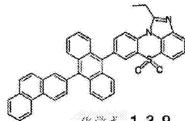
化学式 1-3-9
