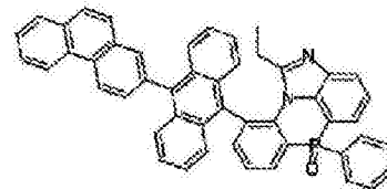
化学式 2-8-9
