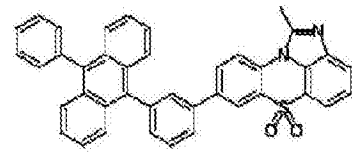
化学式 1-2-18
