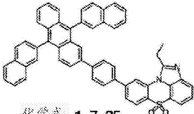
化学式 1-7-25
