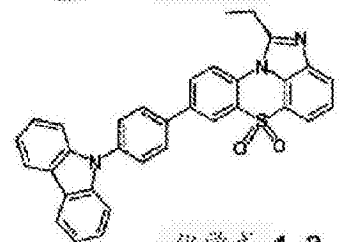
化学式 1-3-42
