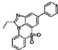
化学式 1-10-2
