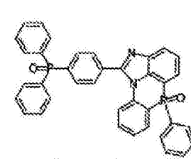
化学式 2-12-3
