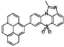
化学式 1-2-28
