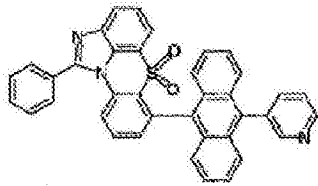
化学式 1-6-10
