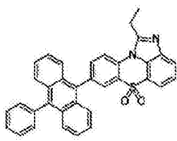
化学式 1-3-1
