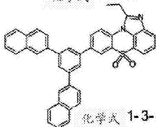
化学式 1-3-40
