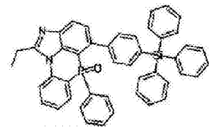
化学式 2-9-12
