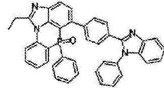
化学式 2-9-9
