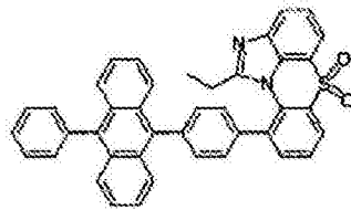
化学式 1-8-17
