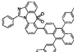
化学式 1-6-20
