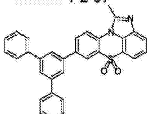
化学式 1-2-40
