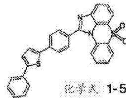
化学式 1-5-36
