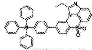
化学式 1-7-48
