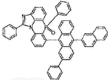
化学式 2-6-16
