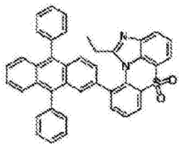
化学式 1-8-19
