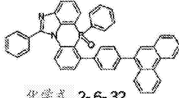
化学式 2-6-32
