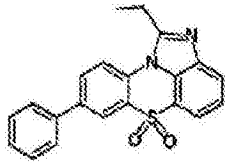
化学式 1-3-37
