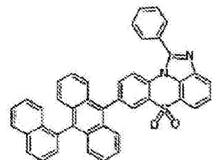
化学式 1-4-3
