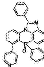
化学式 2-6-38
