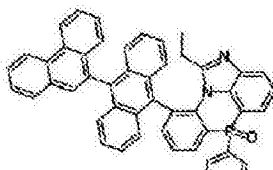
化学式 2-8-7
