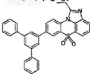
化学式 1-3-40
