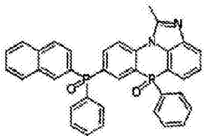
化学式 2-12-4
