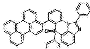
化学式 2-6-29
