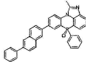
化学式 2-2-27
