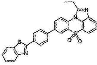
化学式 1-3-46
