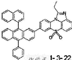
化学式 1-3-22
