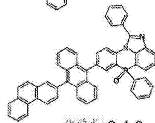
化学式 2-4-9
