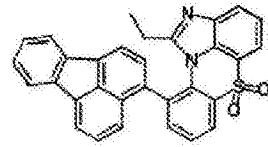
化学式 1-8-30
