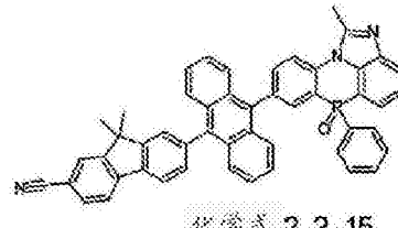
化学式 2-2-15
