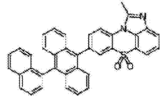
化学式 1-2-3
