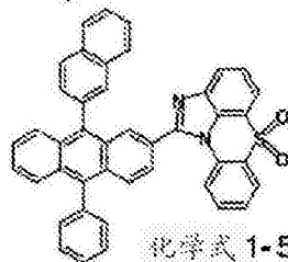
化学式 1-5-20
