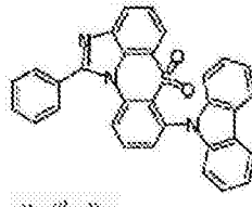
化学式 1-6-50
