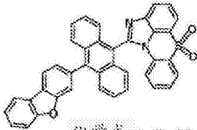
化学式 1-5-13
