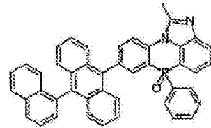
化学式 2-2-3
