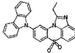
化学式 1-7-50
