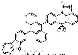
化学式 1-2-13
