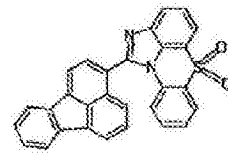
化学式 1-5-30
