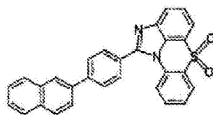
化学式 1-5-26
