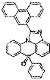
化学式 2-1-5
