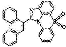
化学式 1-5-31
