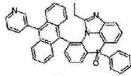
化学式 2-8-10
