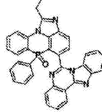
化学式 2-9-17
