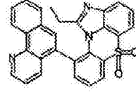
化学式 1-8-33
