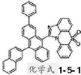
化学式 1-5-13
