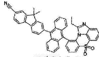
化学式 1-8-15
