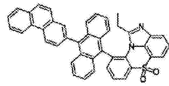
化学式 1-8-9
