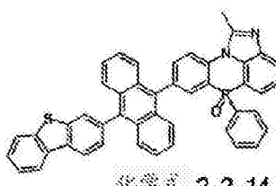
化学式 2-2-14
