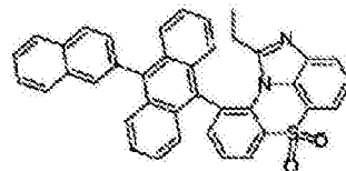
化学式 1-8-2
