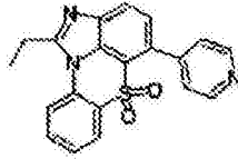
化学式 1-9-2
