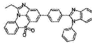
化学式 1-10-9
