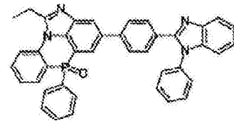
化学式 2-10-9
