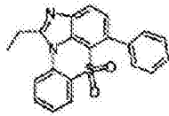
化学式 1-9-1
