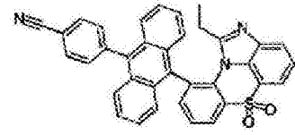
化学式 1-8-12
