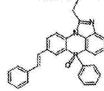
化学式 2-3-54
