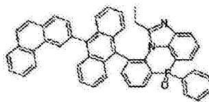
化学式 2-8-8
