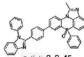
化学式 2-2-45
