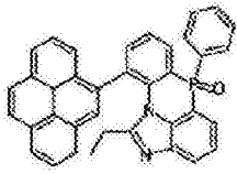
化学式 2-8-28
