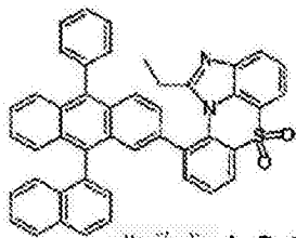
化学式 1-8-22
