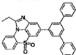
化学式 1-10-4
