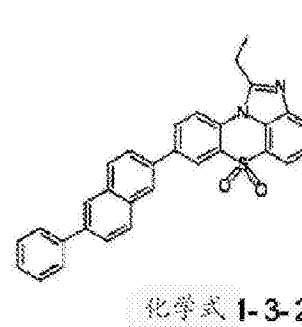
化学式 1-3-24
