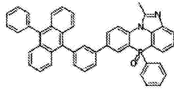
化学式 2-2-18
