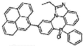
化学式 2-7-28
