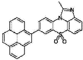
化学式 1-2-28
