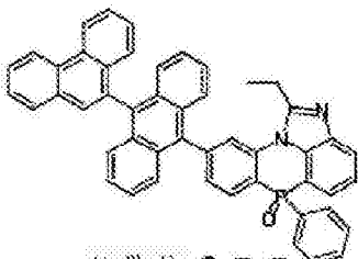
化学式 2-7-7
