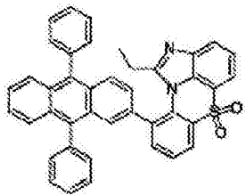
化学式 1-8-19
