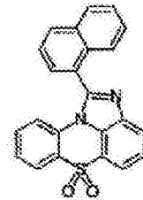
化学式 1-1-4
