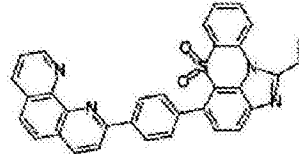
化学式 1-9-11
