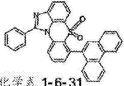
化学式 1-6-31
