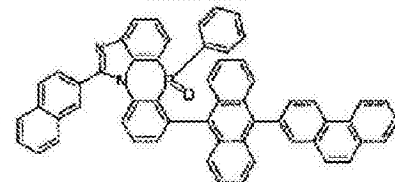
化学式 2-6-9
