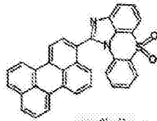
化学式 1-5-29
