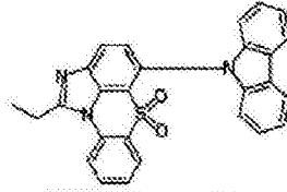
化学式 1-9-14
