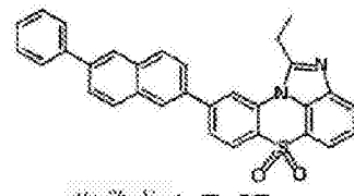
化学式 1-7-27
