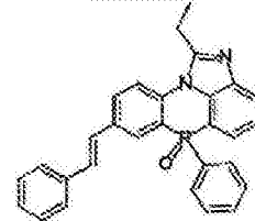
化学式 2-3-54
