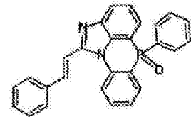
化学式 2-5-54
