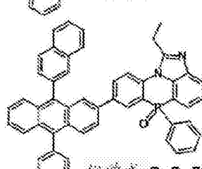
化学式 2-3-20
