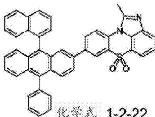
化学式 1-2-22
