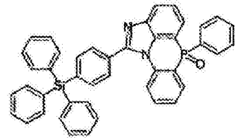
化学式 2-1-4
