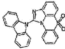
化学式 1-5-50
