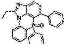
化学式 2-9-2
