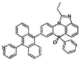
化学式 2-3-10
