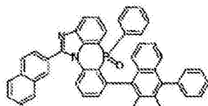
化学式 2-6-1
