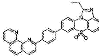
化学式 1-3-47
