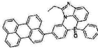
化学式 2-7-29
