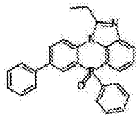
化学式 2-3-37
