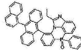
化学式 2-8-3
