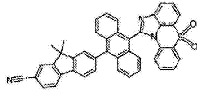
化学式 1-5-15
