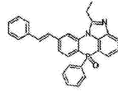
化学式 2-7-54
