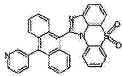
化学式 1-5-10
