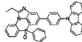
化学式 2-10-6
