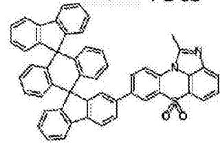
化学式 1-2-36
