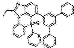
化学式 2-9-4
