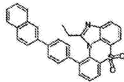
化学式 1-8-26
