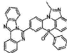
化学式 2-2-53
