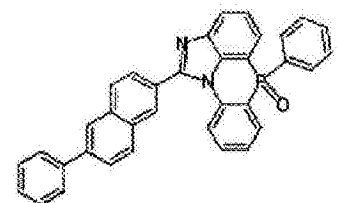
化学式 2-5-27
