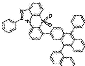
化学式 1-6-22
