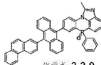
化学式 2-2-9
