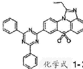
化学式 1-3-38
