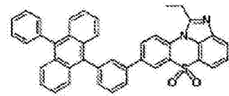
化学式 1-3-18
