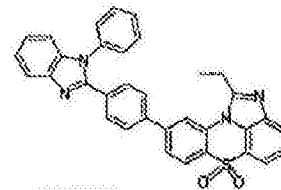
化学式 1-7-45
