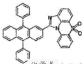
化学式 1-5-19
