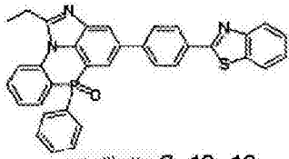
化学式 2-10-10
