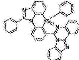
化学式 2-6-53
