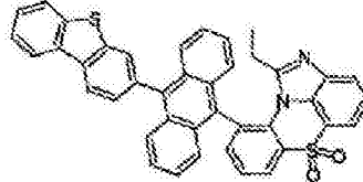
化学式 1-8-14
