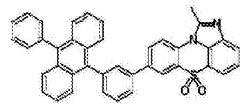
化学式 1-2-18
