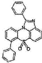
化学式 1-6-37
