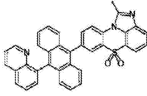
化学式 1-2-11
