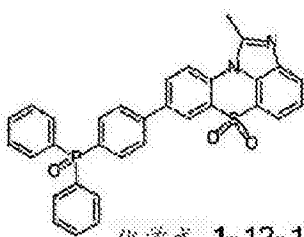
化学式 1-12-1
