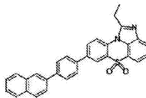
化学式 1-3-26
