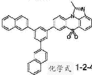
化学式 1-2-40
