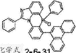
化学式 2-6-31
