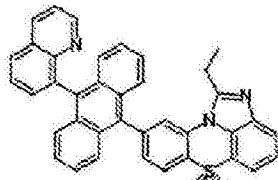
化学式 1-7-11
