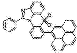
化学式 1-6-28
