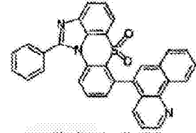
化学式 1-6-33
