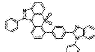
化学式 1-6-45
