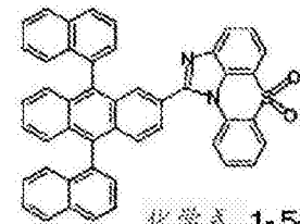
化学式 1-5-21
