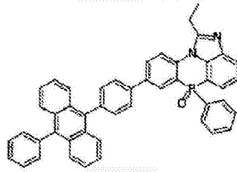
化学式 2-3-17
