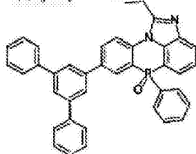
化学式 2-3-40
