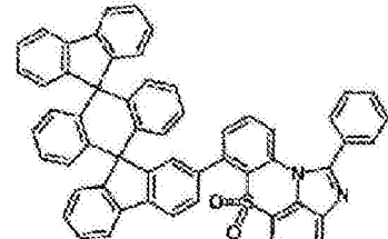
化学式 1-6-36
