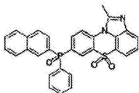
化学式 1-12-4
