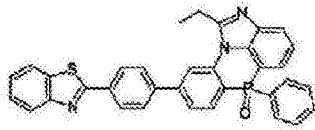
化学式 2-7-46
