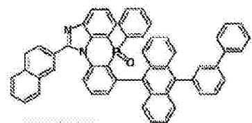
化学式 2-6-6
