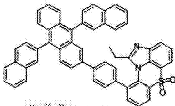
化学式 1-8-25
