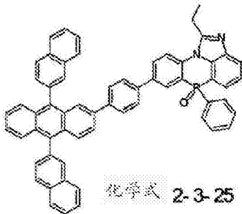
化学式 2-3-22
