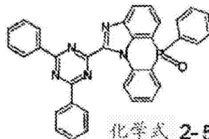
化学式 2-5-38
