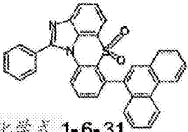
化学式 1-6-31
