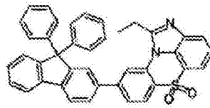
化学式 1-7-35
