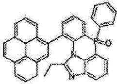
化学式 2-8-28
