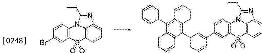
[化合物 2-B]
