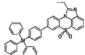
化学式 1-3-48
