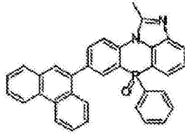
化学式 2-2-31
