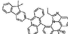
化学式 2-8-5
