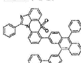
化学式 1-6-24
