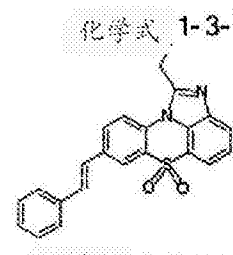
化学式 1-3-54
