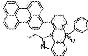
化学式 2-8-29
