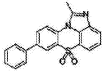
化学式 1-2-37
