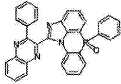
化学式 2-5-49
