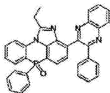
化学式 2-11-13
