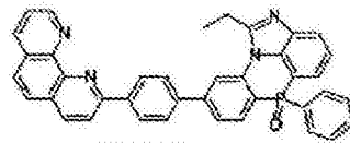
化学式 2-7-47
