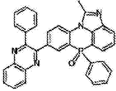
化学式 2-2-49
