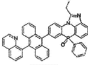
化学式 2-3-11
