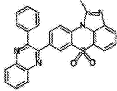
化学式 1-2-49
