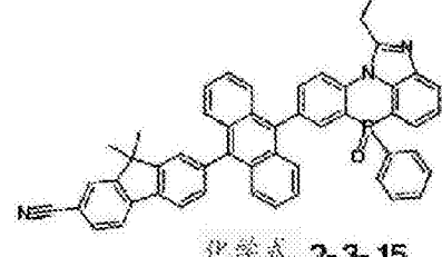
化学式 2-3-15
