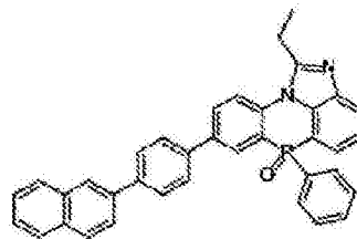
化学式 2-3-26
