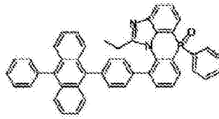
化学式 2-8-17
