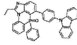
化学式 2-9-6
