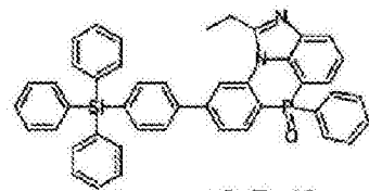
化学式 2-7-48
