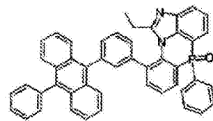
化学式 2-8-18
