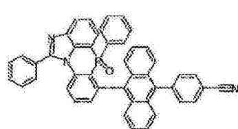
化学式 2-6-12
