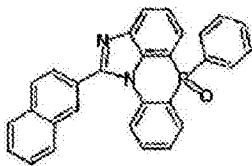
化学式 2-5-37
