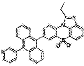
化学式 1-3-10
