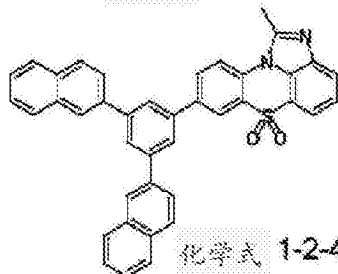
化学式 1-2-40
