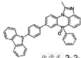
化学式 2-2-42
