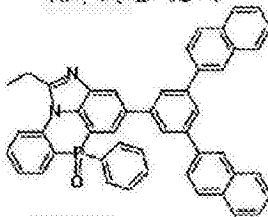
化学式 2-10-7
