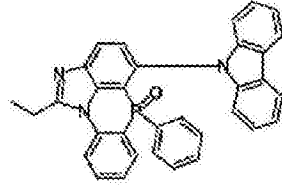
化学式 2-9-14
