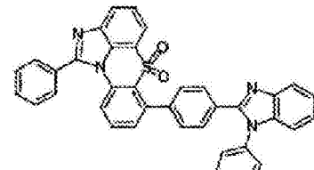
化学式 1-6-45
