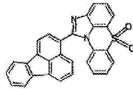
化学式 1-5-30
