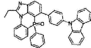
化学式 2-9-6
