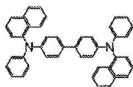
\alpha -NPD
