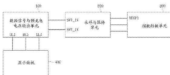
100 ... 数据信号与预充电电压输出单元 200 ... 采样与保持单元 300 ... 模数转换器 400 ... 显示面板
