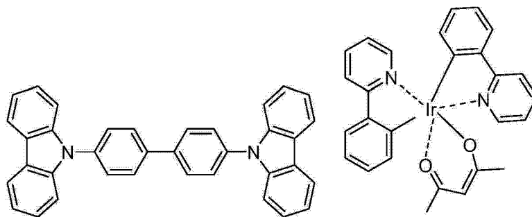
Ir(ppy) 2 acac
