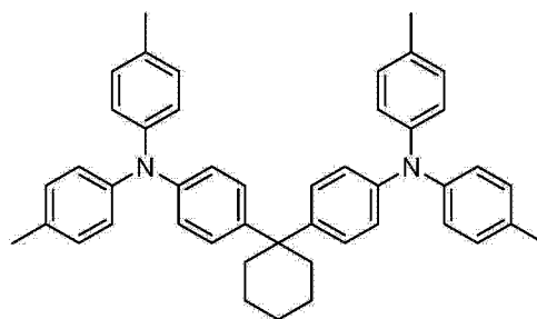
TAPC
